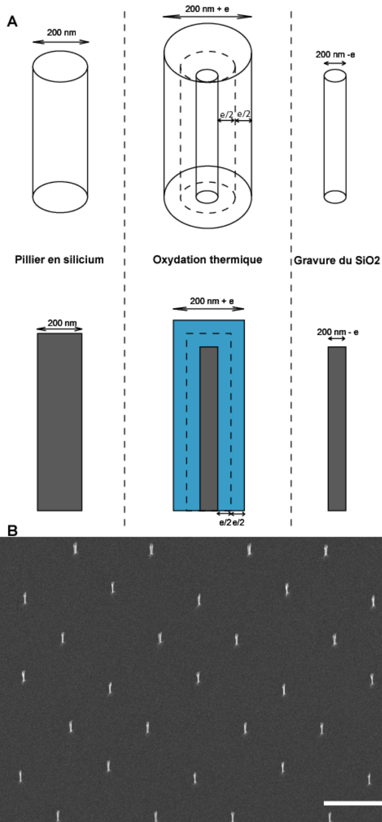
Figure 2.9 : (A) procédé d'amincissement d'un pilier de silicium par oxydation thermique puis gravure HF. (B) réseau de nanoplots de 80\text{ nm} de diamètre obtenus à partir de plots de 140\text{ nm} de diamètre amincis par ce procédé. La barre d'échelle correspond à une longueur de 3\text{ }\mu\text{m} .
