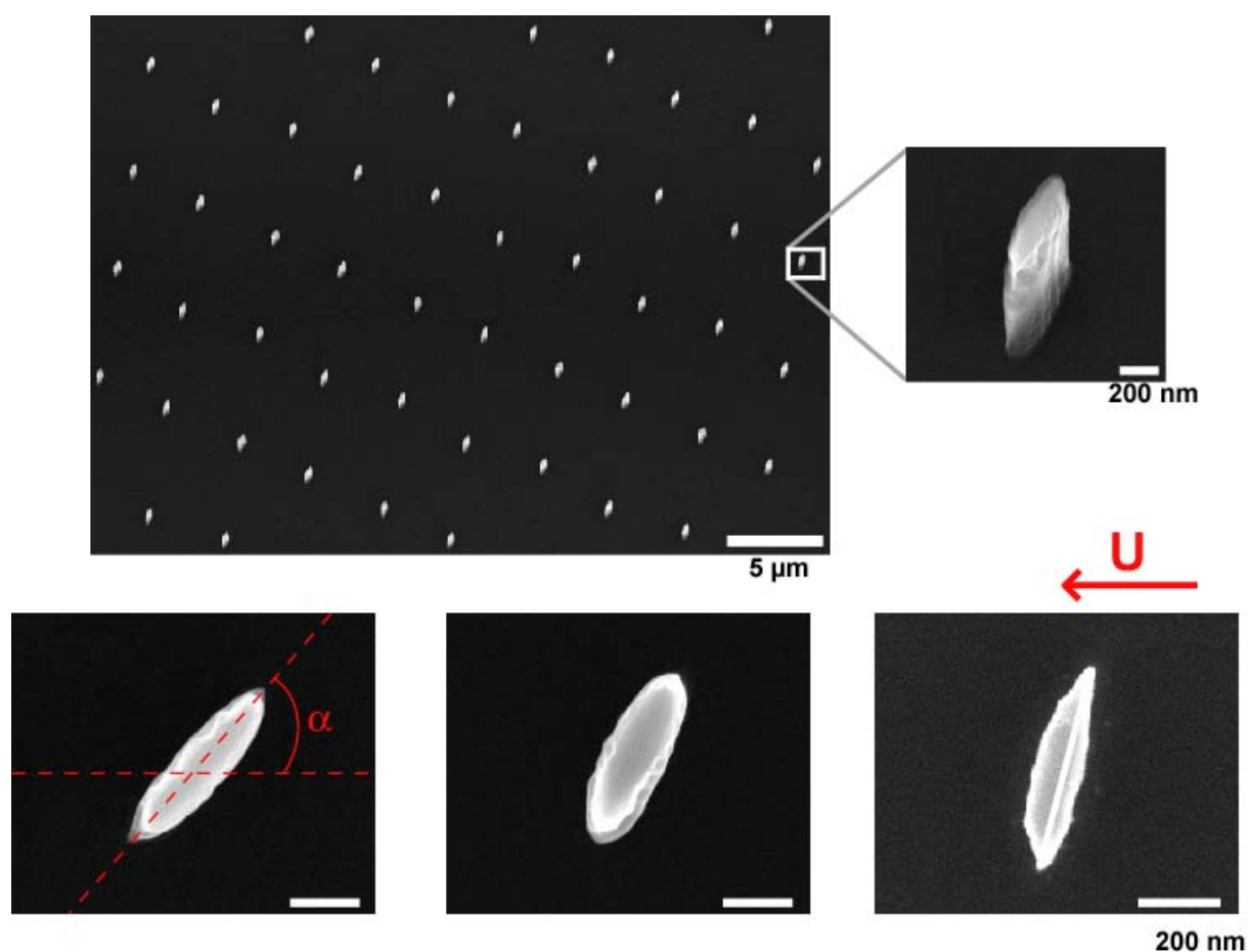
Figure 5.2: images MEB des différentes orientations d'obstacles ellipsoïdaux utilisés dans nos expériences. Dans la configuration 1 ( gauche ), les obstacles sont caractérisés par D=645 nm, d=240 nm et \alpha=47^\circ ; dans la configuration 2 ( milieu ), les obstacles sont caractérisés par D=580 nm, d=200 nm, et \alpha=63^\circ . En fin dans la configuration 3 ( droite ), les obstacles sont caractérisés par D=500 nm, d=130 nm et \alpha=76^\circ . La flèche représente la direction du flux hydrodynamique.
