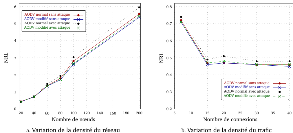
FIGURE 3.14 – Charge de routage normalisée (NRL)
