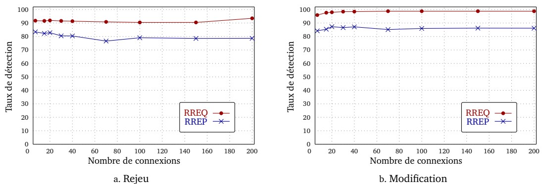
FIGURE 3.6 – Impact de la variation du trafic dans un réseau de 100 nœuds
