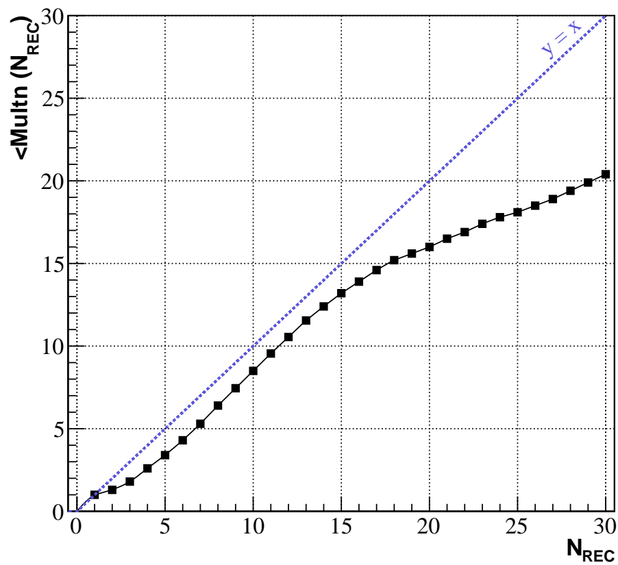
FIGURE 3.50 – Courbe de conversion de N_{NumMax} (N_{REC}) vers \langle Mult(n) \rangle .
