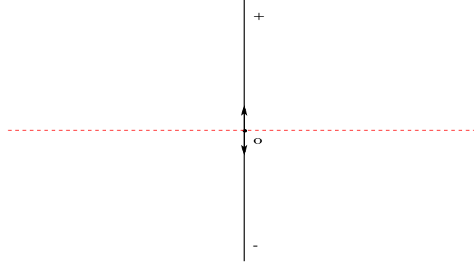
Figure 1.4: Équation du mouvement brownien biaisé.
