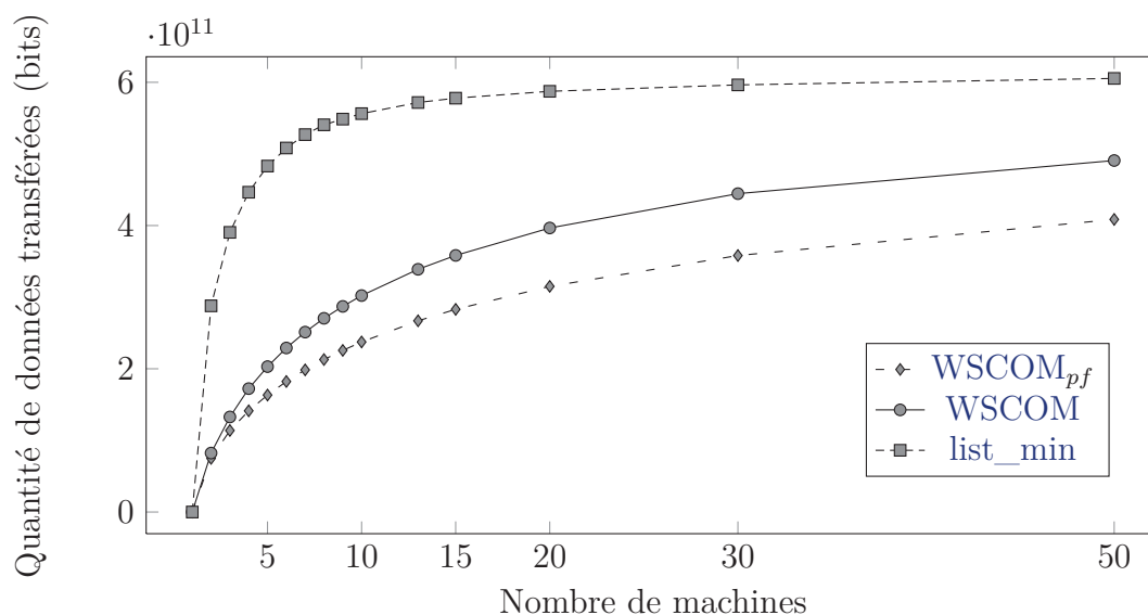
FIGURE 5.17 – Quantité de données transférées par les heuristiques list_min, WSCOM et WSCOM pf en ordonnant des DAG aléatoires sur une plate-forme de type grappe.
