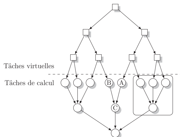
FIGURE 4.3 – Illustration d'une découpe avec un arbre binaire d'un DAG de Makefile.
