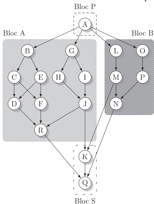
FIGURE 4.6 – Illustration d'une découpe en groupes convexes.
