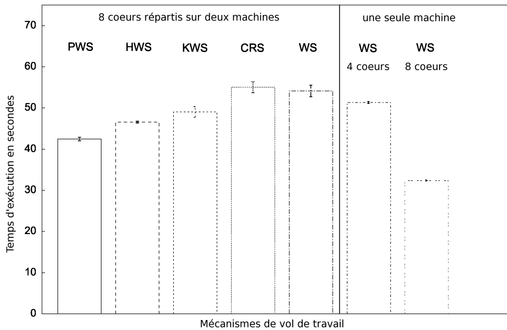
FIGURE 7.8 – Temps d'exécution pour trier un tableau de 4 Giga-octets avec différentes mécanismes de vol de travail en mémoire partagée ou distribuée.
