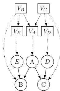
FIGURE 4.13 – Exemple détaillant les choix possibles pour la DHT.
