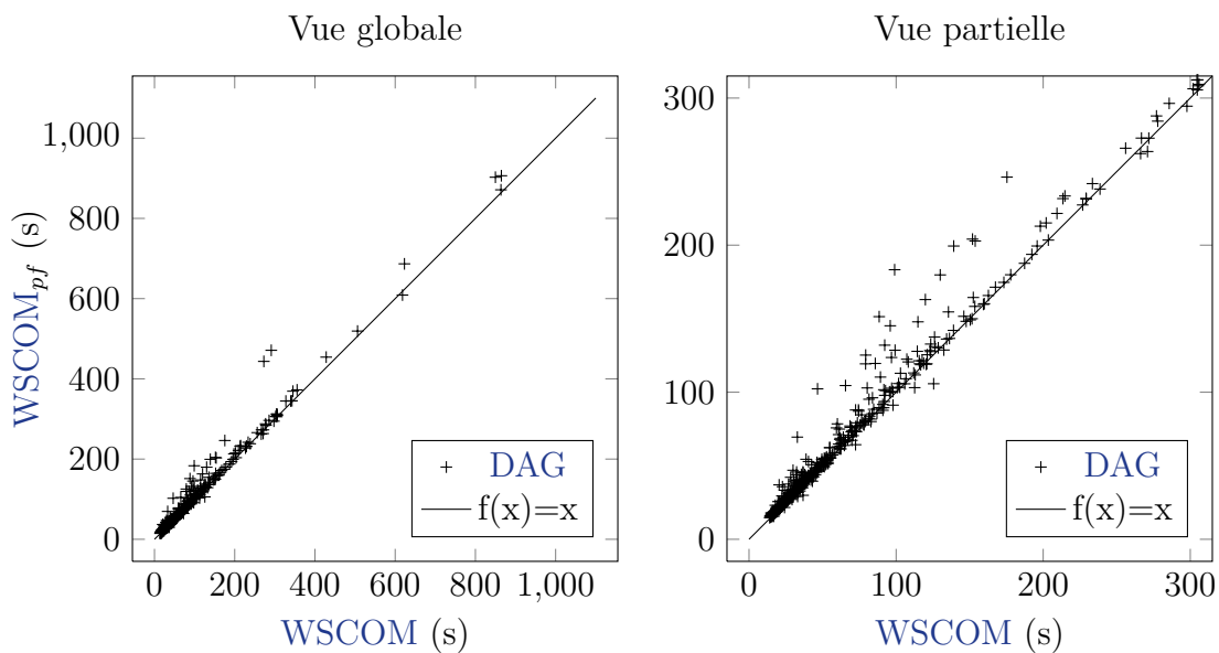
FIGURE 5.19 – Comparaison de WSCOM , WSCOM_{pf} avec des DAG provenant de Makefile sur une grappe.
