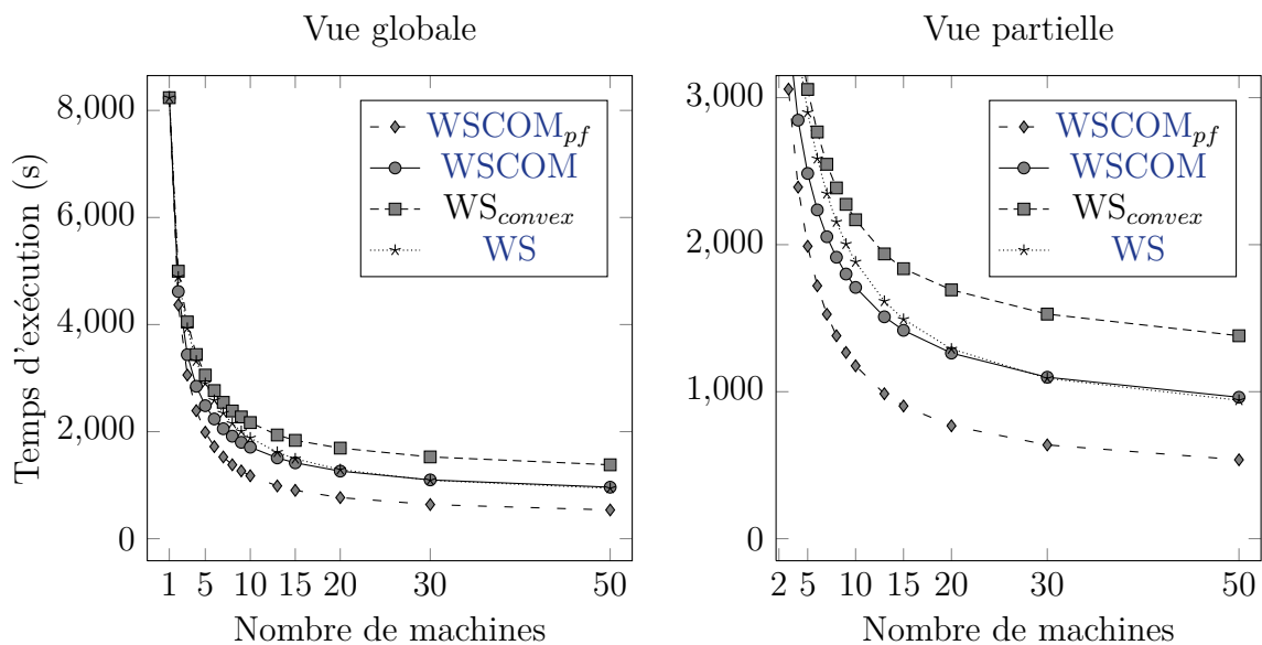
FIGURE 5.11 – Ordonnancement de DAG aléatoires ayant des données volumineuses avec WSCOM, WS_{convex} et WS.
