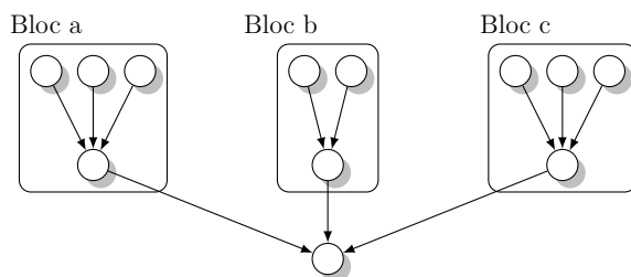
FIGURE 4.2 – Illustration d’un DAG de Makefile classique avec une découpe en blocs.
