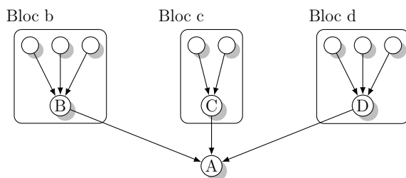
FIGURE 4.8 – Illustration d'un DAG de Makefile classique.
