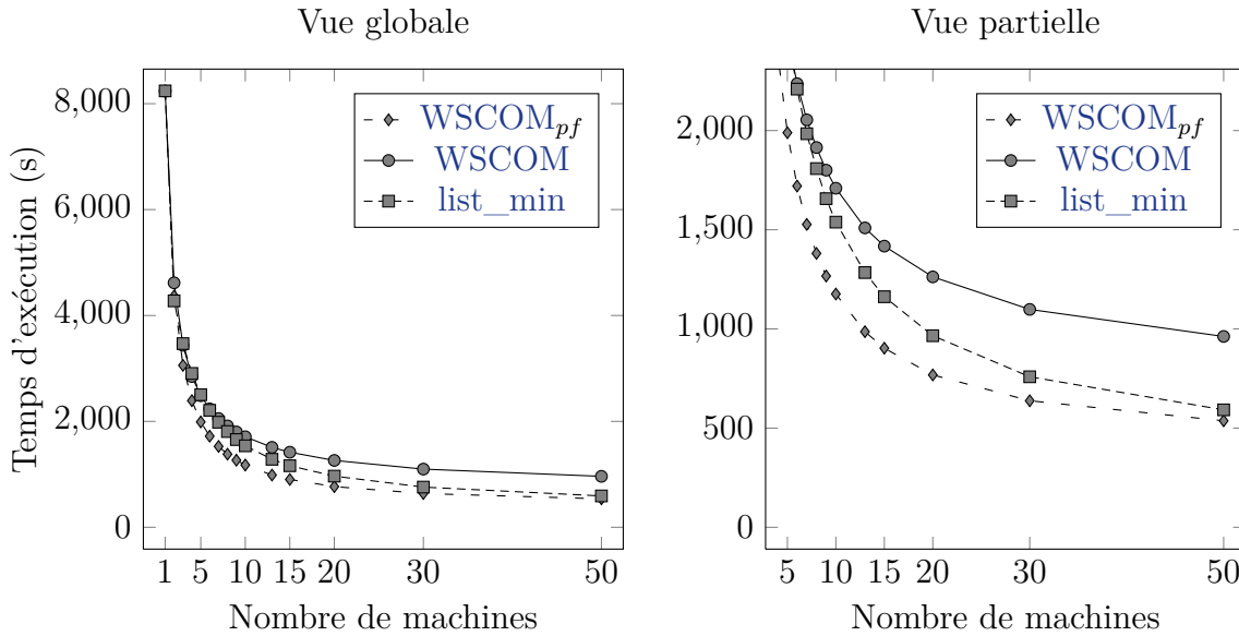
FIGURE 5.16 – Comparaison des heuristiques list_min , wscm et wscm pf sur dag aléatoires ayant des données volumineuses avec une plate-forme de type grappe.
