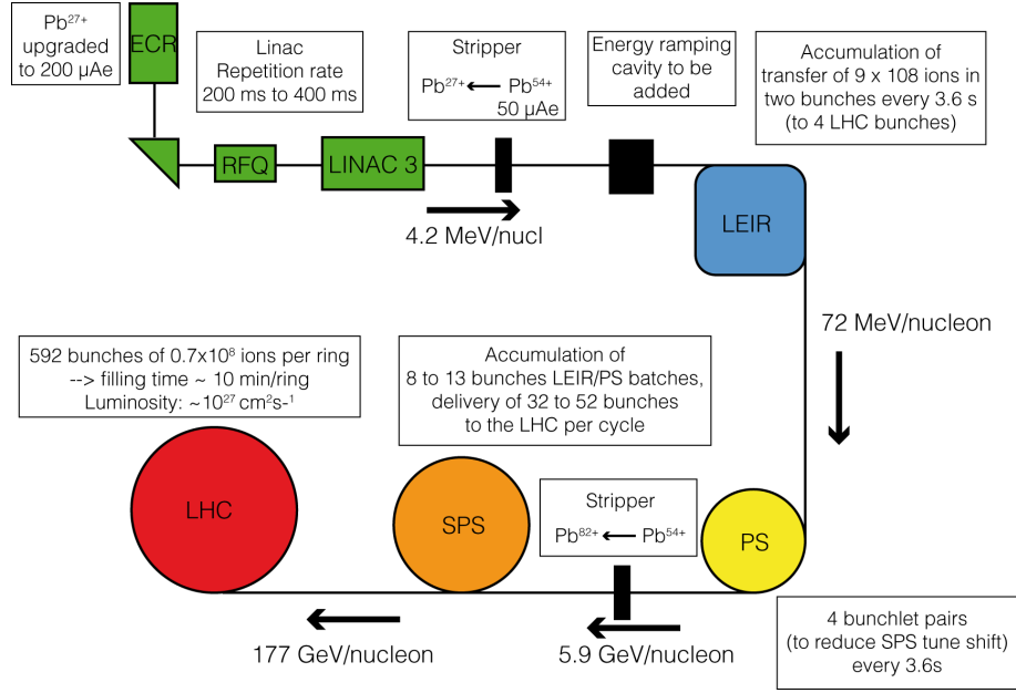
FIGURE 2.2 – Production et accélération des ions Pb
