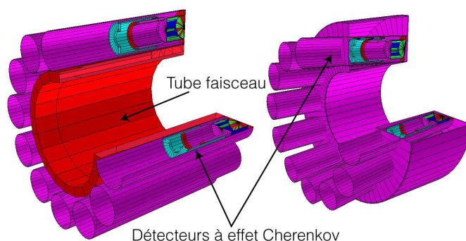
FIGURE 3.16 – Gauche : T0Left , droite : T0Right.
