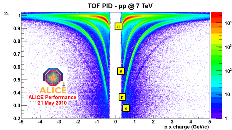
FIGURE 3.11 – Identification de différentes particules par le TOF.
