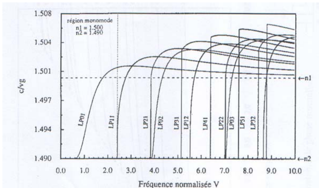
Fig. I.7 la courbe de l'indice effectif en fonction de la fréquence normalisée [31].
