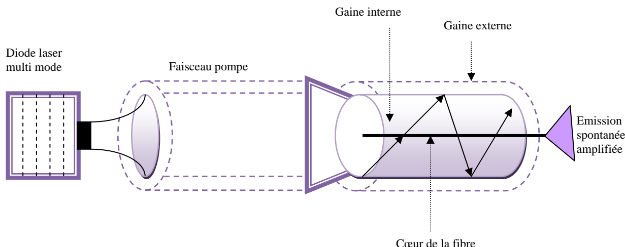
Fig. I.6 Un schéma d'un laser à fibre double gaine dopée aux terres rares
