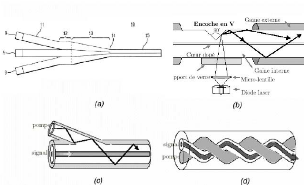
Fig. I.3 Les différentes méthodes de couplage de la lumière dans la gaine interne.
