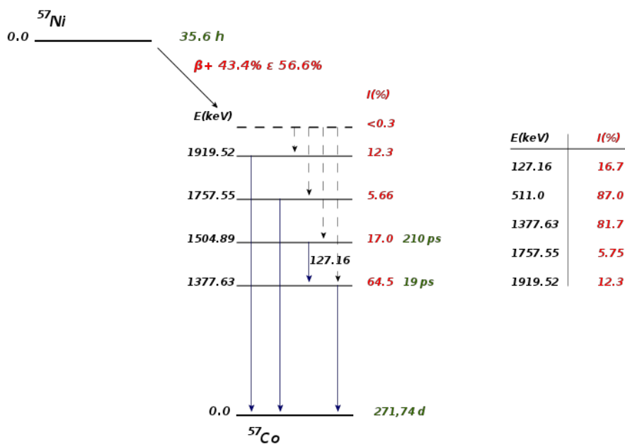
FIGURE 4.14 - Décroissance du ^{57}\text{Ni} et déséxcitation vers le niveau fondamental et les principales raies observables. Les niveaux ayant une probabilité de population négligeable ne sont pas représentés.
