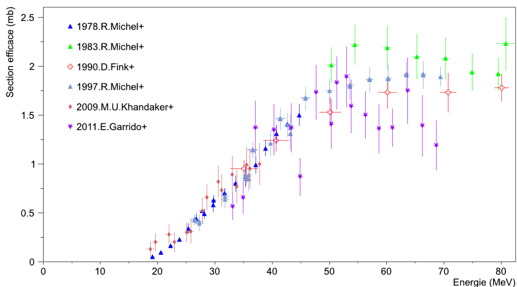
FIGURE 4.25 - Sections efficaces de la réaction {}^{\text{nat}}\text{Ti}(p,X){}^{48}\text{Sc} .
