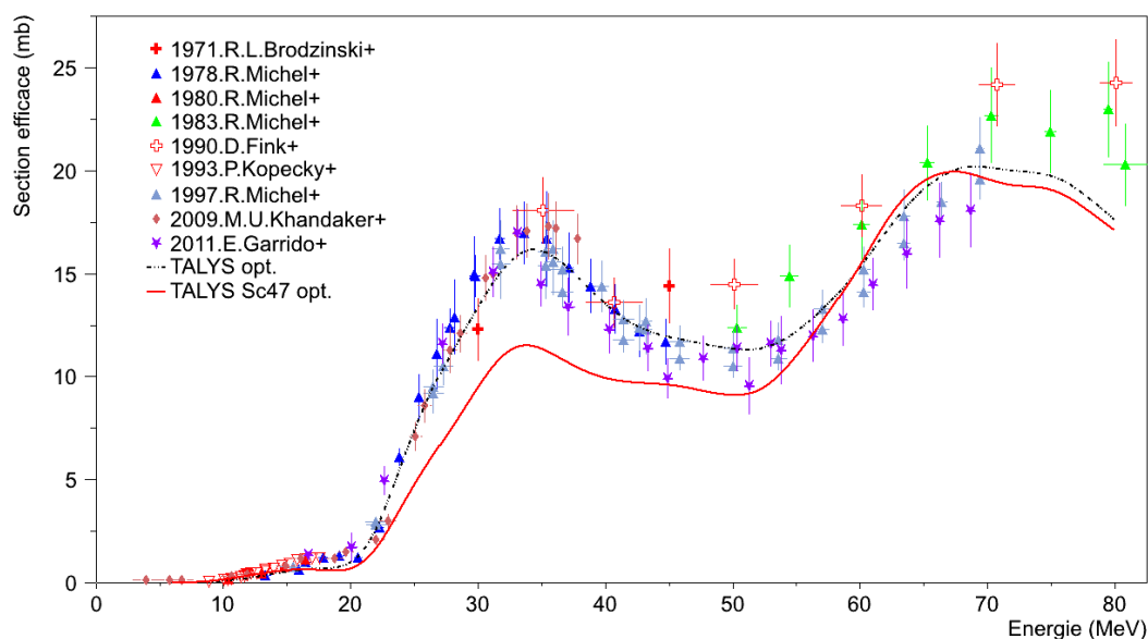
FIGURE 7.10 - Comparaison entre les prédictions théoriques du code TALYS optimisées, pointillés, pour la réaction {}^{\text{nat}}\text{Ti}(p, X) {}^{44\text{m}}\text{Sc} et celles issues du jeu de paramètre optimal de la réaction {}^{\text{nat}}\text{Ti}(p, X) {}^{47}\text{Sc} , trait plein.
