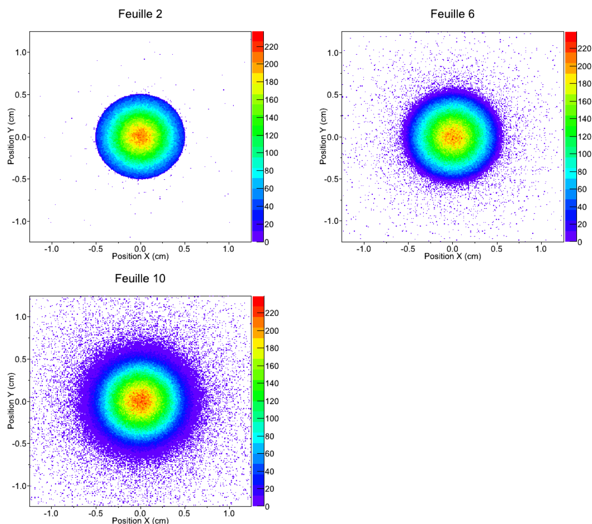
FIGURE 3.5 - Distribution spatiale des particules du faisceau initial sur les feuilles 2, 6 et 10 d'une irradiation à 35 MeV. Les bornes des axes sont conformes aux dimensions des feuilles, 25 mm par 25 mm.
