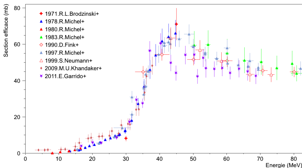
FIGURE 4.24 - Sections efficaces de la réaction {}^{\text{nat}}\text{Ti}(p,X){}^{46}\text{Sc} .
