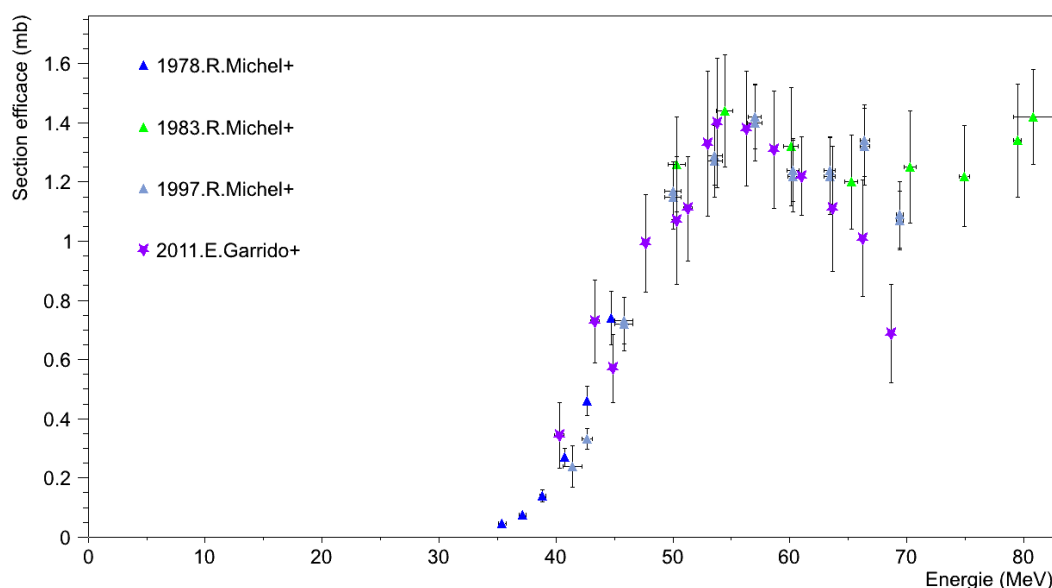
FIGURE 4.20 - Sections efficaces de la réaction {}^{\text{nat}}\text{Ti}(p,X){}^{43}\text{K} .
