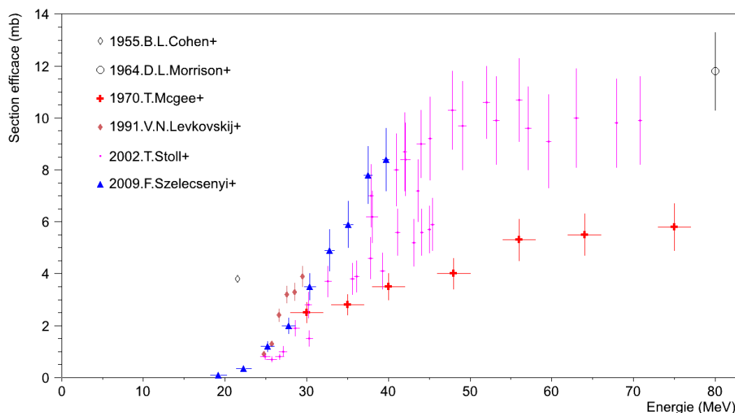
FIGURE 5.2 - Données expérimentales des sections efficaces de la réaction ^{68}\text{Zn}(p, 2p)^{67}\text{Cu} déjà présentes dans la littérature [15].
