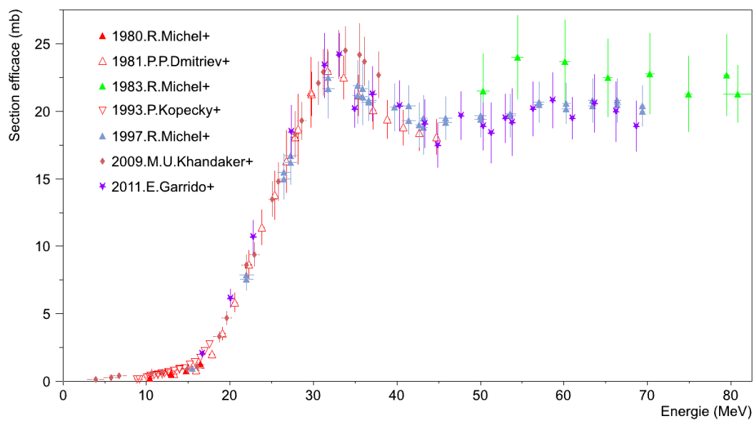
FIGURE 4.17 - Sections efficaces pour la réaction {}^{\text{nat}}\text{Ti}(p, X) {}^{47}\text{Sc} .
