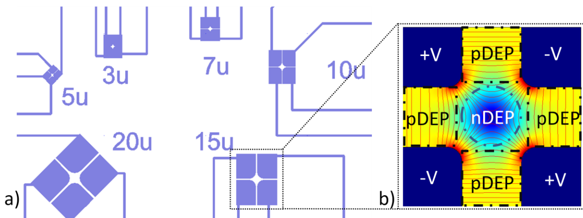
Figure 2-11- a) Dessin de masques de différentes électrodes quadripolaires dont l'espace entre deux électrodes adjacentes est de 20µm, 15µm, 10µm, 7µm, 3µm et 5µm b) Simulation du champ électrique
