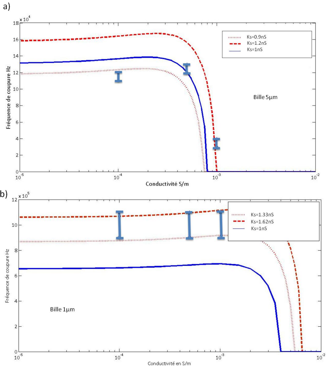
Figure 2-14- Encadrement des valeurs de K_S pour une sphère de a) 5 \mu m de diamètre et de b) 1 \mu m de diamètre à partir de données expérimentales en utilisant un modèle sphérique.
