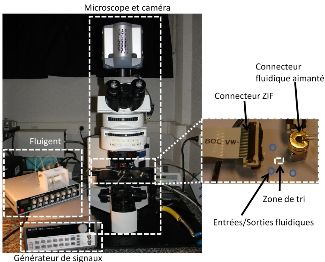
Figure 2-10- Banc de mesure et connectiques fluïdiques ou électriques
