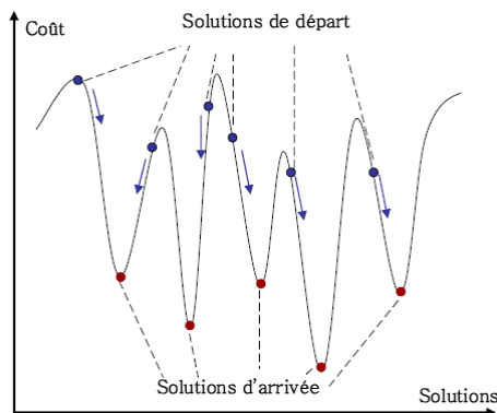
Figure 9 : Illustration de la méthode de « descente multi-start »
