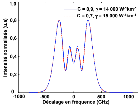
FIGURE 4.1 – Spectres simulés en sortie d'une fibre non-linéaire de 68 \text{ cm} de long ( \alpha = 15 \text{ dB.m}^{-1} ; D = -2 \text{ 000 ps.nm}^{-1}.\text{km}^{-1} ) avec C = 0,9 , \gamma = 14 \text{ 000 W}^{-1}.\text{km}^{-1} (ligne continue) et C = 0,7 , \gamma = 15 \text{ 000 W}^{-1}.\text{km}^{-1} (ligne pointillée) lorsque la puissance crête de l'impulsion d'entrée est de 4,9 \text{ W} .
