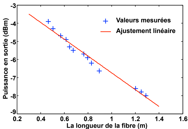
FIGURE 4.25 – Puissance en sortie de la fibre AsSe 2010 en fonction de sa longueur.
