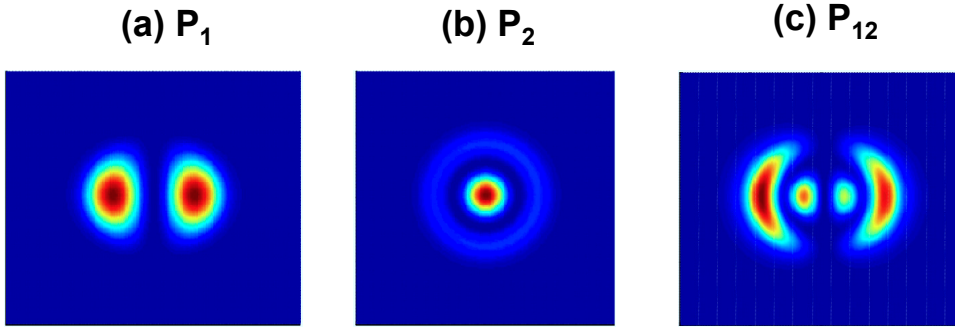
FIGURE 3.6 – Profil transverse des HOMs extraites de trois pics dans la figure 3.5a. (a) Mode LP 11 correspondant au pic P 1 , (b) mode LP 02 correspondant au pic P 2 et (c) mode parasite correspondant au pic P 12 .
