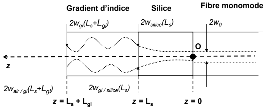
FIGURE 2.8 – Paramètres du faisceau dans la gradissimo.
