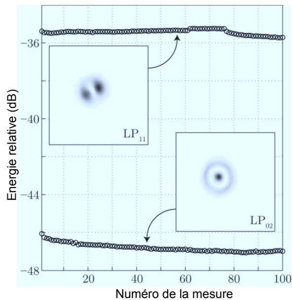
FIGURE 3.12 – Répétabilité de la technique pour la fibre multimode à saut d'indice, d'après [13].
