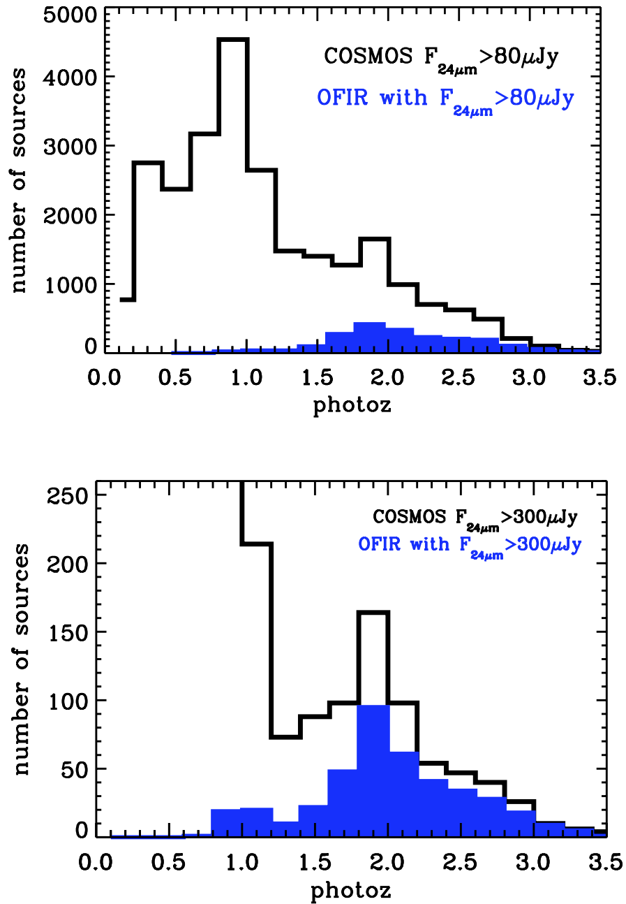
FIGURE 6.2 – Haut Distribution en redshift des galaxies optiquement faibles mais brillantes en IR avec F_{24\mu m} > 0.08\text{ mJy} (histogramme plein bleu) comparé à la population MIPS totale dans COSMOS (trait noir). Bas Distribution en redshift obtenues pour les sources satisfaisant la condition F_{24\mu m} > 0.3\text{ mJy} (même définition des couleurs que précédemment) La contribution relative des galaxies optiquement faibles mais brillantes en IR à 1.5 < z < 3 augmentent avec la luminosité en IR-moyen ( \sim 30\% pour une coupure en flux à 0.08\text{ mJy} et \sim 60\% pour une coupure en flux à 0.3\text{ mJy} ).
