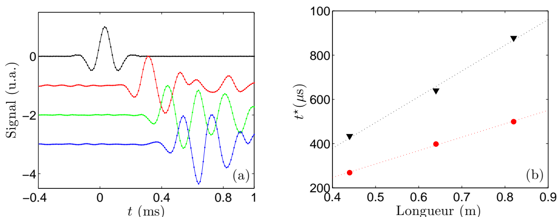
FIG. IV.11 – (a) : Signaux enregistrés par le capteur piézoélectrique en bout de chaîne pour trois longueurs de chaîne différentes soumises à F_0 = 186 \text{ N} . La courbe du haut correspond au signal envoyé à l'émetteur. Les courbes ont été décalées verticalement pour une meilleure lisibilité. On observe le décalage temporel entre les trois courbes qui donne le temps de propagation. (b) : Mesure du temps de vol t^* du point à mi-hauteur en fonction de la longueur de chaîne pour une force statique F_0 = 186 \text{ N} (●) et F_0 = 43 \text{ N} (▼). On trouve respectivement c_s = 1632 \text{ m/s} et c_s = 945 \text{ m/s} .
