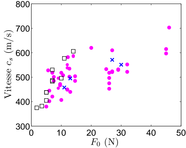
FIG. VI.11 – Evolution de la vitesse c_s des ondes acoustiques pour trois empilements différents tous avec un motif hexagonal. Les mesures faites pour différentes chaînes de forces mais appartenant à un même empilement ont été regroupées sous un même symbole. Le symbole ( \bullet ) correspond aux mesures faites sur les cinq chaînes de forces de la Fig. VI.10. Le symbole ( \times ) représentent les mesures faites à 10^5 images/s.
