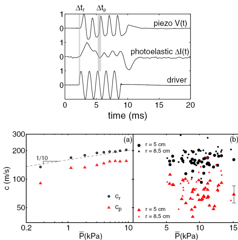
FIG. VI.17 – Tiré de [113]. Mesure de la vitesse des ondes acoustiques dans un milieu 1D (a) et 2D (b). Les intervalles \Delta t_r et \Delta t_p permettent d'estimer les deux vitesses c_r (○) et c_p (△).
