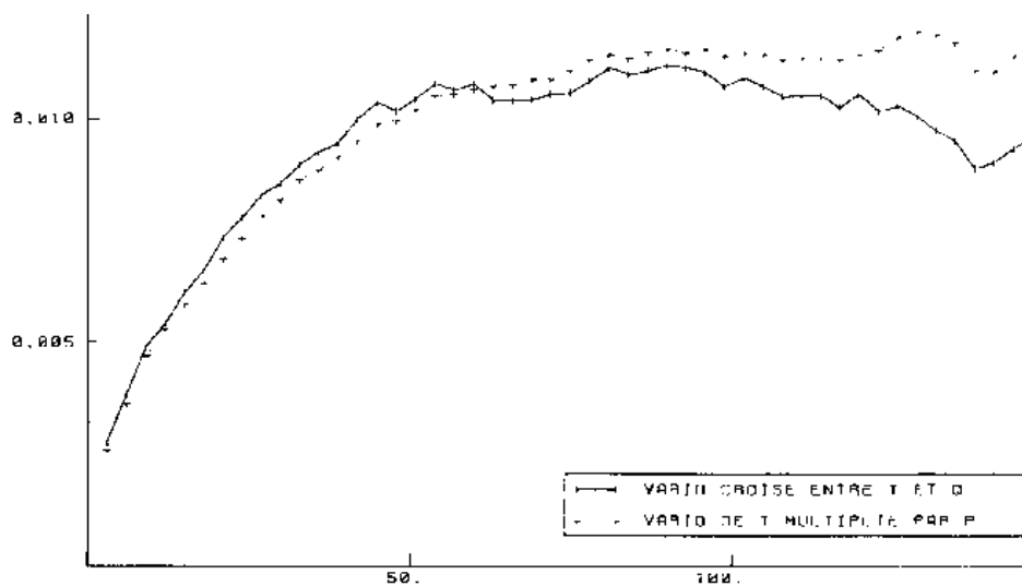
Figures 9. Variographie de variables utiles minéral et métal. En haut, variogrammes simples du minéral, du métal, et du résidu : on notera le contraste entre la structure du minéral (assez continue), et celle du métal (beaucoup plus variable), due au résidu. En bas : le variogramme croisé entre minéral et métal est pratiquement proportionnel au variogramme simple du minéral. (Extrait de Bordessoule et al., 1988.)
