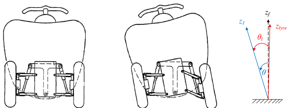
Figure 4.11 : Mouvement de la lyre avant lors de l'inclinaison
