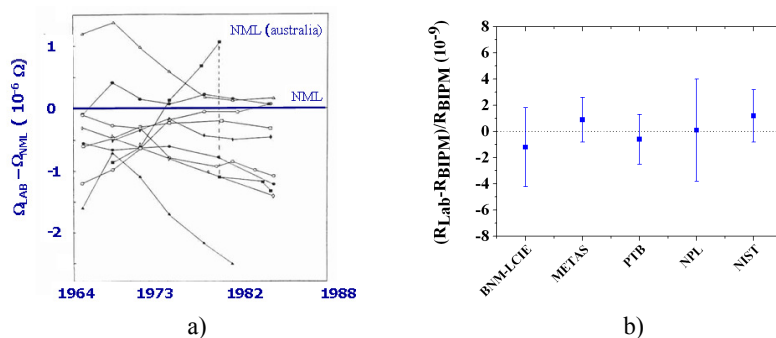
FIGURE 1.3 – a) Comparaison de l'ohm entre différents NMIs ( \Omega_{LAB} ) et le NMI d'Australie ( \Omega_{NMI} ); b) Comparaison bilatérale entre le BIPM et différents NMIs.
