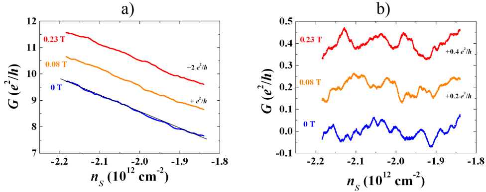
FIGURE 9.23 – En a), conductances brutées exprimées en e^2/h mesurées à T = 350 \text{ mK} avec I = 30 \text{ nA} pour différentes inductions magnétiques (les deux courbes supérieures ont volontairement été décalées de +e^2/h et +2e^2/h pour améliorer la lisibilité). En b), conductances obtenues après soustraction d'un terme linéaire en n_s (les deux courbes supérieures ont volontairement été décalées de +0.2e^2/h et +0.4e^2/h pour améliorer la lisibilité).
