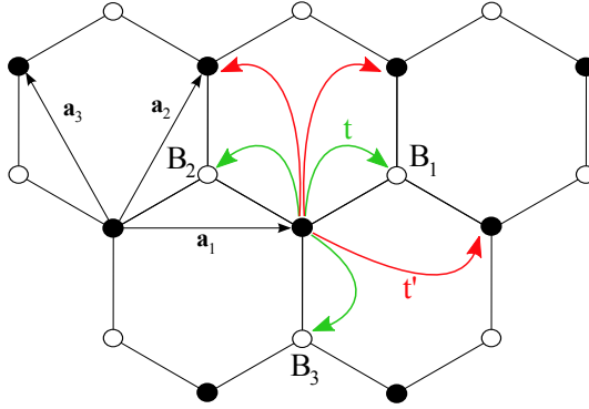
FIGURE 5.2 – Représentation schématisée des sauts aux plus proches voisins ( t , flèches vertes) et aux seconds plus proches voisins ( t' , flèches rouges) dans une monocouche de graphène.
