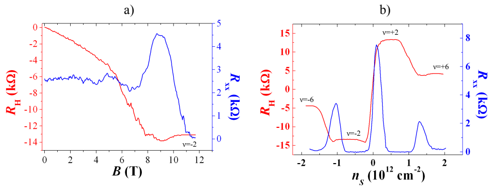
FIGURE 9.27 – Effet Hall quantique dans la monocouche ML002 observé : a) en faisant varier l'induction magnétique à densité constante n_S \approx -8.2 \times 10^{11} \text{ cm}^{-2} et b) en faisant varier la densité à induction magnétique constante B = 11.7 \text{ T} . Les deux mesures ont été faites à T = 1.3 \text{ K} et I = 200 \text{ nA} . En trait rouge on a fait figurer la résistance de Hall et en trait bleu la résistance longitudinale.
