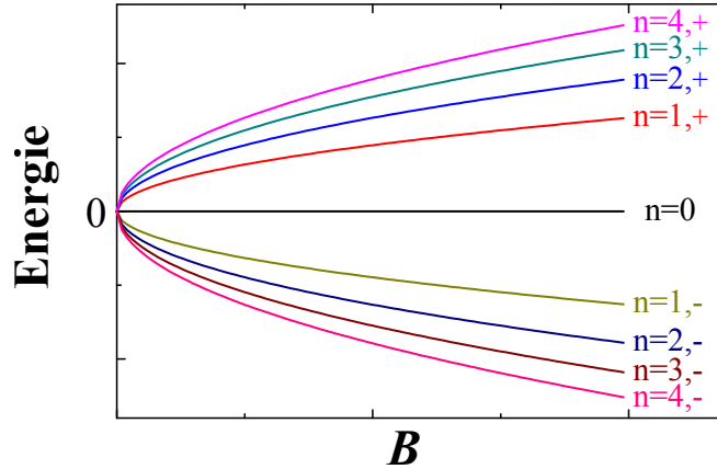
FIGURE 6.1 – Niveaux de Landau d'énergies positive et négative dans une monocouche en fonction du champ magnétique
