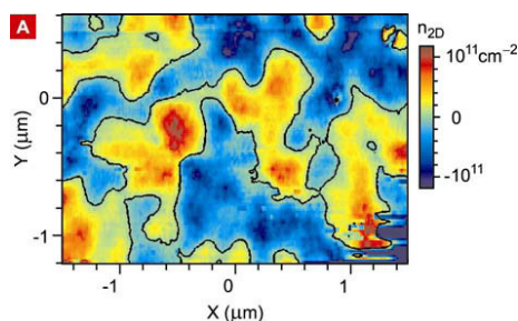
FIGURE 9.2 – Observation des flaques d'électrons et de trous; la figure, tirée de [70], représente la variation spatiale de densité de porteurs de charge mesurée à T = 0.3 \text{ K} (en bleu les flaques de charges positives et en rouge celles de charges négatives).
