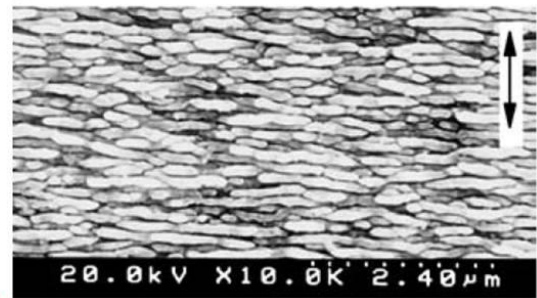
Figure I-24 : (1) Image MEB d'un dommage réalisé dans un miroir Ta_2O_5/SiO_2 . [11] (2) Image SEM de ripples obtenus sur une couche de TiN, la flèche permet de visualiser l'orientation de la polarisation. [146].
