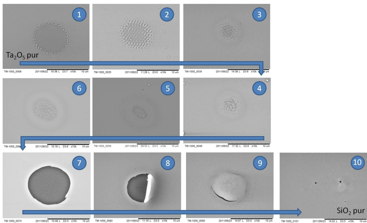
Figure V-12 : Images MEB de dommages obtenus pour des fluences proches du seuil d'endommagement, échantillons de mélanges \text{Ta}_2\text{O}_5/\text{SiO}_2 .
