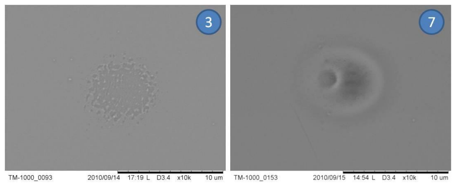
Figure V-10 : Images MEB de dommages sur mélanges \text{HfO}_2/\text{SiO}_2 pour une fluence proche du seuil d'endommagement. Les échantillons non représentés ici se comportent comme l'échantillon 3.
