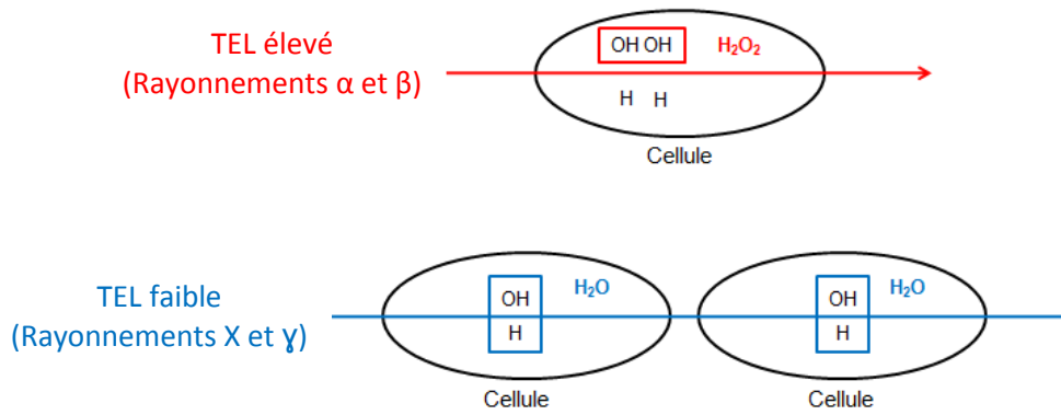
Figure 5 : Ionisation et transfert linéaire d'énergie (TEL)
