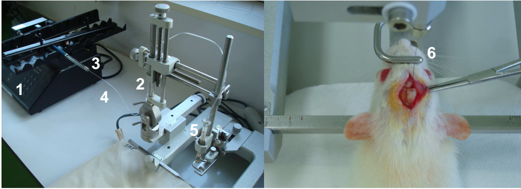
Figure 2 : Systèmes d'injection par SI et par CED. L'ensemble du dispositif comprend : une pompe Harvard PHD 2,000 (1), le cadre de stéréotaxie petit animal, la seringue Hamilton 100µL 22 gauges contenant les NCLs (3), la tubulure externe en PE/PVC (4), la seringue Hamilton 10 µL (5) et l'aiguille de 32G implantée dans le striatum droit du rat (6).
