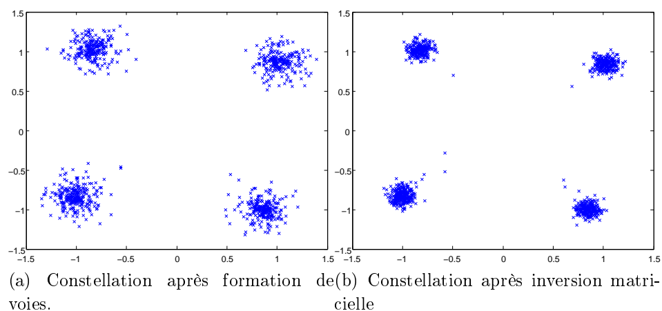
FIGURE 4.23 – Comparaison des constellations après formation de voies et après inversion matricielle sur 8 capteurs. SNR = 23 dB.
