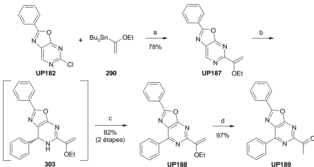
Schéma 88. Conditions et réactifs : (a) \text{PdCl}_2(\text{PPh}_3)_2 , DMF, 75°C, 12h. (b) PhLi, THF, -78 °C, 30 min. puis 3h à 0 °C. (c) \text{MnO}_2 , \text{CH}_2\text{Cl}_2 , reflux, 2h. (d) 1M HCl, \text{H}_2\text{O} , t.a., 2h.
