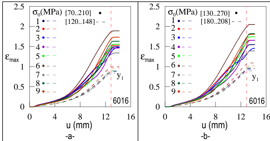
Figure 62. Evolution de \varepsilon_{max} pour 9 répartitions spatiales différentes de \sigma_0 en fonction du déplacement de l'indenteur, (a) pour une distribution équiprobable et aléatoire de \sigma_0 comprise entre [70..210MPa] et [120..148MPa], (b) pour une distribution équiprobable et aléatoire de \sigma_0 comprise entre [130..270MPa] et [180..208MPa].
