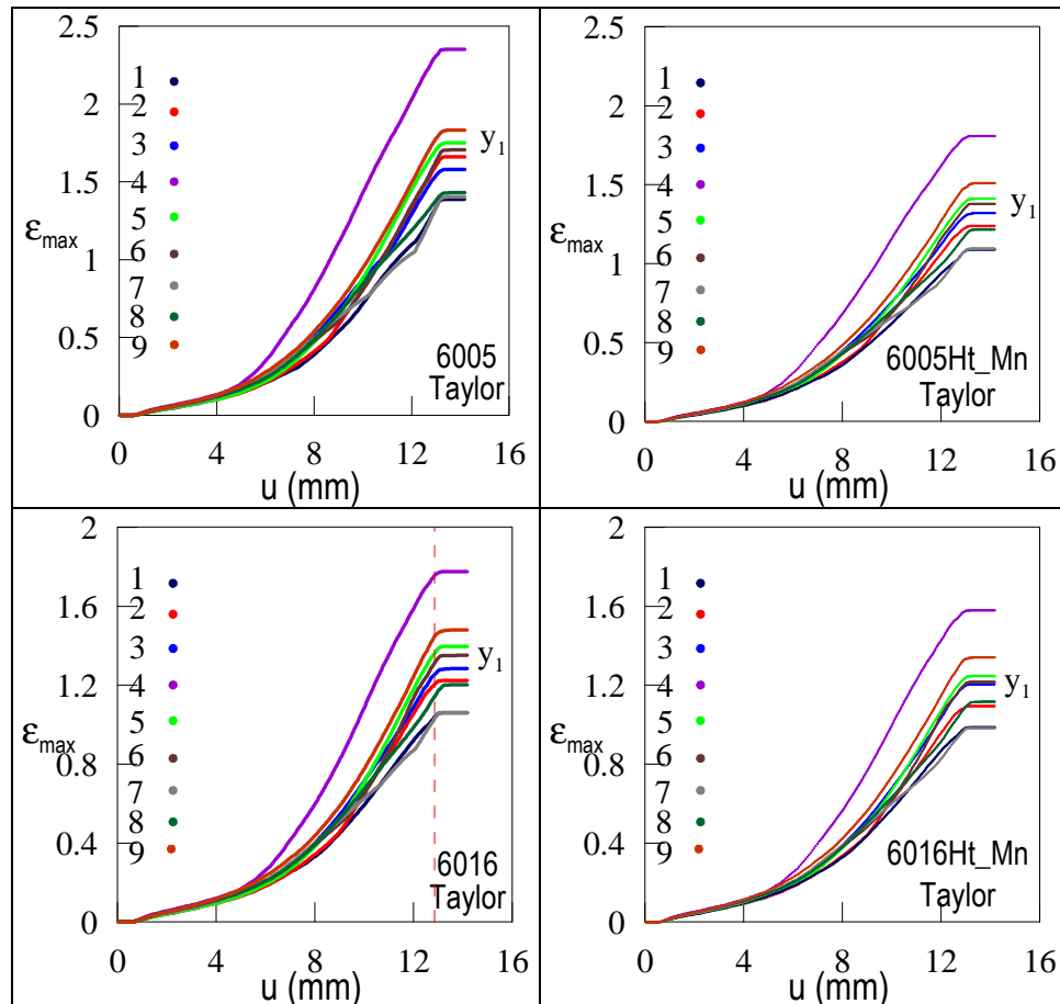
Figure 145. Evolution de \epsilon_{max} pour 9 répartitions spatiales de \sigma_0 en fonction du déplacement de l'indenteur durant un essai de pliage d'une tôle hétérogène avec une distribution de \sigma_0 et une loi de comportement basée respectivement sur la distribution du facteur de Taylor et la loi de comportement de chaque alliage.
