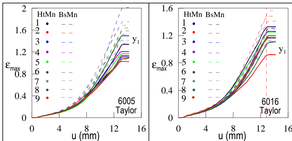
Figure 70. Evolution de \epsilon_{max} en fonction du déplacement de l'indenteur durant la simulation d'un essai de pliage d'une tôle hétérogène avec une distribution de \sigma_0 et une loi de comportement basée respectivement sur la distribution du facteur de Taylor et la loi de comportement de chaque alliage. Pour chaque graphique, les numéros correspondent à des répartitions spatiales de \sigma_0 différentes. De plus, les répartitions spatiales entre alliages sont également différentes.
