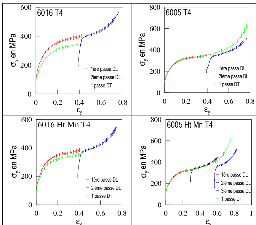
Figure 99. Courbes expérimentales contrainte \sigma_y /déformation \epsilon_y durant un essai de compression plane avec les incertitudes de mesure sur la contrainte, Comparaison entre des essais dans la direction DL et DT.
