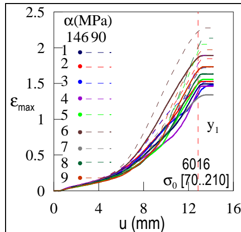
Figure 64. Evolution de \epsilon_{max} pour 9 répartitions spatiales différentes de \sigma_0 en fonction du déplacement de l'indenteur pendant la simulation de l'essai de pliage avec un \sigma_0 distribué de manière aléatoire et équiprobable entre [70..210MPa] et un coefficient \alpha=90 ou 146MPa.
