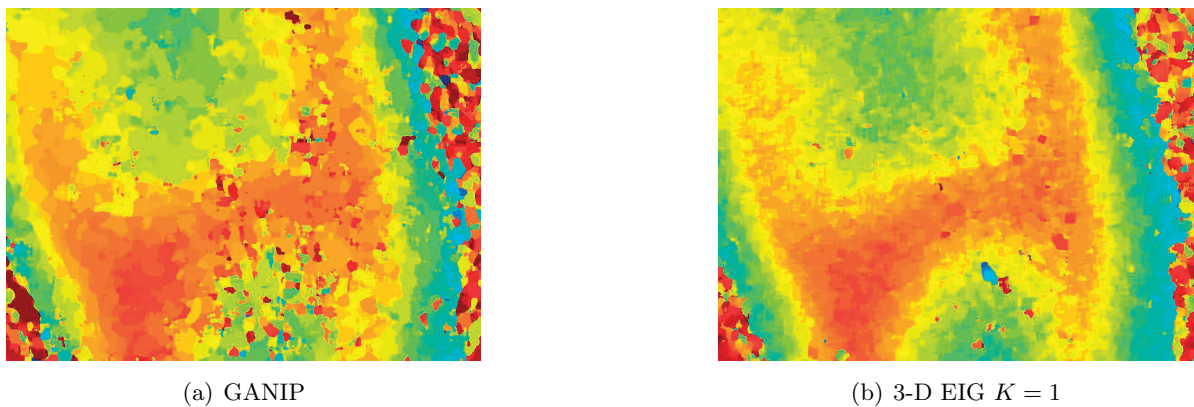
Fig. 10.5 – Cartes des profondeurs reconstruites ( r = 10 pixels) et non interpolées pour la séquence d’images II. Échelle des couleurs en z : 0 ●● 29.25 ●● 58.5 ●● 87.75 ●● 117 ●● 146.25 ●● 175.5 \mu\text{m} . La carte des profondeurs obtenue avec la méthode GANIP ( M=270 pour m_{\max}=255 ) est dégradée par de nombreux artefacts excessivement rougeâtres traduisant des régions de la séquence d’images où la mosaïque apparaît mal fermée à la netteté. Le lecteur pourra se référer à la Fig. 9.6 pour plus de comparaisons.
