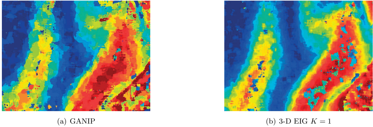
Fig. 10.4 – Cartes des profondeurs reconstruites ( r = 10 pixels) et non interpolées pour la séquence d’images I. Échelle des couleurs en z : 0 ●●● 26.1 ●●● 52.2 ●●● 78.3 ●●● 104.4 ●●● 130.5 \mu\text{m} . La carte des profondeurs obtenue avec la méthode GANIP ( M=270 pour m_{\max}=255 ) comporte moins de trous abrupts causés par des inversions de contraste que la méthode 3-D EIG K = 1 pourtant très robuste. Le lecteur pourra se référer à la Fig. 9.7 pour plus de comparaisons.
