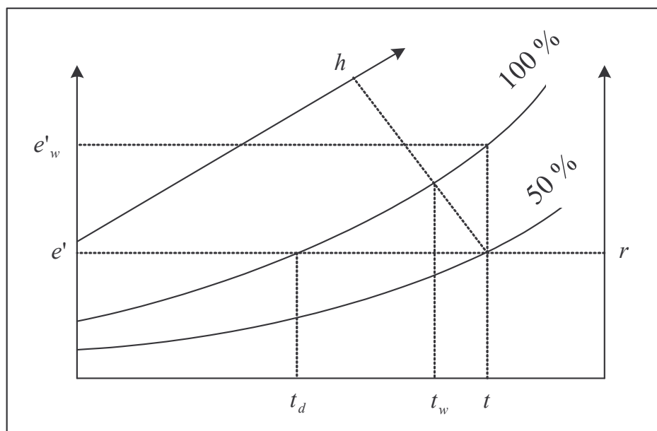
Figure 2. Utilisation du diagramme psychrométrique.
