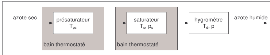
Figure 20. Schéma de principe du générateur d'air humide actuel du LNE.
