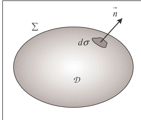
Figure 29. Domaine d'intégration.
