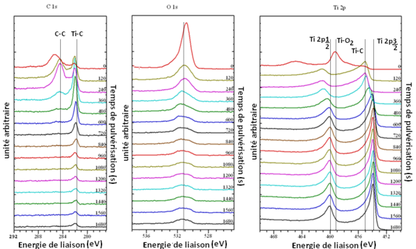
Figure IV. 20 : Spectres XPS C 1s, O 1s et Ti 2p du Ti-6Al-4V implantés avec des ions carbones et oxygènes à une fluence de 40 U.A.
