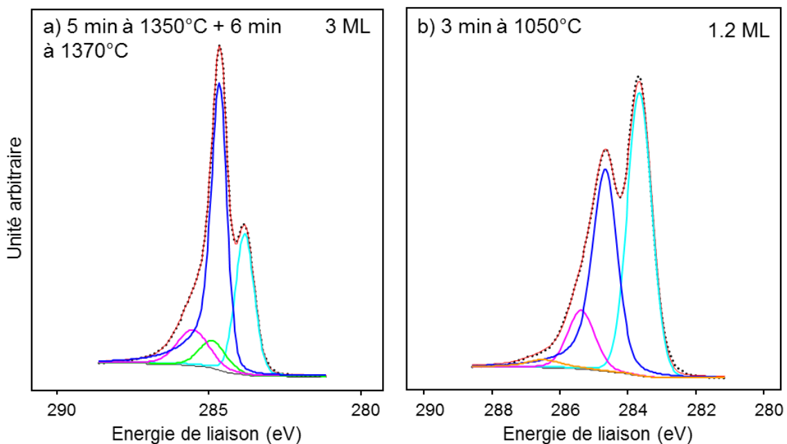
Figure 3. 10. Spectres C1s sur face Si ( h\nu = 1487 eV). Après graphitisation (a), 4 composantes sont nécessaires pour décomposer le spectre expérimental : une composante liée au substrat (turquoise), une seconde pour le graphène (bleu marine) et deux autres pour la reconstruction (6\sqrt{3} \times 6\sqrt{3})R30^\circ (rose et verte). Quant à la croissance (b), l'interface n'étant pas clairement identifiée, une seule composante la modélise (rose), en plus des composantes de substrat (turquoise), de graphène (bleu marine) et d'oxydation (orange).
