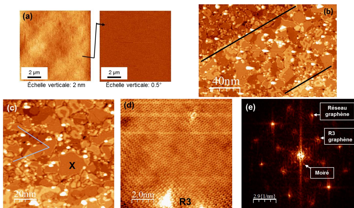
Figure 4. 9. Images par microscopie à champ proche d'une croissance de 20 min à 1050°C face C:
