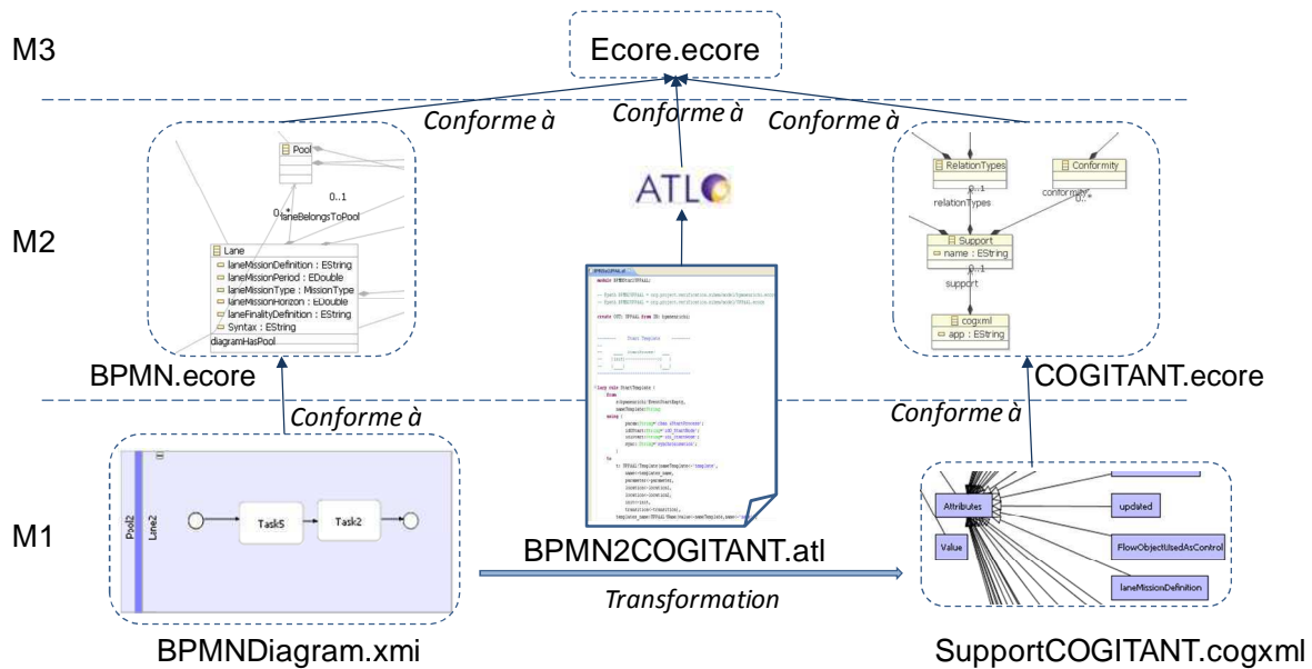
Figure 31. Transformation de BPMN enrichi vers des graphes conceptuels
