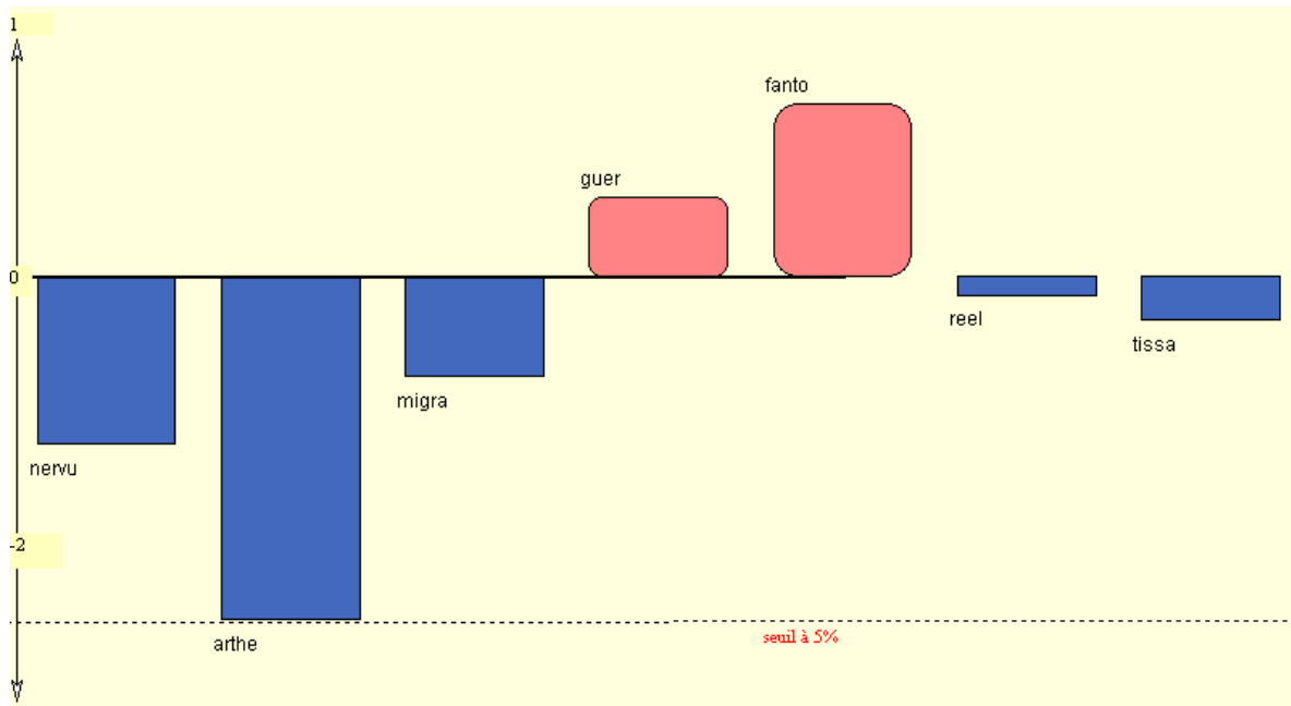
Fig. 28 : Accroissement inverse calculés sur N (occurrences)
