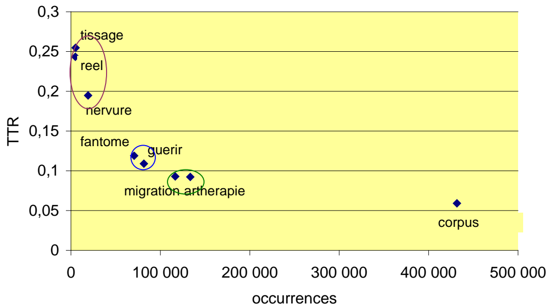
Fig. 24 : le TTR en fonction du nombre d'occurrences
