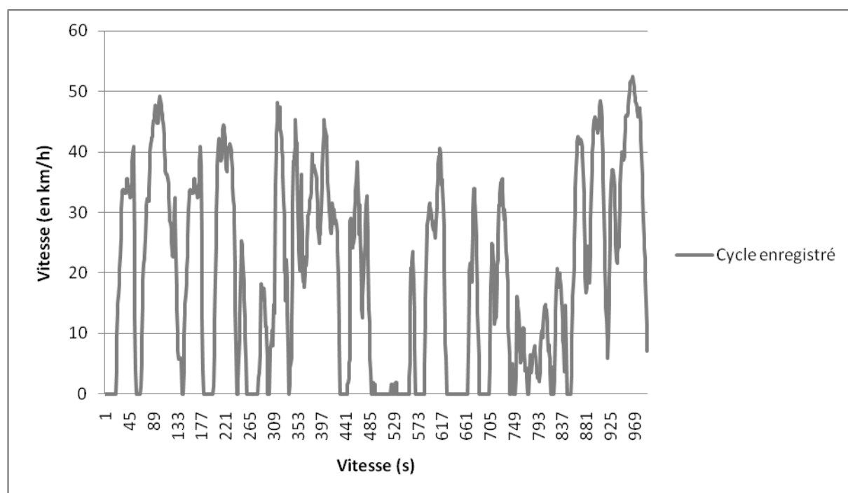
Figure 55 : Diagramme vitesse / temps du cycle enregistré
