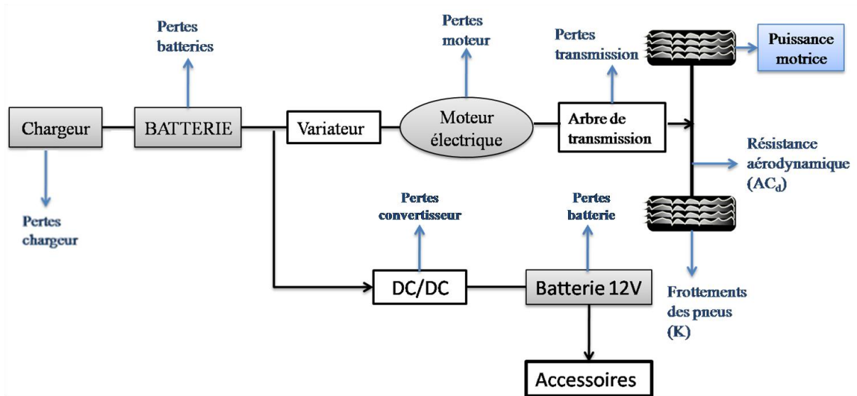
Figure 20 : Phase de traction, la batterie fournit la puissance motrice et les pertes
