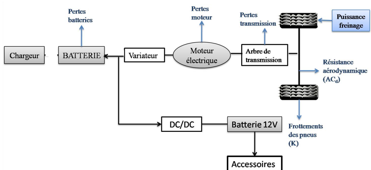
Figure 21 : Phase de freinage, la batterie enmagasine une partie de l'énergie restituée
