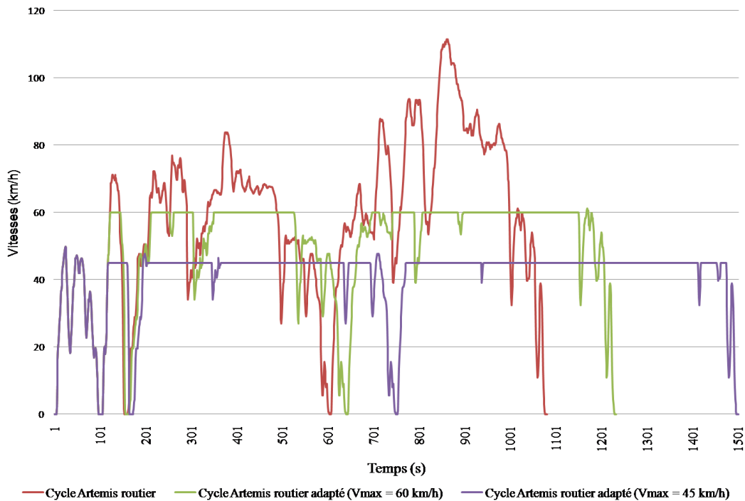
Figure 17 : Adaptation du cycle Artémis routier aux performances des véhicules étudiés
