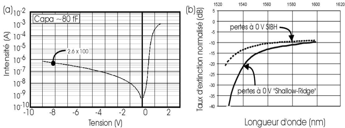
Fig. IV-21 : Mesure de courants de fuite et de capacité (a) pour un modulateur « Shallow-Ridge » de 2.6 x 100 μm². Comparaison des pertes de propagation à 0 V entre un modulateur SIBH de 1.8 x 100 μm² et un modulateur « Shallow-Ridge » de 2.6 x 50 μm² (b) tous deux à base d'AlGaInAs provenant de la même épitaxie.
