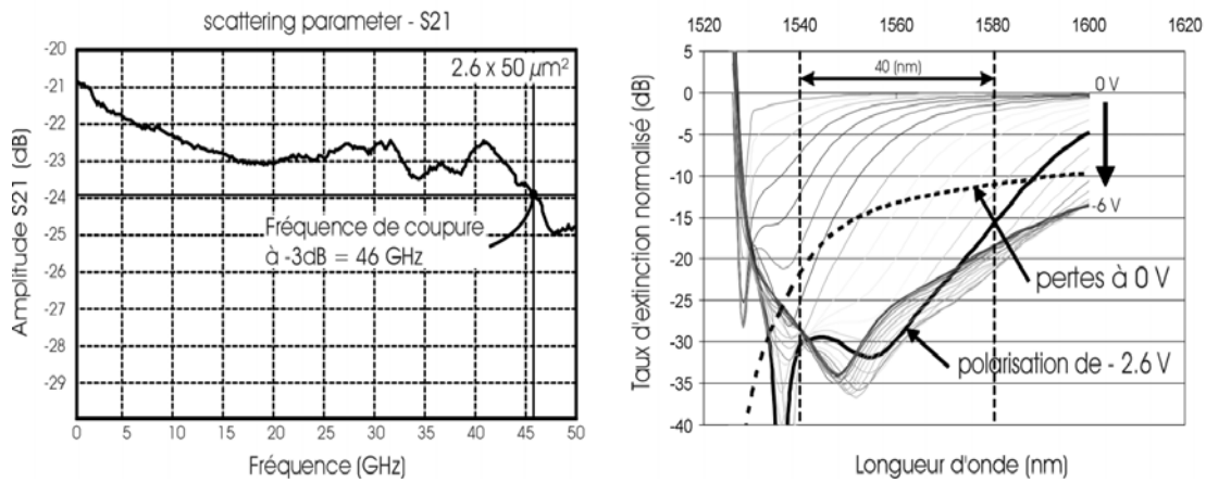
Fig. IV-20 : Mesure de bande passante et de taux d'extinction pour un modulateur « Shallow-Ridge » à base d'AlGaInAs de 2.6 x 50 μm².
