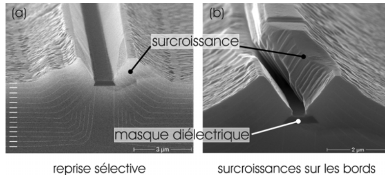
Fig. I-12 : Images prises au Microscope Electronique à Balayage de rubans d'InP de 1 µm de large et 3 µm de hauteur recouvert d'un masque de \text{Si}_3\text{N}_4 de 250 nm d'épaisseur après reprise MOVPE. Les deux images représentent le même ruban à différents endroits sur le substrat repris.
