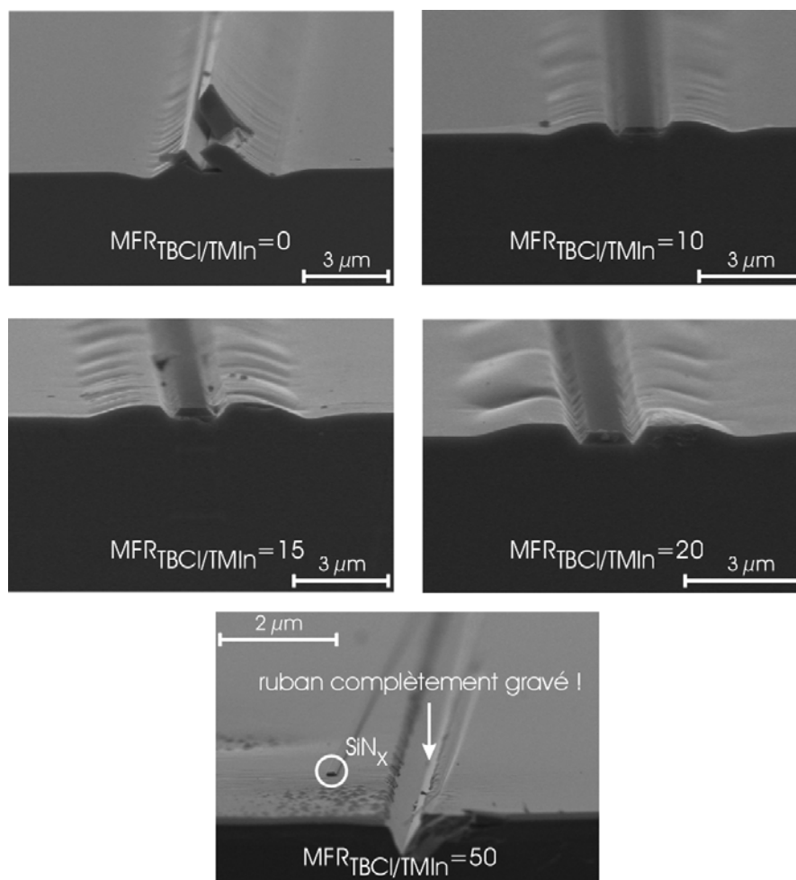
Fig. I-37 : Images MEB d'un ruban de 3\ \mu\text{m} de hauteur repris en MOVPE à 670^{\circ}\text{C} - 100\text{ mbar} avec adition progressive de TBCL.
