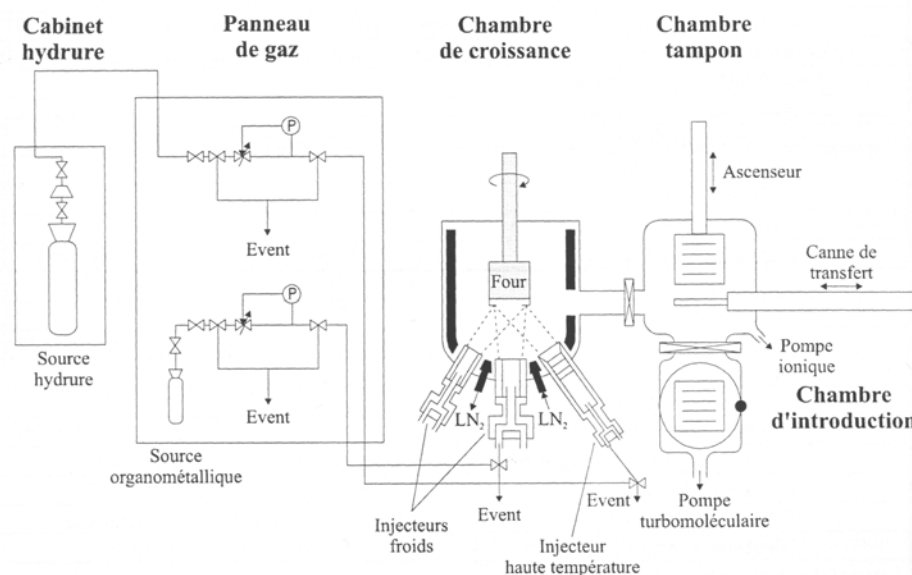
Fig. I-5 : Schéma de principe d'un réacteur CBE.
