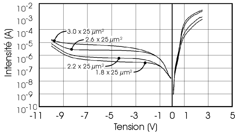
Fig. IV-8 : Mesures I(V) de courants de fuite sur plaque entière de modulateurs SIBH de 25 \mu\text{m} de long en fonction de la largeur du ruban (1.8 à 3 \mu\text{m} ). Les mesures sont donc limitées par l'isolation électrique entre les modulateurs sur le même ruban.
