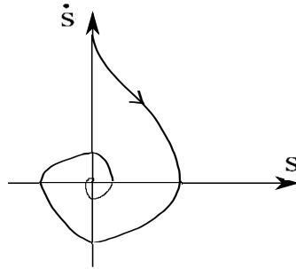
FIG. 3.2: Algorithme du twisting.
