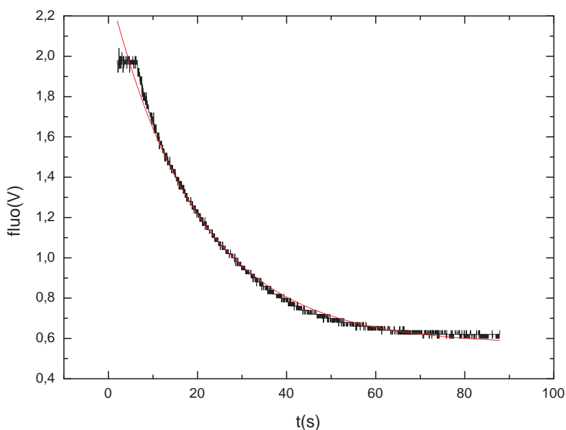
Figure 4.8 — Durée de vie du piège magnéto-optique 3D après installation du piège magnéto-optique 2D sur l'expérience. Un ajustement par une exponentielle donne une durée de vie de 17 secondes.
