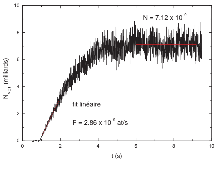
Figure 4.7 — Chargement du piège magnéto-optique 3D après installation du piège magnéto-optique 2D sur l'expérience. La mesure de la pente en début de chargement donne directement une mesure du flux d'atomes du piège magnéto-optique 2D. On trouve F = 2.86 \cdot 10^9 \text{ at.s}^{-1} .
