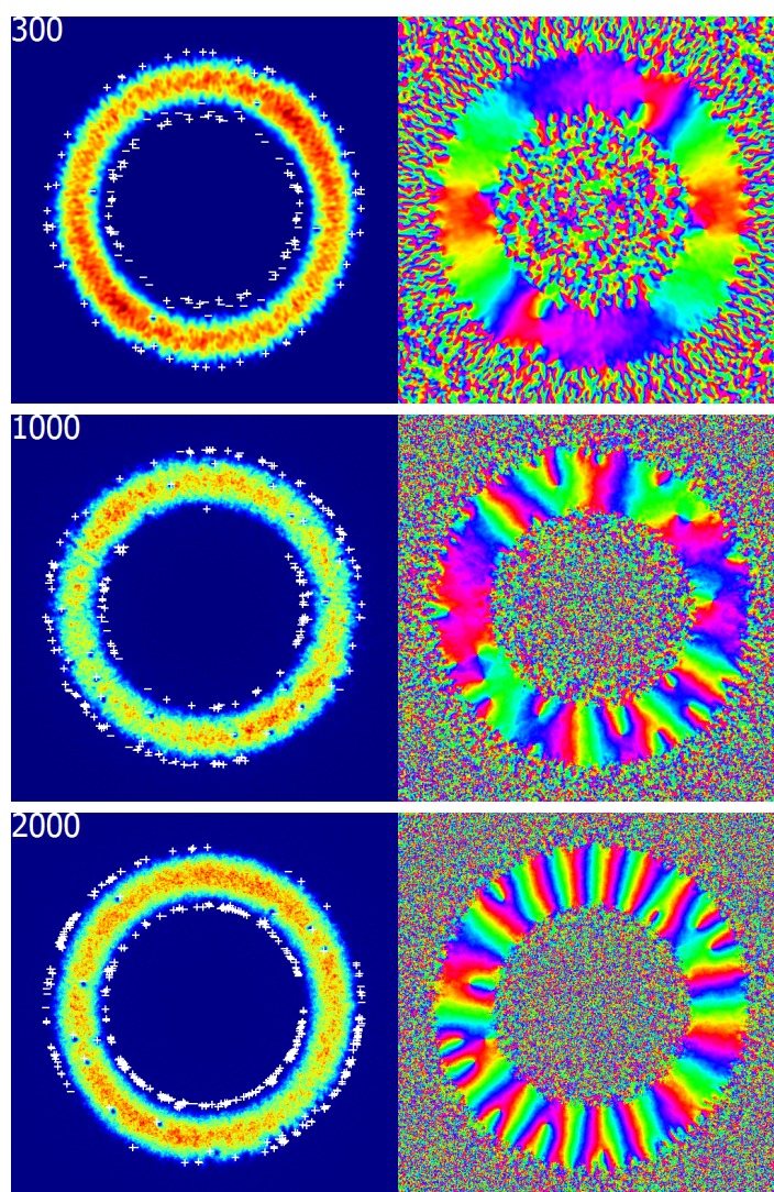
Figure 5.18 — Déformation elliptique en rotation. Les paramètres sont \mu = 8 , r_0 = 20 , \epsilon = 0.0125 et \Omega_{\text{rot},f} = 0,14 . Les trois images montrent la densité et la phase de la fonction d'onde aux instants t = 300, t = 1000 et t = 2000 . Sur la première image, quelques anti-vortex sont rentrés dans l'épaisseur de l'anneau par l'intérieur, et la circulation au milieu de l'anneau est nulle. Sur les deux images suivantes, on constate une circulation non nulle en observant la phase.
