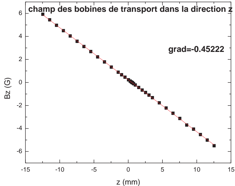
Figure 2.7 — Mesure du champ magnétique B_z dans l'axe des bobines en fonction de la hauteur z . La mesure a été réalisée avec un courant de 4 A, et renormalisée pour que la pente corresponde au gradient pour une intensité de 1 A. Le gradient mesuré est de 0,45\text{G}\cdot\text{mm}^{-1} , soit 4,5\text{G}\cdot\text{cm}^{-1}
