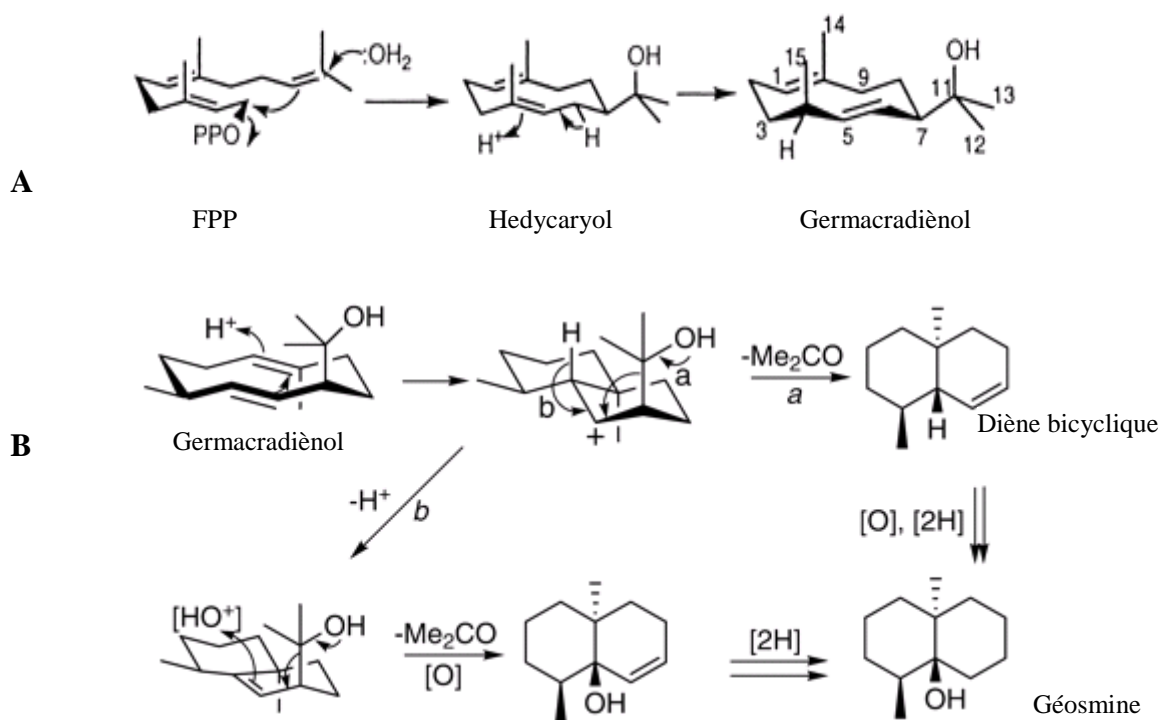
Figure 8. A-cyclisation du FPP catalysée par la sesquiterpène synthase de S. coelicolor ; B-mécanisme de conversion du germacradiénol en géosmine, d'après Cane et Watt (2003)
