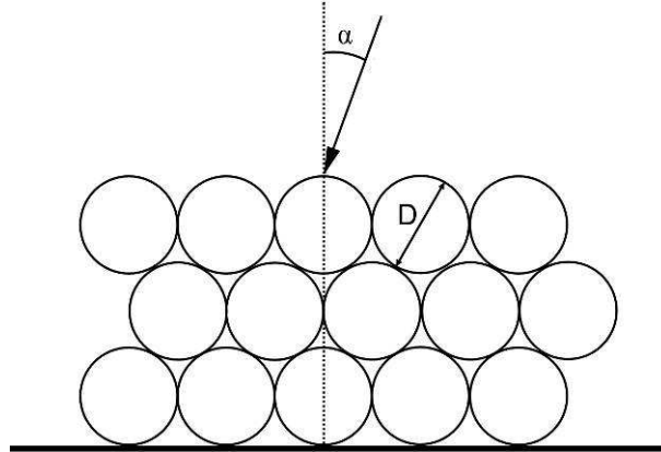
Figure 3.41. Illustration d'un cristal photonique colloïdale et d'un faisceau incident.
