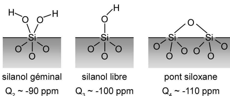
Figure 3.35. Illustration de l'environnement des atomes de silicium de type \text{Q}_2 , \text{Q}_3 et \text{Q}_4 dans la silice ainsi que les déplacements chimiques généralement observés pour ces noyaux (en considérant une référence de TMS).
