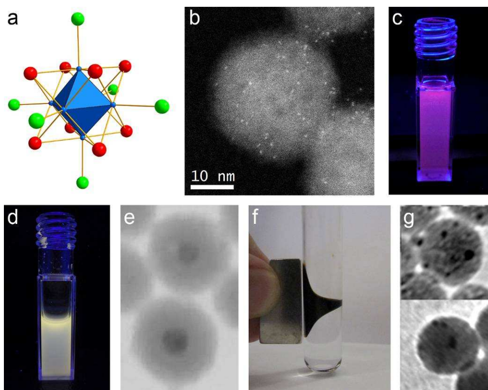
Figure C.1. Galerie des matériaux synthétisés au cours de cette thèse, avec : la représentation schématique d'un motif à cluster octaédrique (a), une image HAADF-STEM de nanoparticules de K_4[Re_6S_8(OH)_6]@SiO_2 (b), la luminescence de nanoparticules de Cs_4[Re_6S_8Br_6]@SiO_2 dispersées dans de l'eau (c), des nanoparticules de ZnO-Cs_2[Mo_6Br_{14}]@SiO_2 avec des propriétés d'émission modulables (d), une image STEM de nanoparticules de NaYF_4:Er/Yb-Cs_2[Mo_6Br_{14}]@SiO_2 aux propriétés d'upconversion (e), un colloïde de nanoparticules de \gamma -Fe 2 O 3 superparamagnétiques qui ont ensuite été associées avec des clusters dans des nanoparticules de silice (f), des nanocristaux d'argent et d'or décorant des nanoparticules de Cs_2[Mo_6Br_{14}]@SiO_2 qui ont joué le rôle de réducteur (g).
