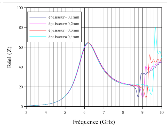
Figure 4.68: Influence du paramètre " afente " sur Réel(Z)
