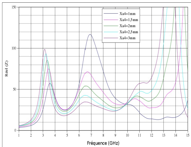
Figure 2.55: Influence du paramètre "Xa4" sur Réel Z
