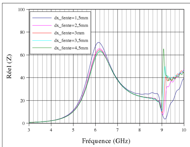
Figure 4.65: Influence du paramètre "dx_fente" sur Réel(Z)
