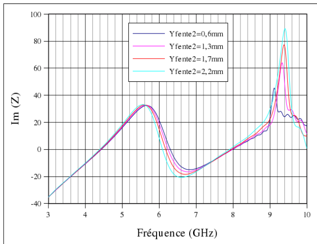
Figure 4.63: Influence du paramètre "Yfente2" sur Im(Z)
