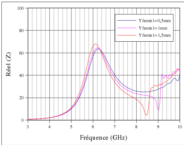
Figure 4.60: Influence du paramètre "Yfente1" sur Réel(Z)
