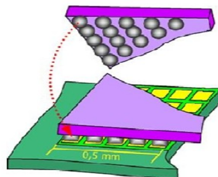
Figure 3.5: Illustration montrant une photo prise par microscope électronique ainsi que la dernière étape de la méthode "Flip-Chip"
