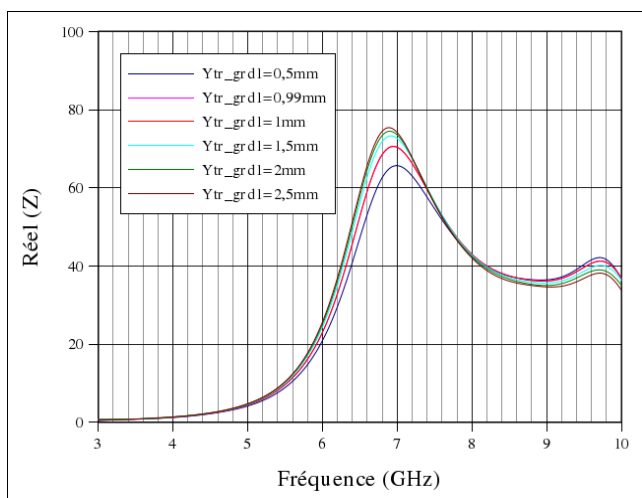
Figure 4.34: Influence du paramètre " Ytr_grd1 " sur Réel( Z )
