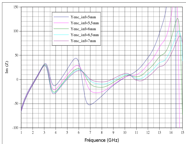
Figure 2.46: Influence du paramètre "Yenc_inf" sur ImZ
