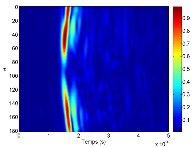
Figure 3.81: Réponse temporelle du prototype "carte de crédit" dans le plan XOZ
