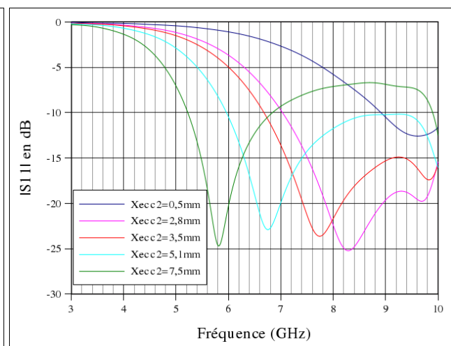
Figure 4.37: Influence du paramètre "Xecc2" sur l'amplitude du coefficient de réflexion
