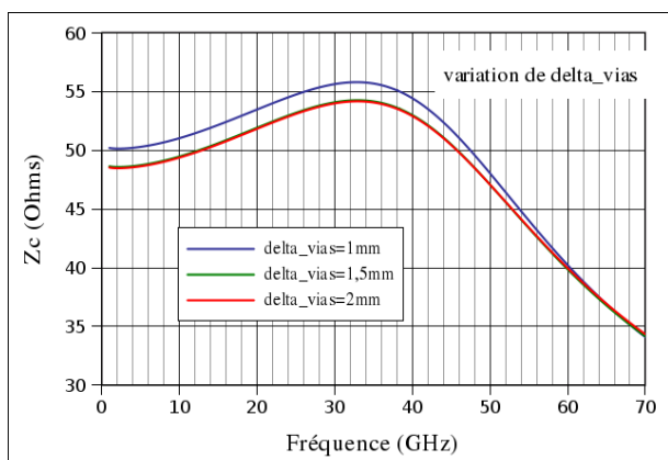
Figure 2.16: Influence du paramètre " delta\_vias " sur l'impédance caractéristique de la GCPW avec vias
