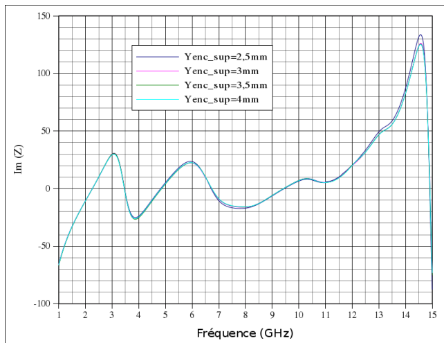
Figure 2.40: Influence du paramètre "Yenc_sup" sur ImZ
