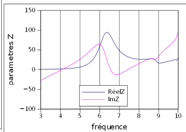
Figure 3: Paramètres Z de la structure 3D ECC
