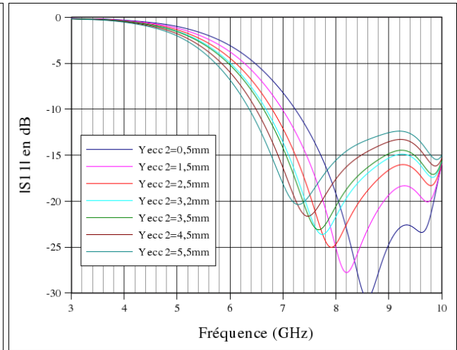
Figure 4.43: Influence du paramètre "Yecc2" sur le |S11|
