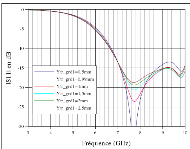
Figure 4.33: Influence du paramètre " Ytr_grd1 " sur l'amplitude du coefficient de réflexion
