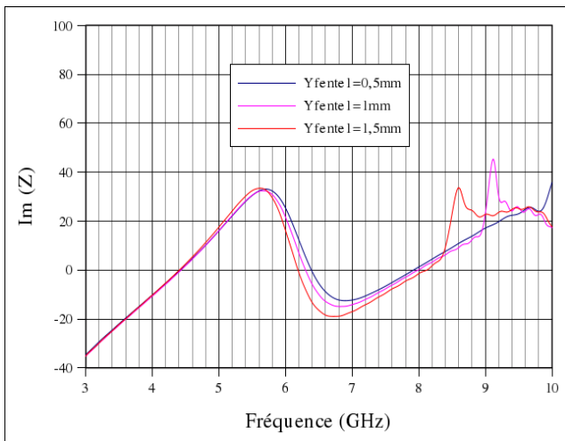
Figure 4.62: Influence du paramètre "Yfente1" sur Im(Z)
