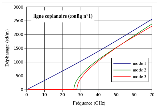
Figure 2.6: Modes générés de la ligne coplanaire 50 Ω
