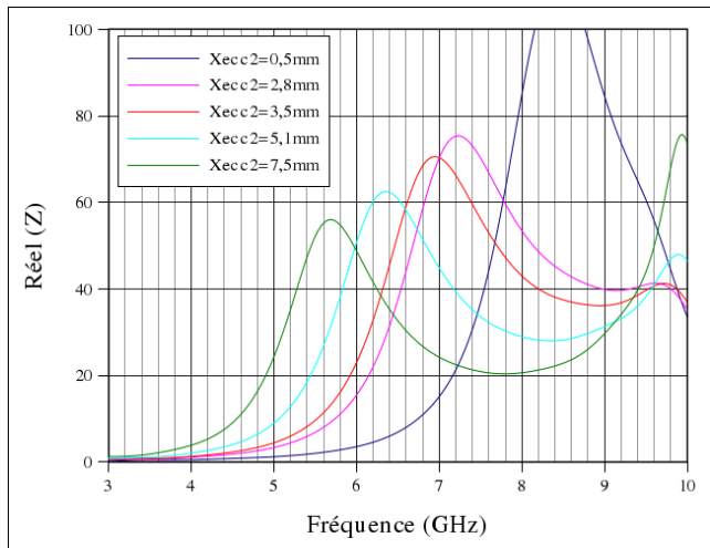
Figure 4.39: Influence du paramètre "Xeccc2" sur Réel(Z)
