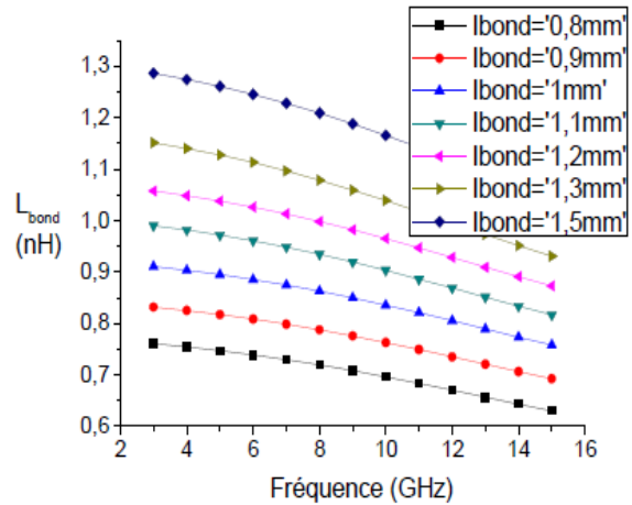
Figure 3.23: Extraction de l'inductance du modèle en "pi" en fonction de la longueur du wirebond
