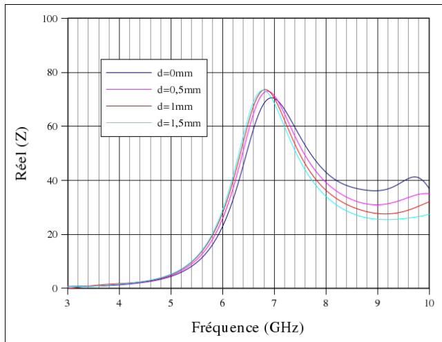
Figure 4.28: Influence du paramètre "d" sur Réel(Z)
