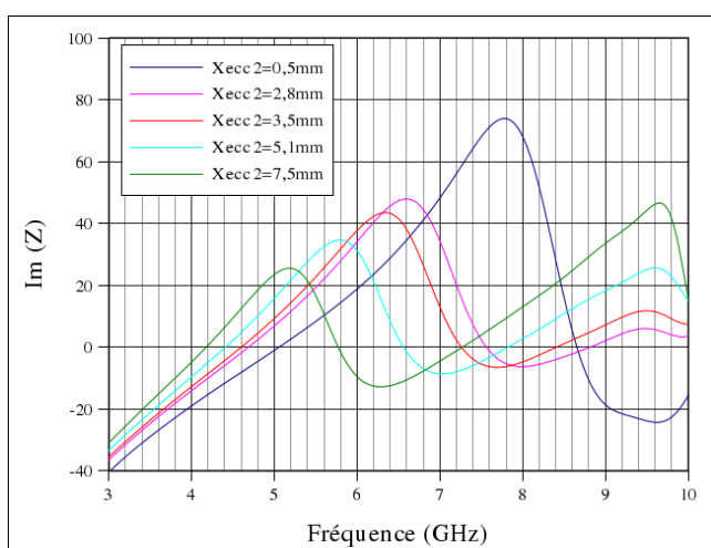
Figure 4.41: Influence du paramètre "Xeccc2" sur Im(Z)
