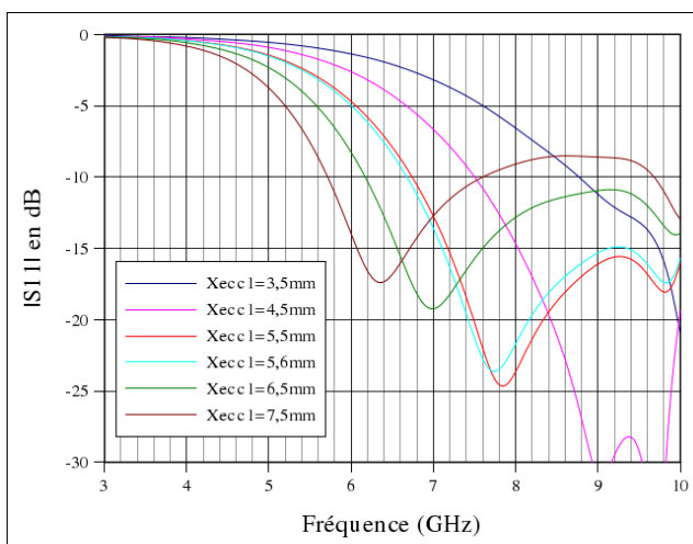
Figure 4.36: Influence du paramètre "Xecc1" sur l'amplitude du coefficient de réflexion
