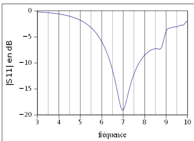
Figure 2: Amplitude du coefficient de réflexion de la structure 3D ECC
