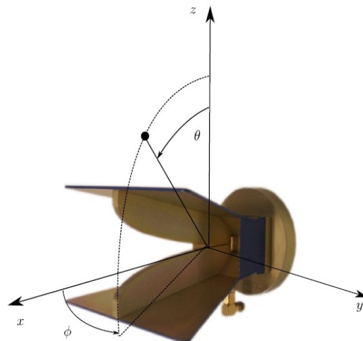
Figure 3.50: Antenne de référence (SH2000)
