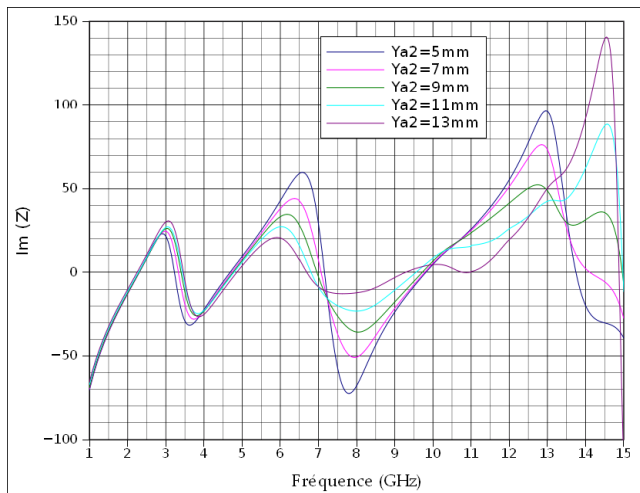
Figure 2.69: Influence du paramètre "Ya2" sur Im Z
