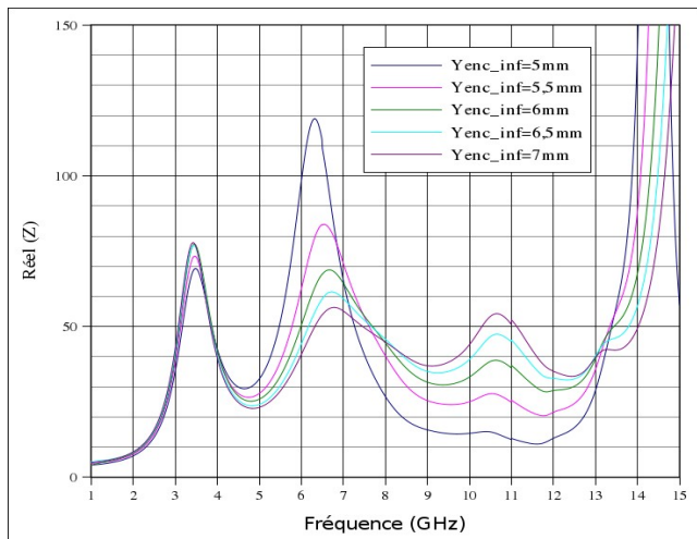
Figure 2.44: Influence du paramètre "Yenc_inf" sur RéelZ
