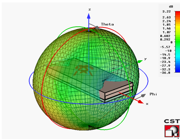
Figure 4.107: Gain réalisé (PCB = 0,7mm) à 8 GHz
