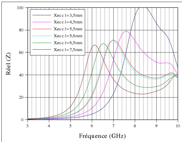
Figure 4.38: Influence du paramètre "Xeccc1" sur Réel(Z)
