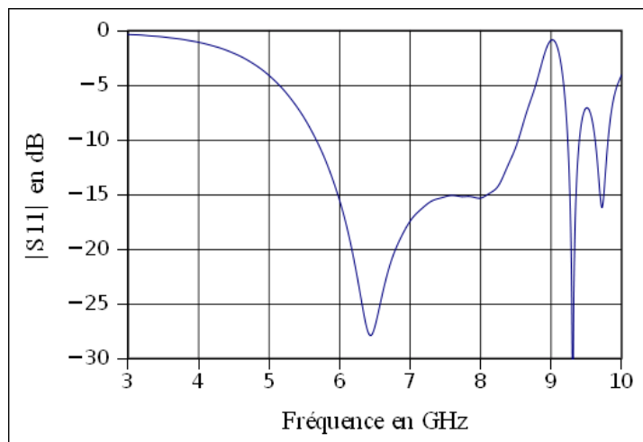
Figure 4.102: Amplitude du coefficient de réflexion de la structure ECC co designé après l'ajout des plots
