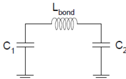
Figure 3.21: Illustration du modèle en "pi" d'un wirebond"
