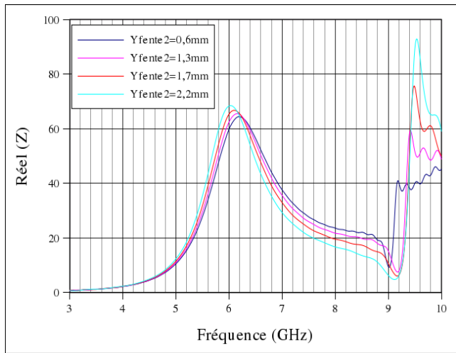
Figure 4.61: Influence du paramètre "Yfente2" sur Réel(Z)
