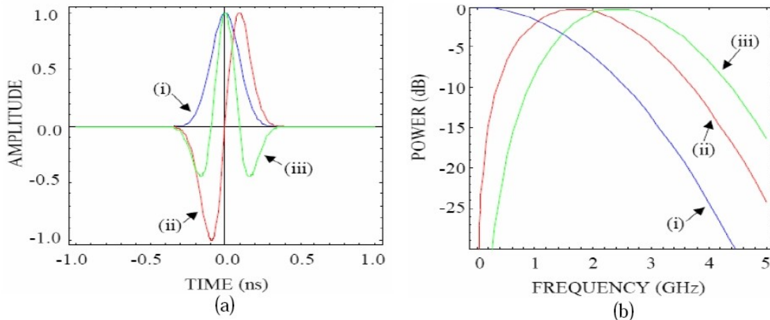
Figure 1.18: Les impulsions de forme Gaussienne et ses dérivées et leurs spectres fréquentiels
