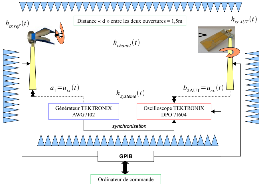
Figure 3.61: Système permettant de trouver la réponse impulsionnelle de l'antenne AUT (USB Key)
