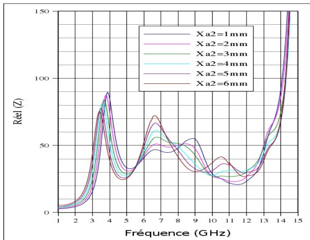
Figure 2.53: Influence du paramètre "Xa2" sur Réel Z
