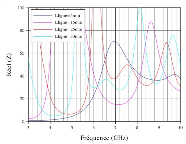
Figure 4.22: Influence du paramètre " Lligne " sur Réel( Z )
