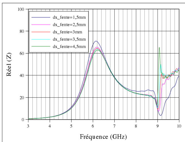
Figure 4.65: Influence du paramètre "dx_fente" sur Réel(Z)
