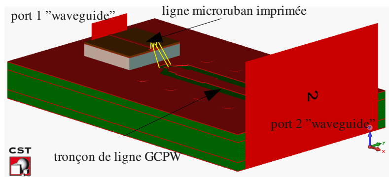
Figure 3.6: Illustration du bloc puce + substrat + tron  on de ligne GCPW mod  lis   avec CST Microwave Studio
