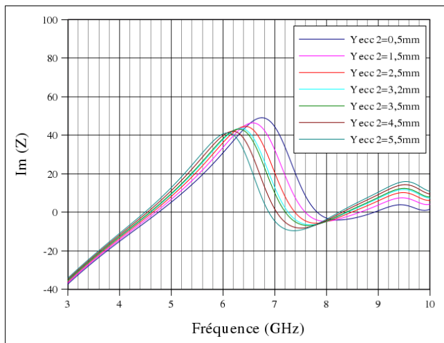
Figure 4.47: Influence du paramètre "Yecc2" sur Im(Z)
