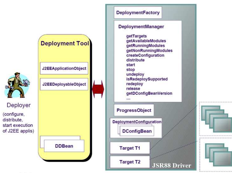
FIG. 2.17 – Architecture de déploiement d'un serveur JEE
