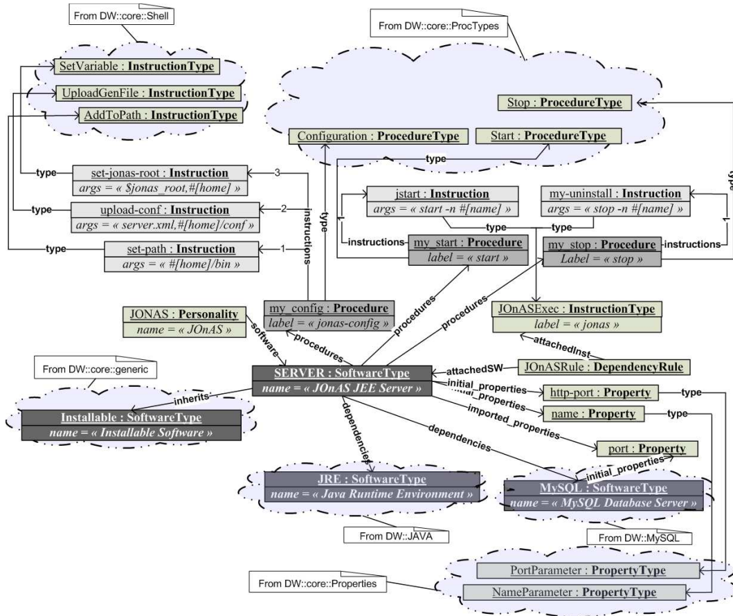
FIG. 4.4 – Modélisation de logiciel avec DeployWare : le serveur JEE JOnAS
