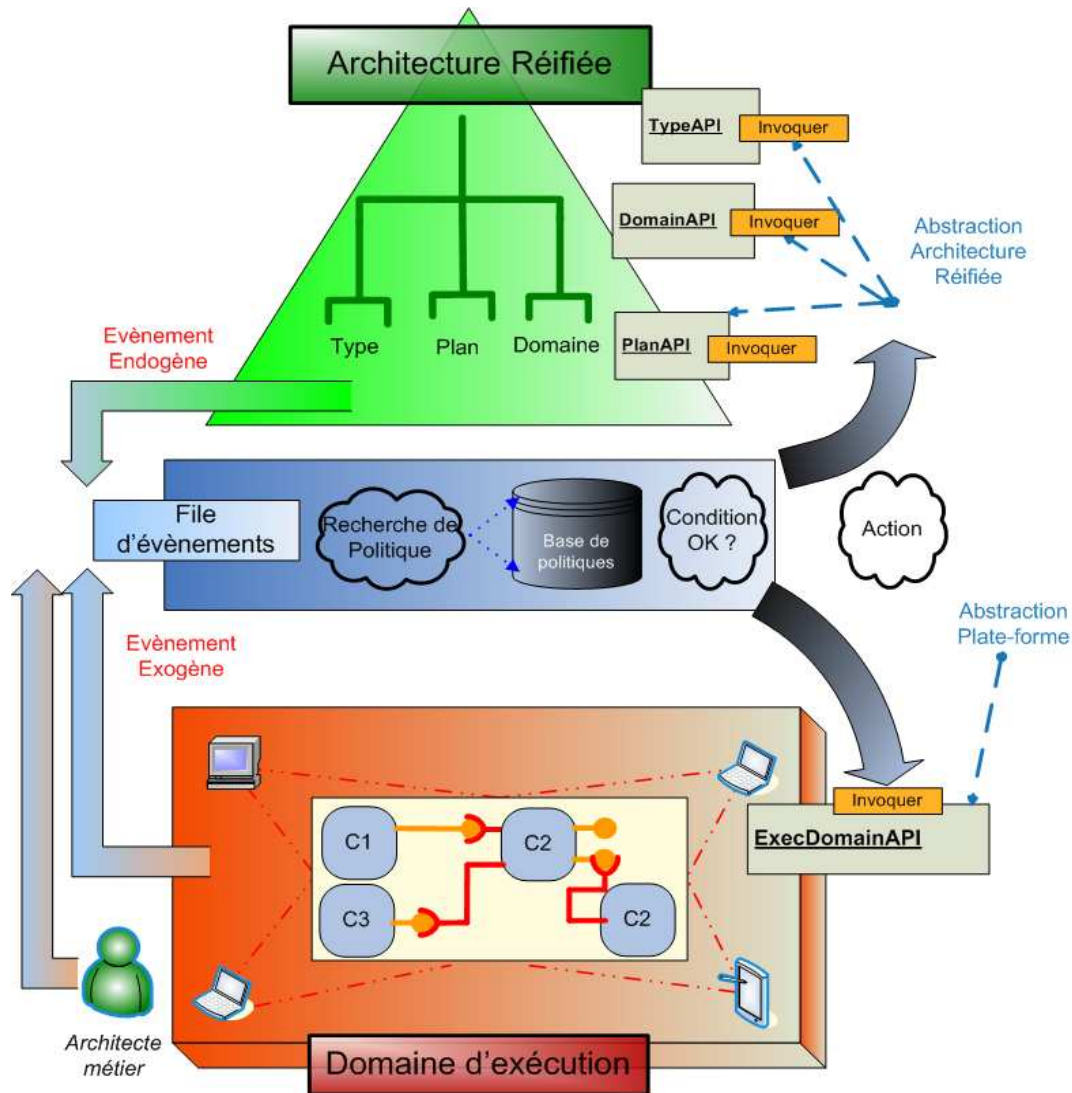
FIG. 6.3 – Vue d'ensemble du prototype DACAR
