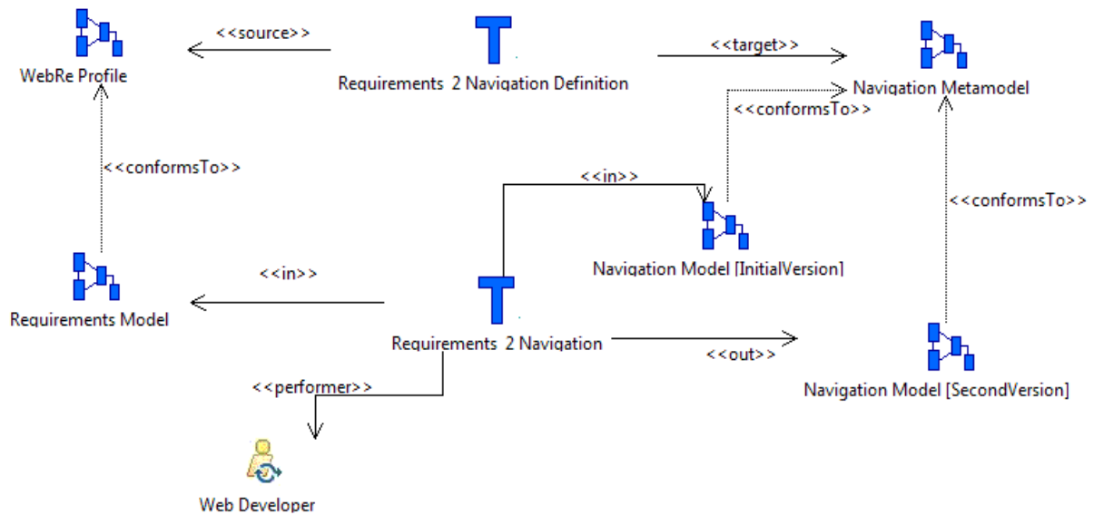
Figure V.9 La transformation « Requirements 2 Navigation » et sa définition
