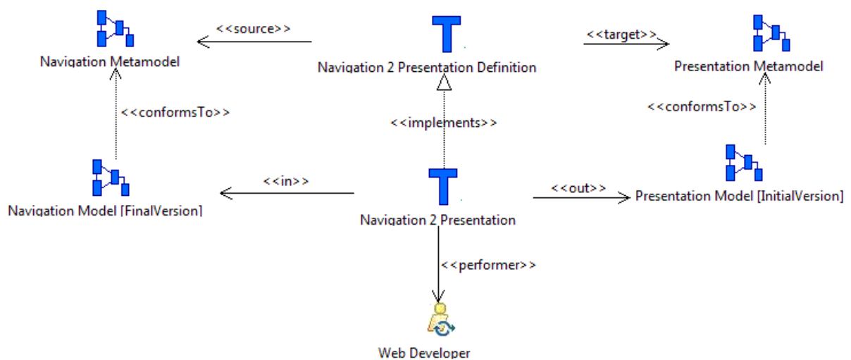
Figure V.11 La transformation « Navigation 2 Presentation » et sa définition
