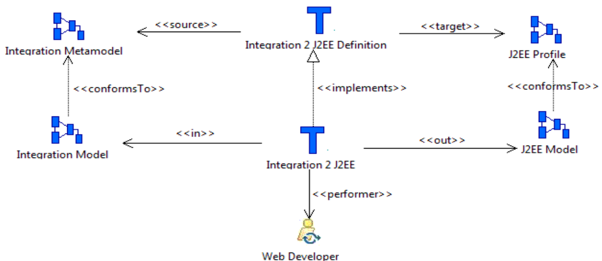
Figure V.15 La transformation « Integration 2 J2EE » et sa définition
