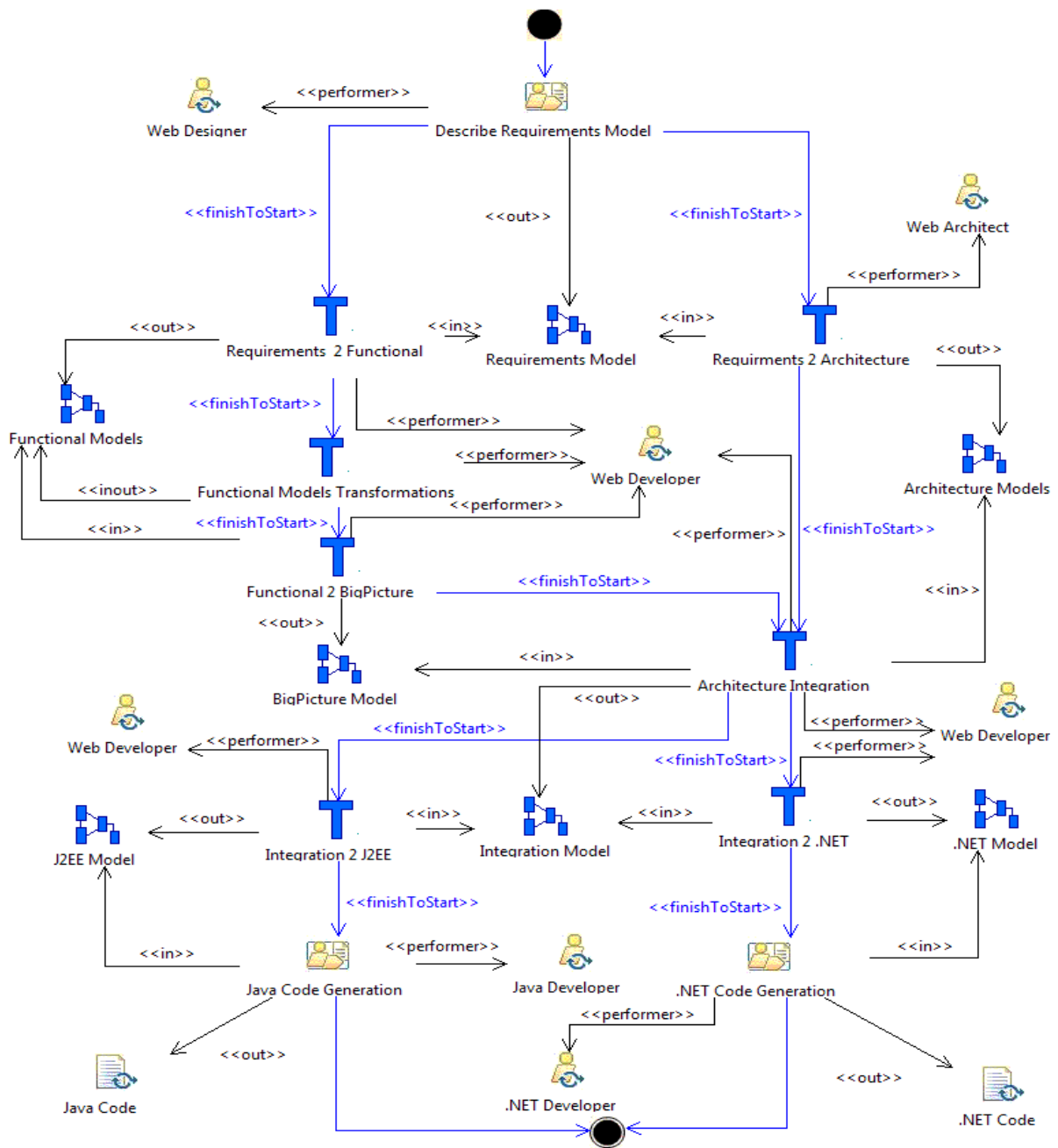
Figure V.3 Description structurelle du Processus UWE
