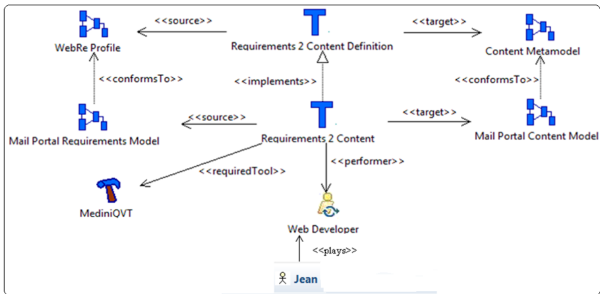
Figure V.20 Adaptation de la transformation « Requirements 2 Content »
