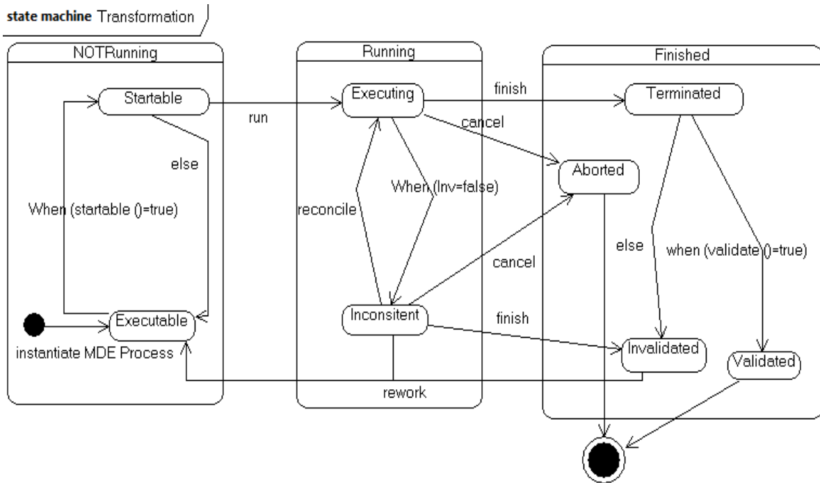
Figure V.18. Rappel du comportement d'une transformation du processus UWE
