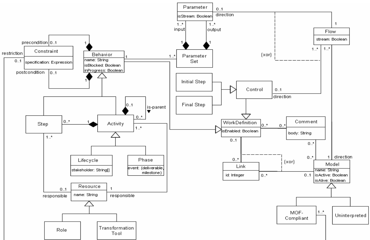
Figure II.18 Le métamodèle de l'approche de Porres [Porres et al, 2006]
