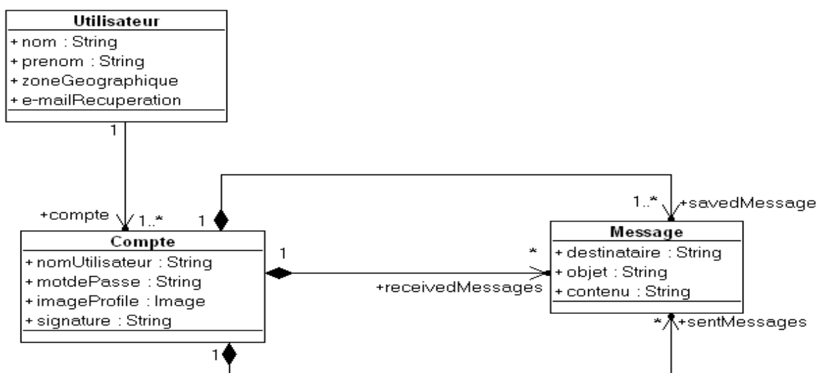
Figure V.35 Modèle de contenu produit par la transformation « Requirements 2 Content »
