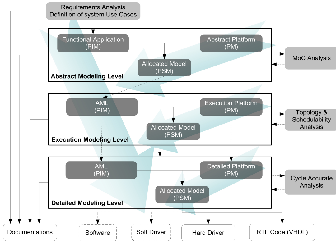
Figure II.15 Vue d'ensemble du processus MoPCoM [Koudri, 2010]
