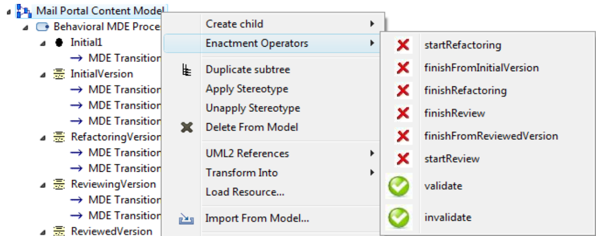
Figure V.38 État des opérateurs du modèle du contenu après son passage à l'état « FinalVersion »
