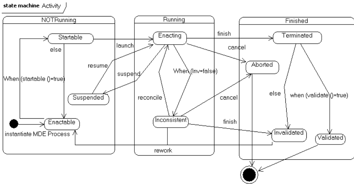
Figure V.17. Rappel du comportement de l'activité « Describe Requirements Model »
