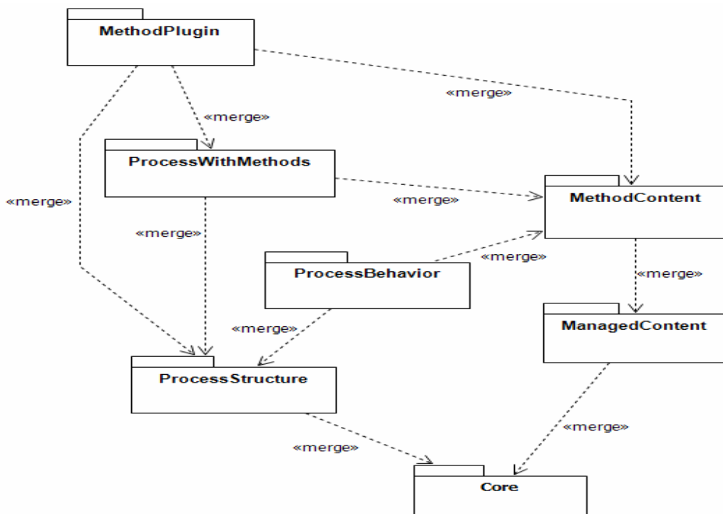
Figure II.4 Structure du métamodèle de SPEM 2.0 [OMG-SPEM 2.0, 2008]
