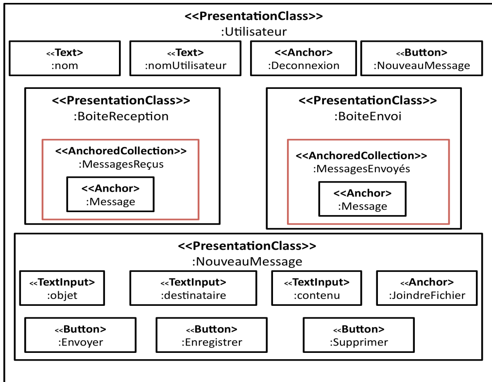
Figure V.41 Modèle de présentation de la classe « Utilisateur »
