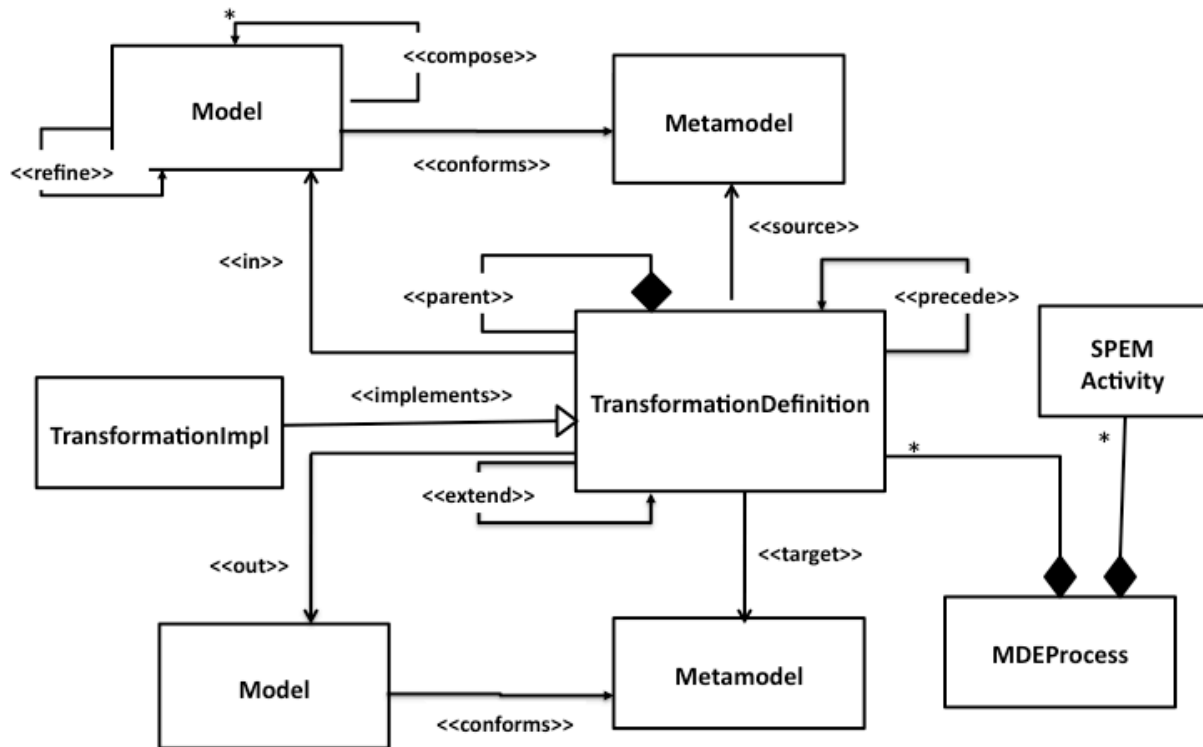
Figure III.2. Modèle conceptuel de l'approche adoptée dans SPEM4MDE
