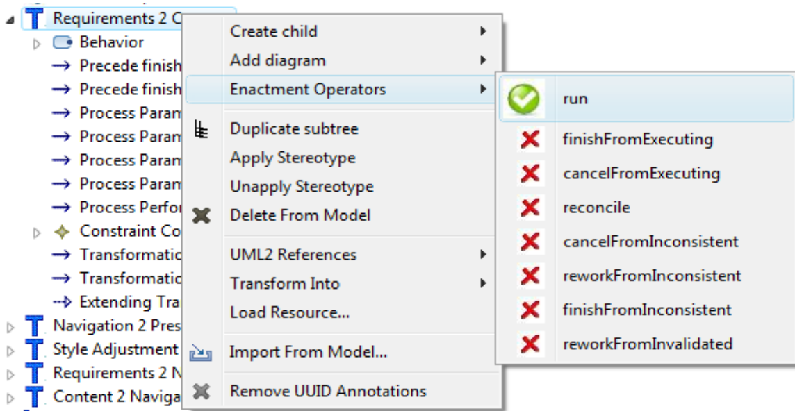
Figure V.32 État des opérateurs de mise en œuvre de « Requirements 2 Content » après son passage à l'état « Startable »
