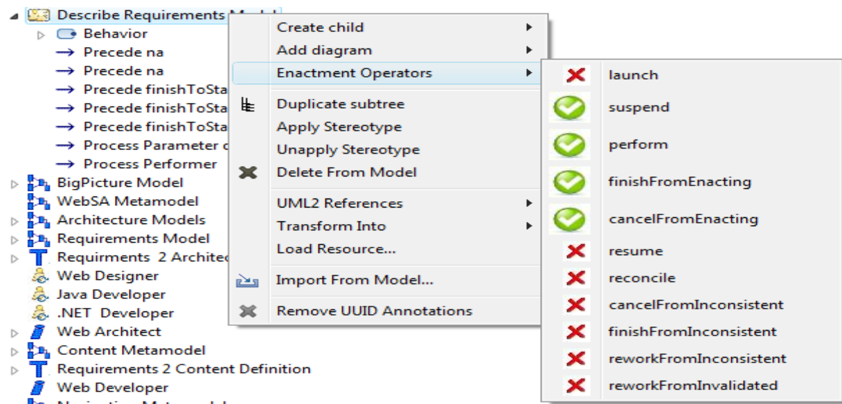
Figure V.25 État des opérateurs de mise en œuvre de l'activité « Describe Requirements Model » après son lancement
