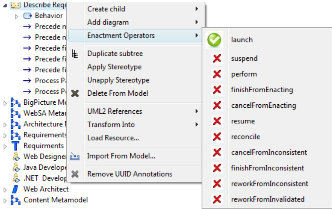
Figure V.23 Opérateurs de mise en œuvre de l'activité « Describe Requirements Model »
