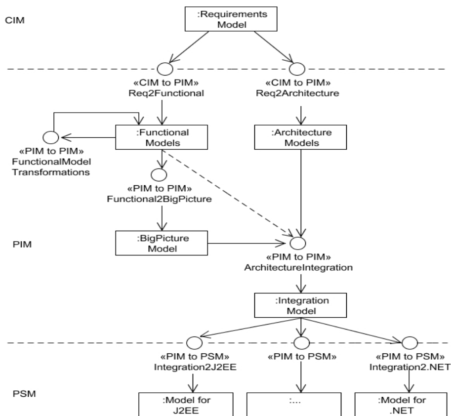
Figure II.11 Vue d'ensemble du processus UWE [Koch, 2006]
