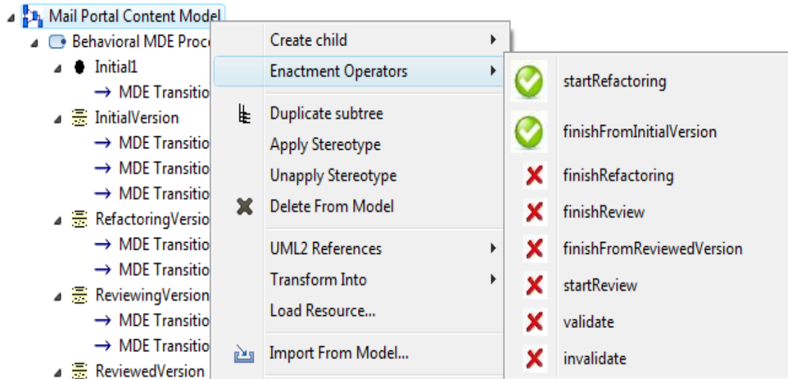
Figure V.36 État des opérateurs du modèle du contenu après son passage à l'état « InitialVersion »
