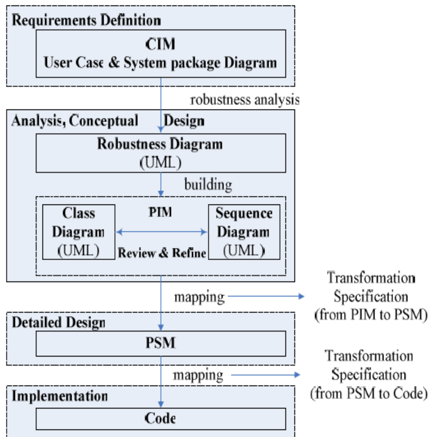
Figure II.13 Le processus IDM dédié à la plate-forme E-learning [Cong et al., 2010]
