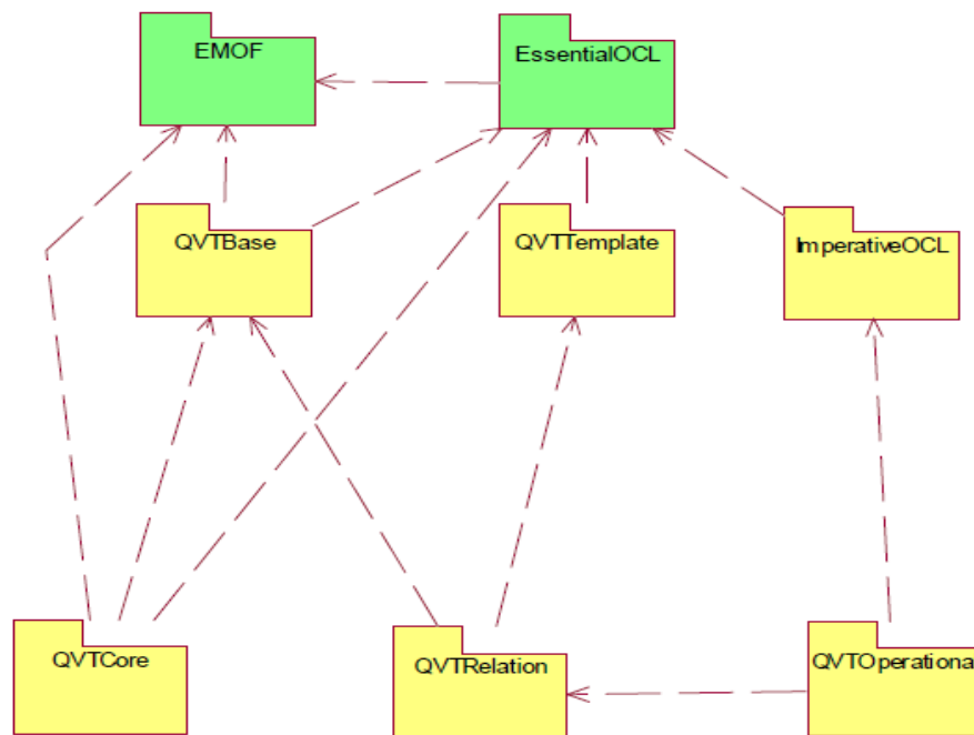
Figure III.6 La structuration en paquetages de MOF 2.0 QVT [OMG-QVT, 2008]
