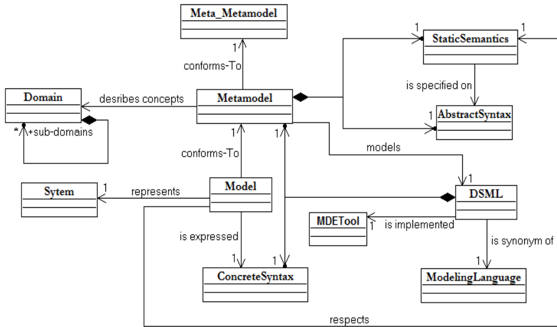
Figure II.2 Notions de base en ingénierie des modèles
