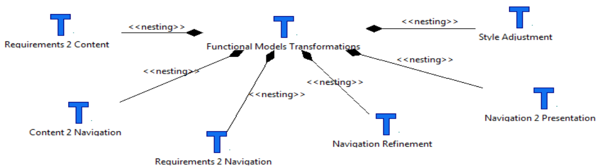
Figure V.4 Les transformations des modèles fonctionnels du processus UWE
