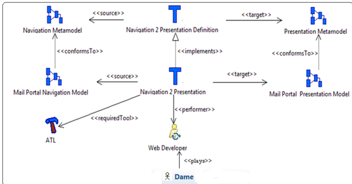
Figure V.22 Adaptation de la transformation « Navigation 2 Presentation ».
