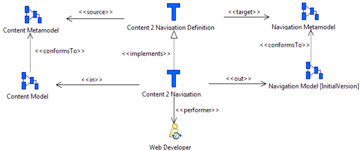
Figure V.8 La transformation « Content 2 Navigation » et sa définition
