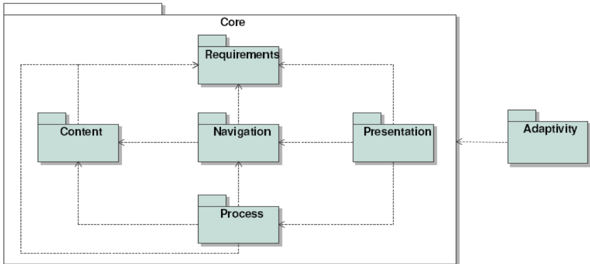
FIG. 5 Les paquets du métamodèle UWE [Kroiß et al., 2008]
