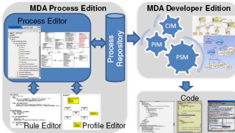
Figure II.17 Vue d'ensemble de l'environnement Transforms [Maciel et al., 2009]
