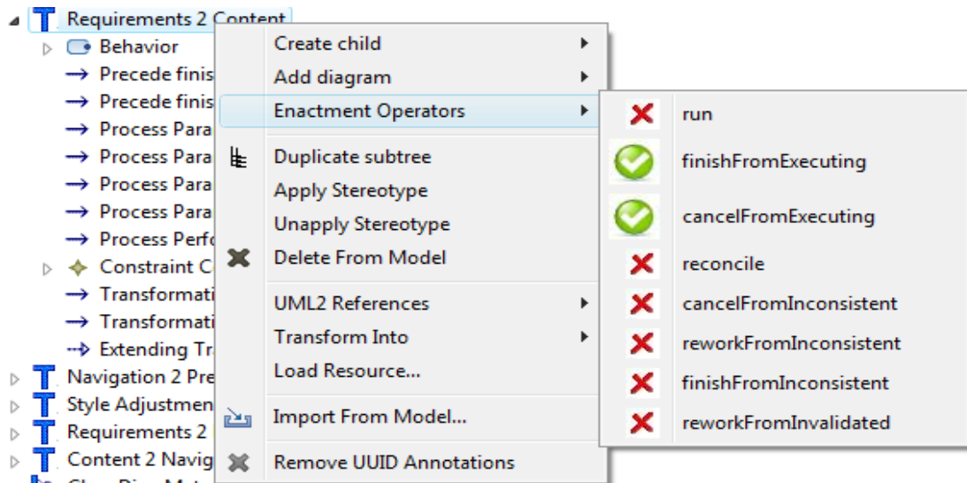
Figure V.34 État des opérateurs de mise en œuvre après l'exécution de l'opérateur « run ».
