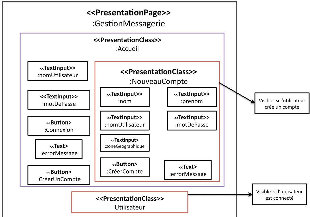
Figure V.40 Modèle de présentation produit par la transformation « Navigation 2 Presentation »
