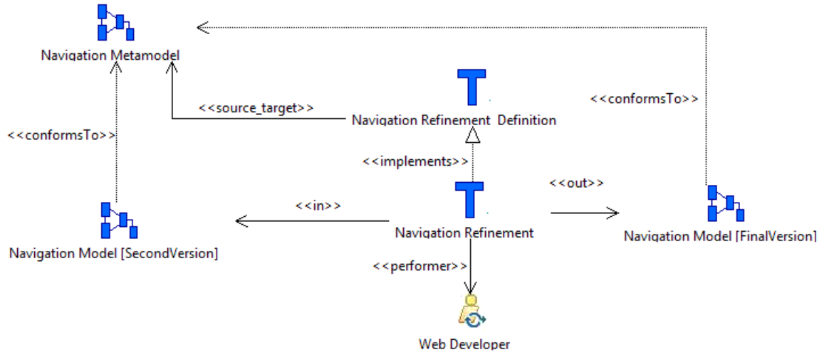
Figure V.10 La transformation « Navigation Refinement » et sa définition
