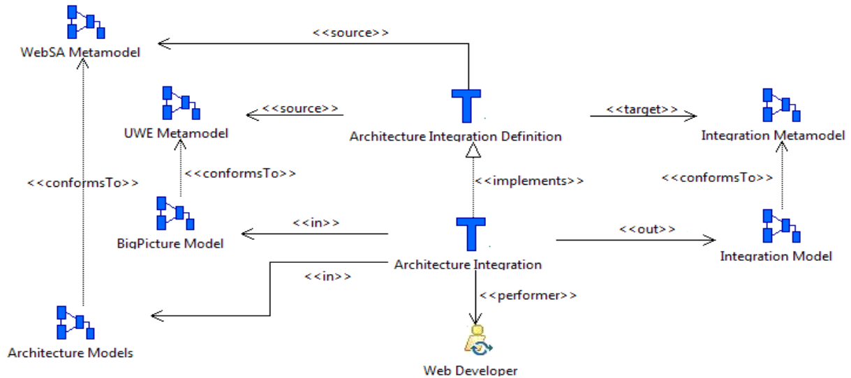
Figure V.14 La transformation « Architecture Integration » et sa définition
