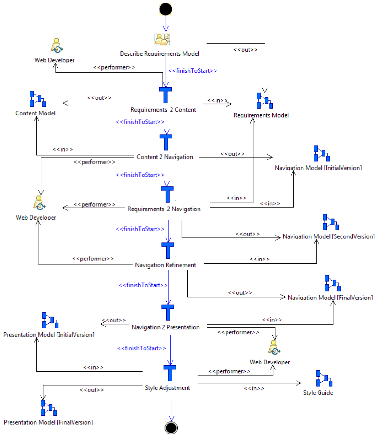
Figure V.6 Enchaînement des transformations des modèles fonctionnels
