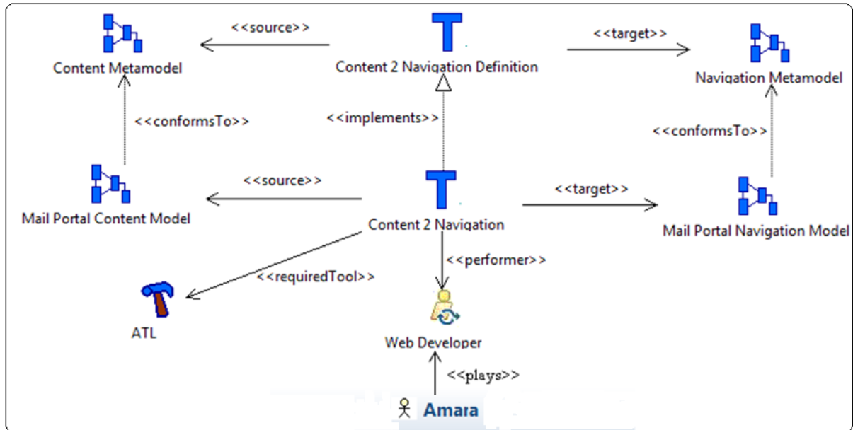
Figure V.21 Adaptation de la transformation « Content 2 Navigation »
