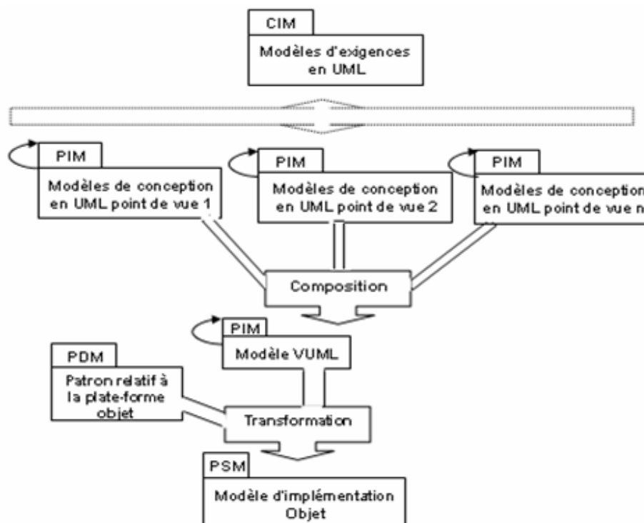
Figure II.14 Processus de composition structurelle dans VUML [Anwar et al., 2010]
