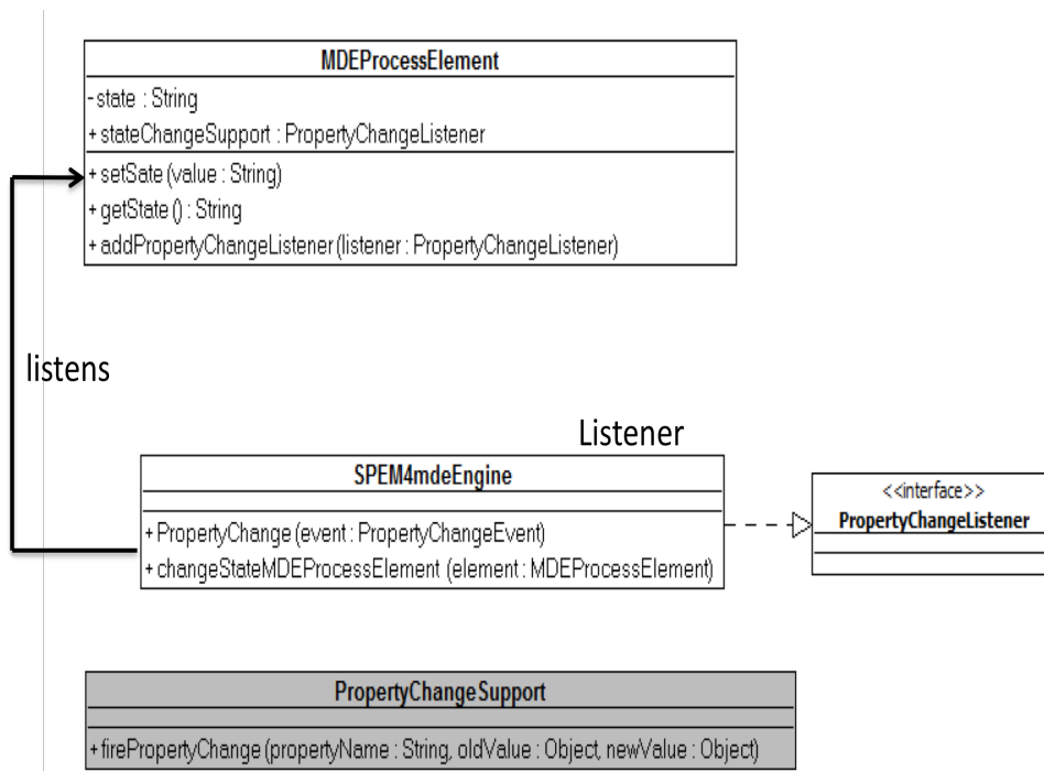
Figure IV.21 Mécanisme d'écoute et de traitement d'un événement de changement d'état
