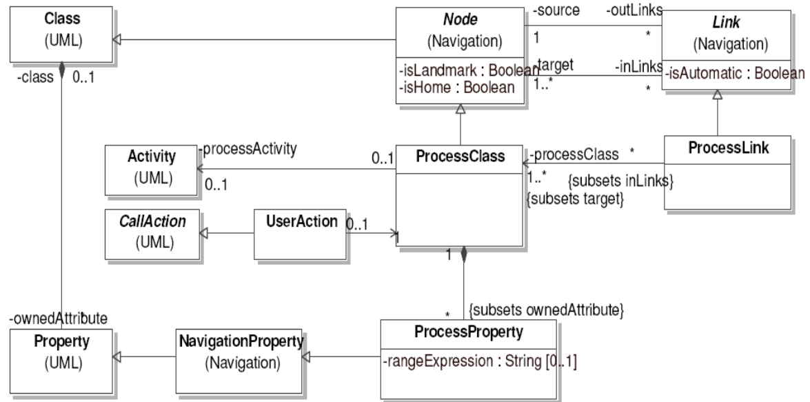
FIG. 10 Le paquetage « Process » [Kroiß et al., 2008]
