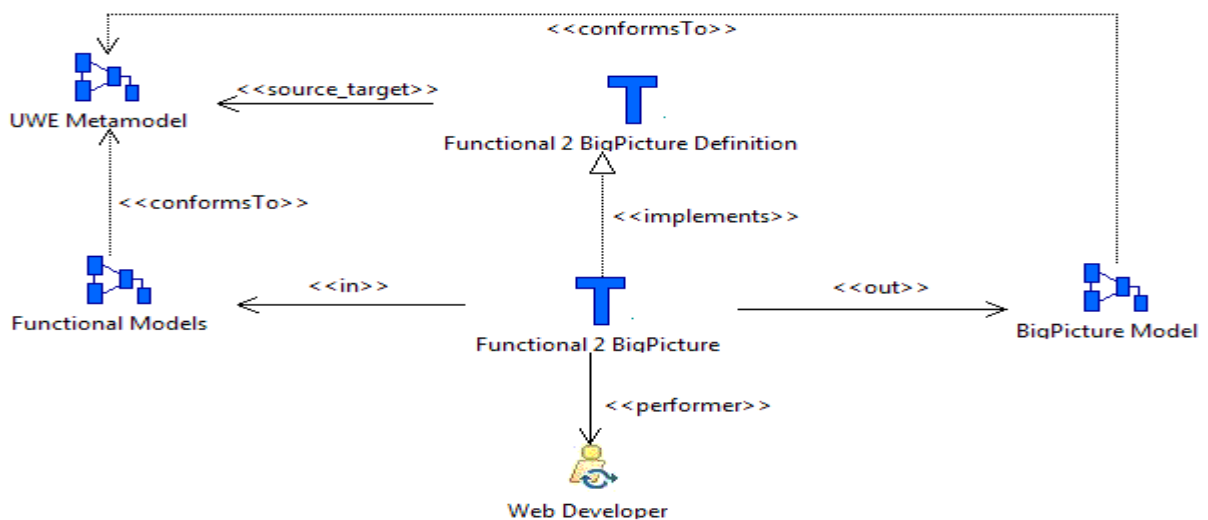
Figure V.13 La transformation « Functional2BigPicture » et sa définition
