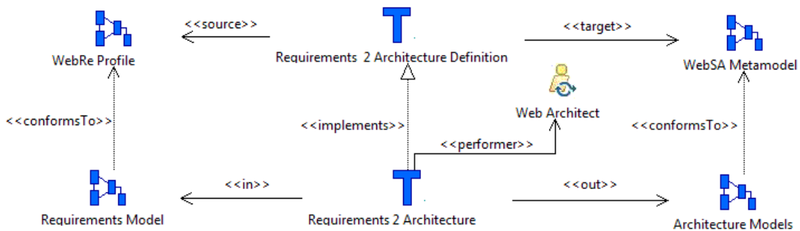
Figure V.5 Relations entre la transformation « Requirements 2 Architecture » et sa définition
