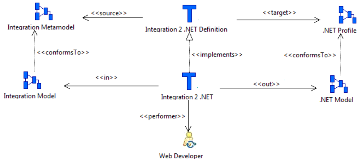
Figure V.16 La transformation « Integration 2 .NET » et sa définition
