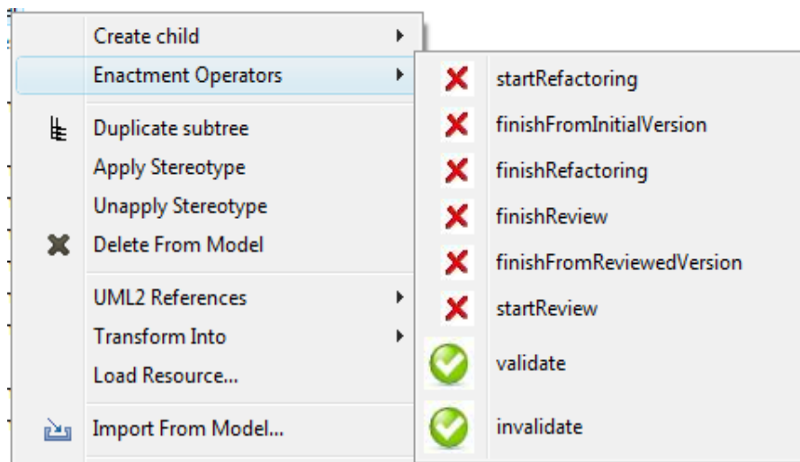
Figure V.29 État des opérateurs après le passage du modèle produit à l'état « FinalVersion »
