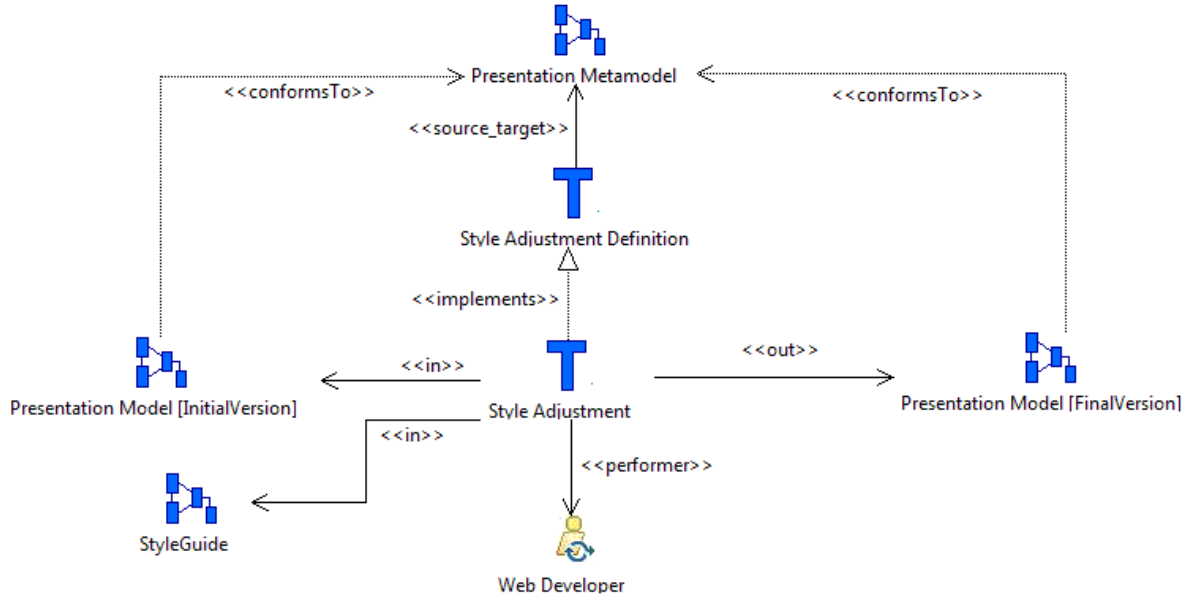
Figure V.12 La transformation « Style Adjustment » et sa définition
