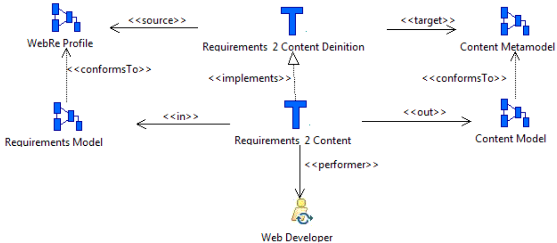
Figure V.7 Relations entre la transformation « Requirements 2 Content » et sa définition
