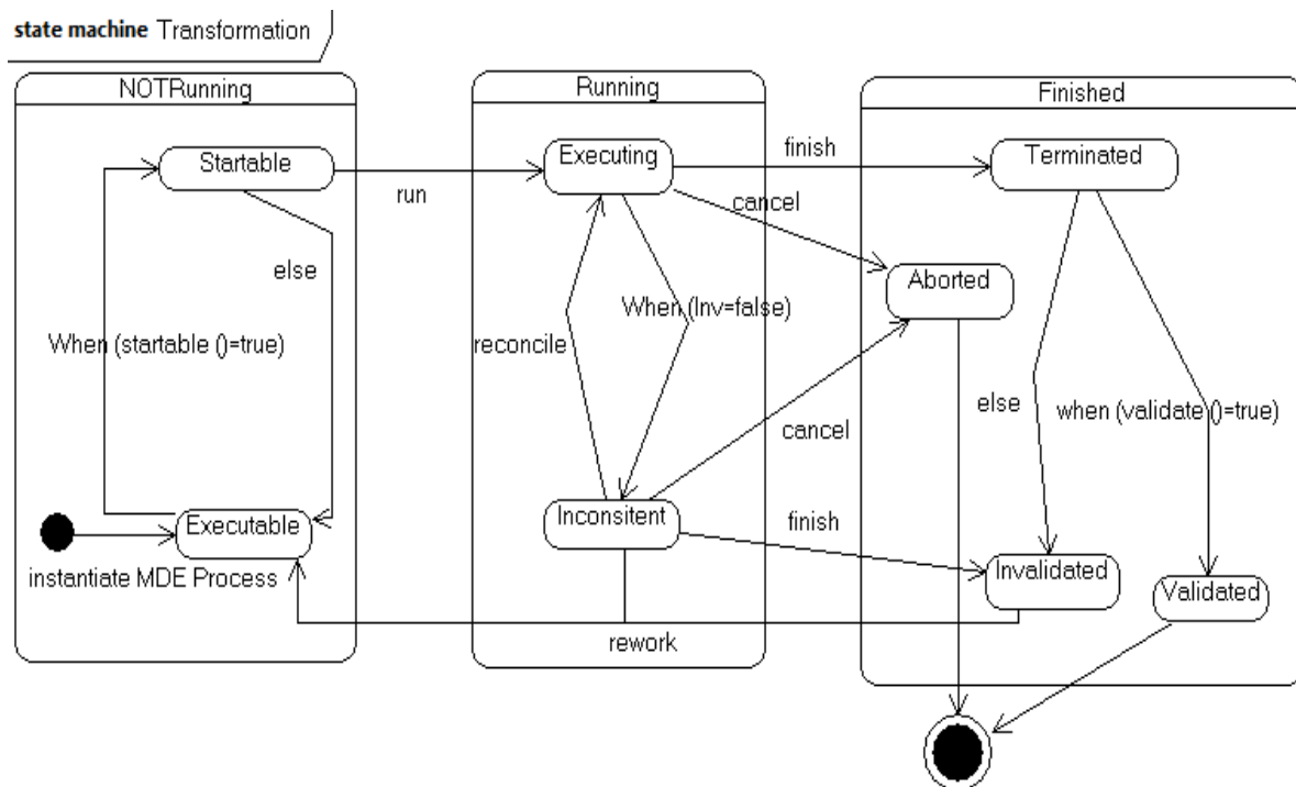
Figure III.8. Comportement par défaut d'une transformation
