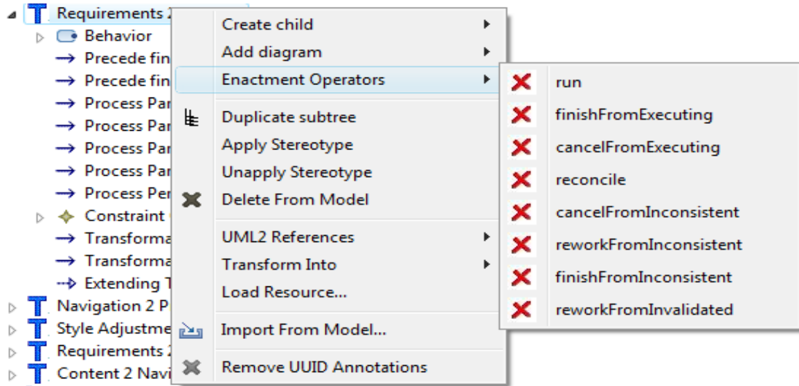
Figure V.30 Opérateurs de mise en œuvre de la transformation « Requirements 2 Content »
