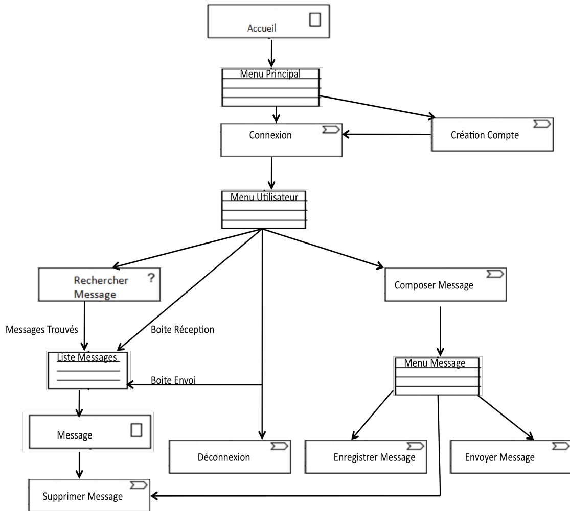
Figure V.39 Modèle de navigation produit par la transformation « Content 2 Navigation »
