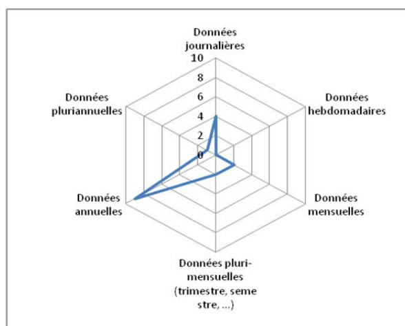
Graphique 20 - Discrétisation temporelle des données individuelles
