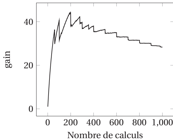
FIGURE 6.4 : Gain en fonction du nombre de calculs pour l'étude paramétrique sur l'ailette
