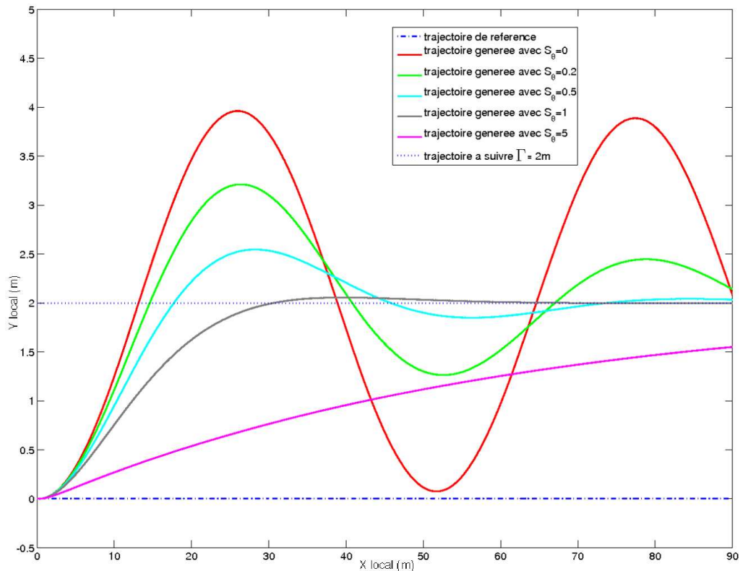
FIGURE 3.9 – Différentes prédictions de la trajectoire parallèle à celle de référence d'écart latéral \Gamma = 2m en fonction des valeurs de minimisation de l'écart angulaire S_{\theta}
