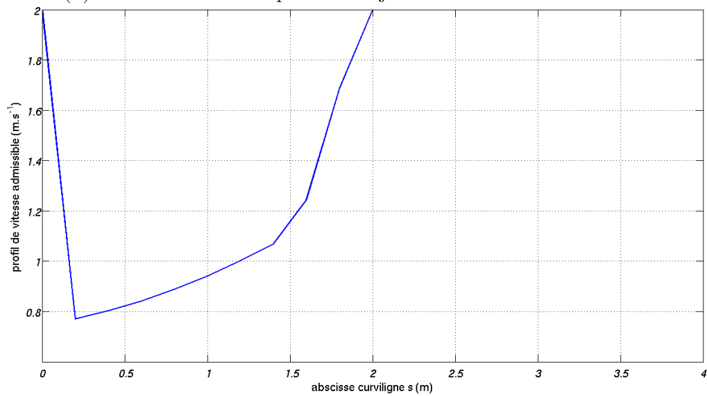
(b) Profil de vitesse associé
