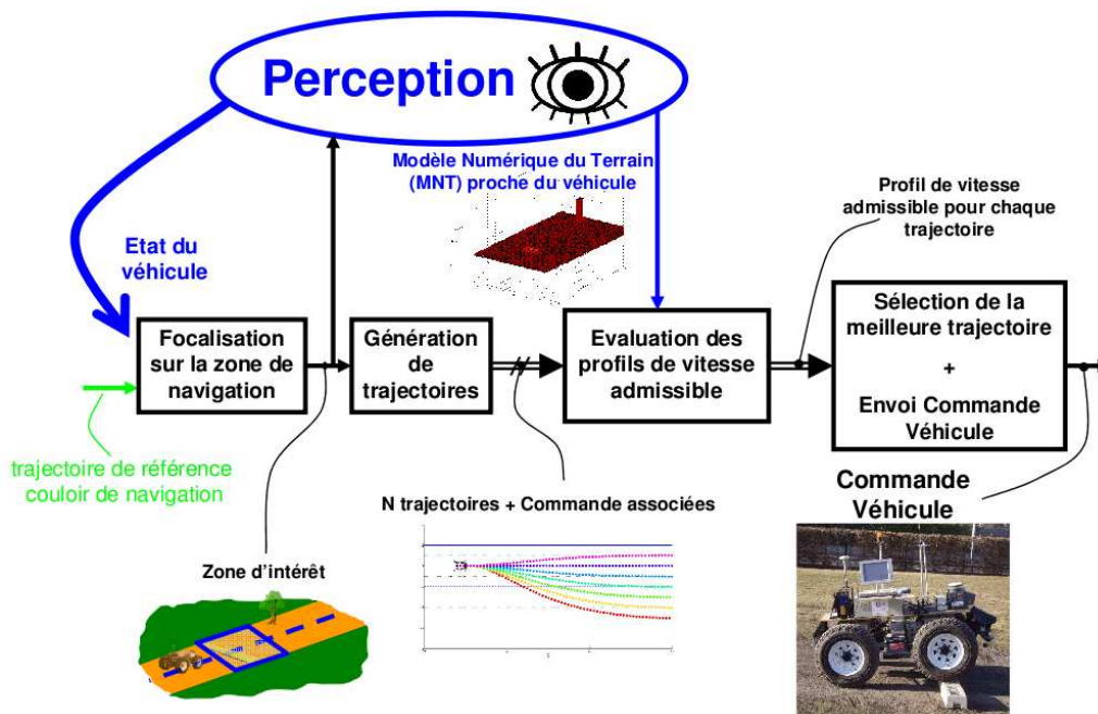
FIGURE 3.2 – Présentation des différentes étapes de notre système
