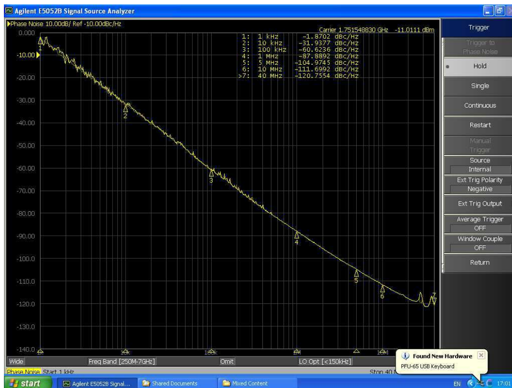
Figure 7-14 : Le bruit de phase dans l'oscillateur OSC_21_INV
