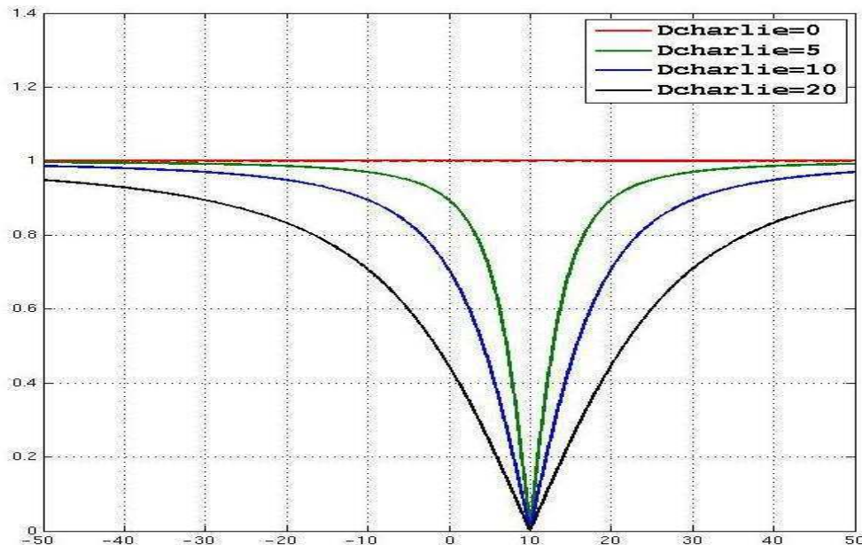
Figure 3-16 : La valeur absolue de la dérivée de Charlie(s) pour différentes valeurs de D_{charlie}
