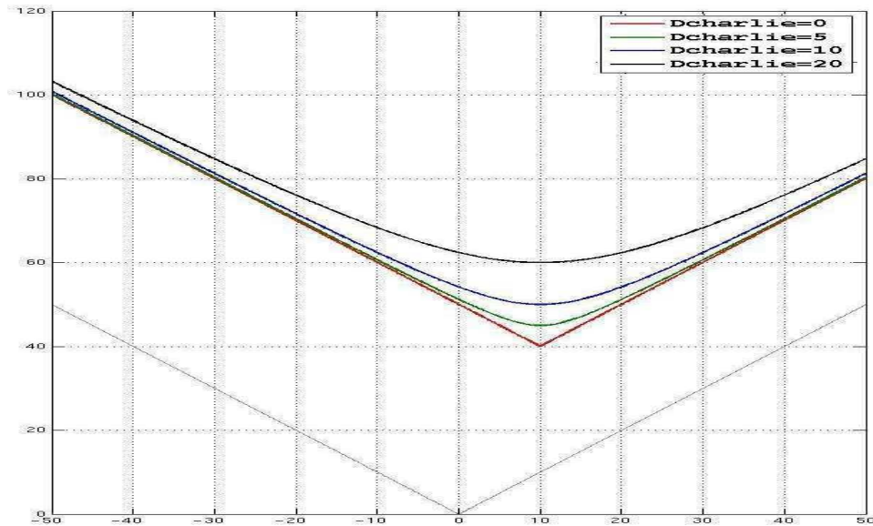
Figure 3-15 : Le diagramme de Charlie pour différentes valeurs de D_{charlie}
