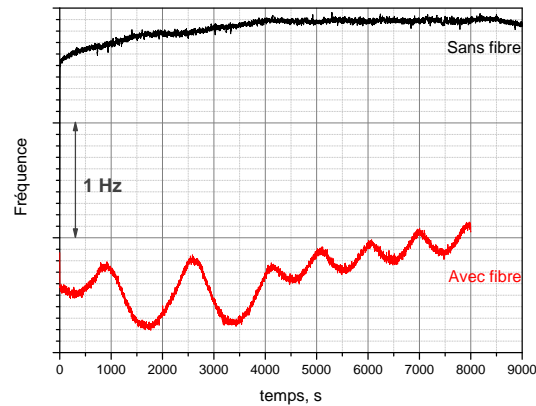
Figure 3.17 – Variations de la fréquence d'horloge avec et sans fibre optique. Les variations périodiques sont largement réduites dans le cas sans fibre optique. Les variations long terme (dérive) correspondent au changement de la température du modulateur acousto-optique. L'écart en fréquence entre les deux courbes correspond au changement de l'intensité laser (sans fibre, l'intensité est augmentée d'un facteur 2).
