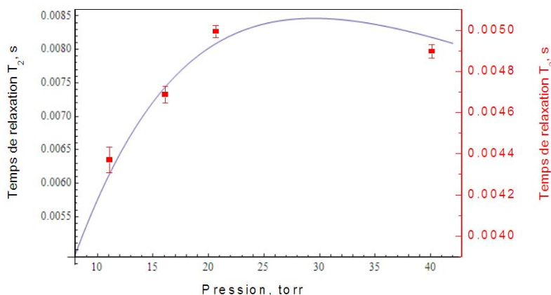
Figure 5.23 – Temps de relaxation de la cohérence T_2 en fonction de la pression de gaz tampon. Points rouges - mesures expérimentales. Conditions expérimentales: cellules de diamètre 20 mm et de longueur 20 mm, température 29°C, diamètre du faisceau 12 mm, intensité 973 \mu\text{W}/\text{cm}^2 , champ magnétique 210 mG, schéma double- \Lambda , méthode Franzen. Courbe bleu - valeurs calculées.
