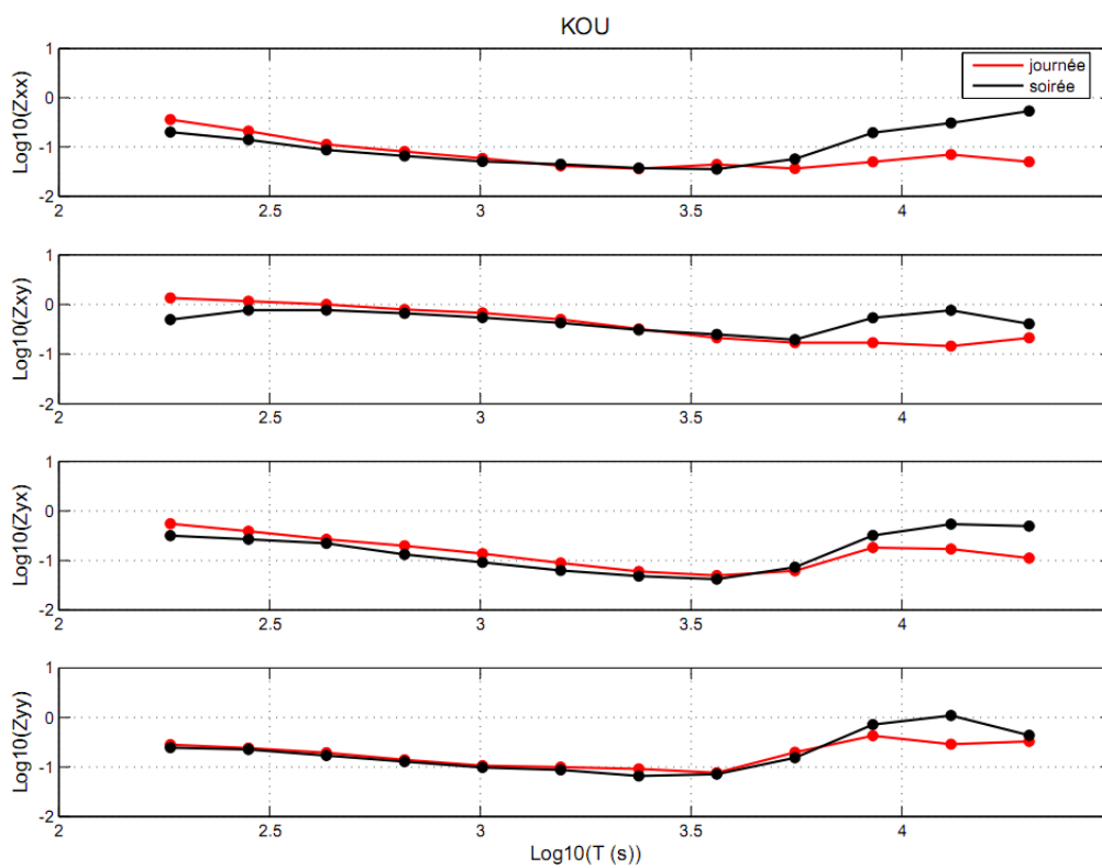
Figure 6.7: Composantes du tenseur MT calculées aux stations de l'AIEE. Les courbes en noir et en rouge sont calculées pour les données enregistrées en soirée et en journée, respectivement.
