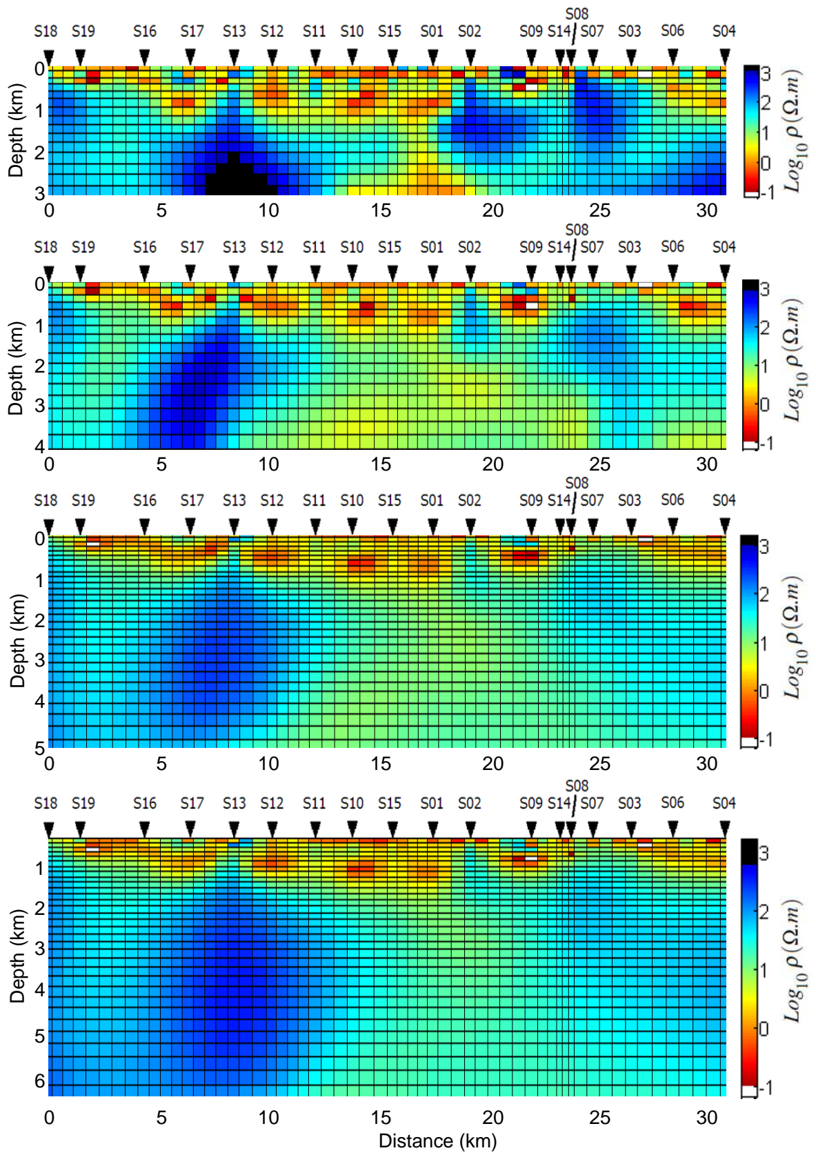
Figure 4.16: La comparaison des résultats des inversions pour un niveau de bruit de 20% des différents modèles correspondent à l'analyse détaillée des 3, 4, 5 et 6 premiers kilomètres.
