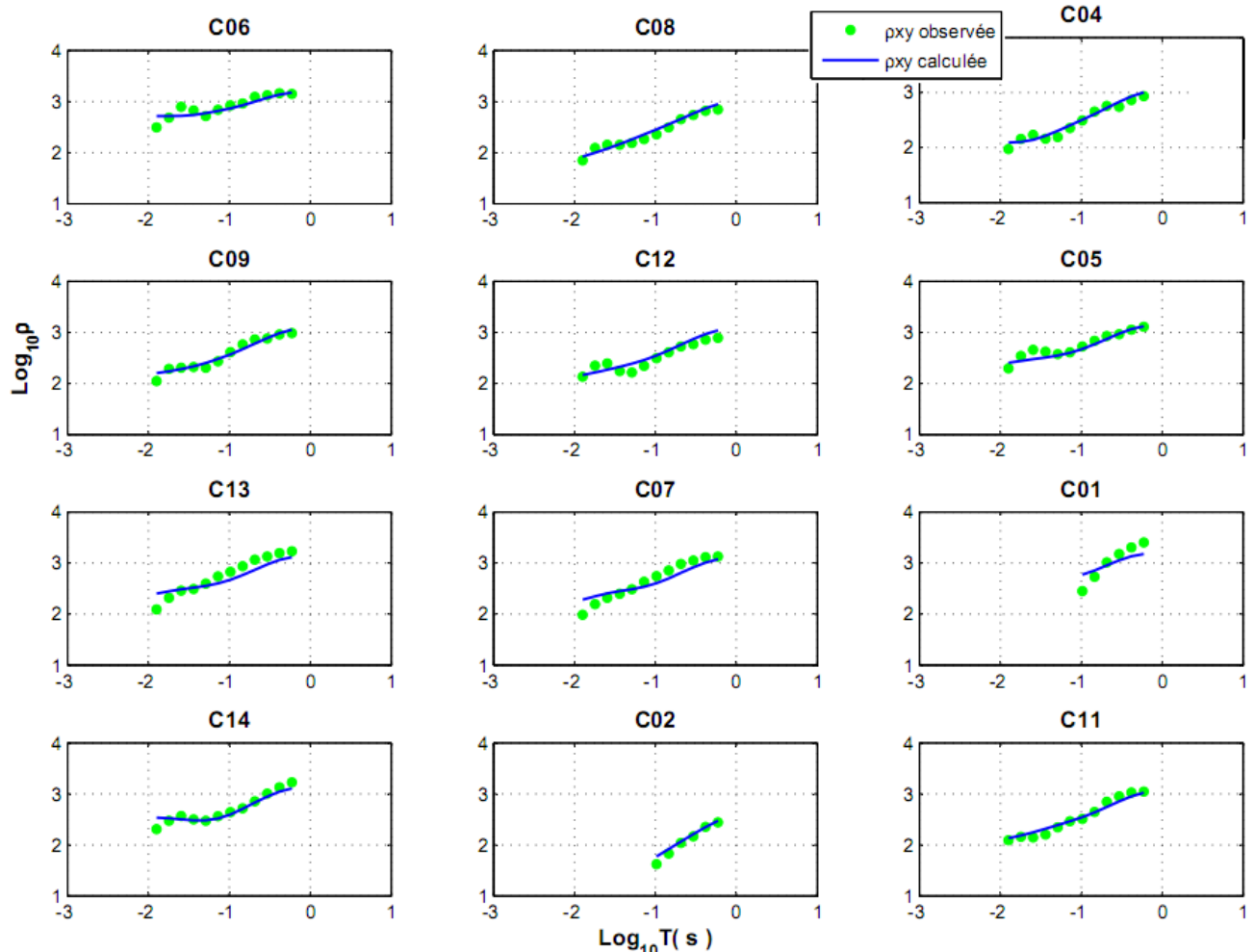
FIGURE 5.20: Les résistivités observées et calculées à partir du modèle obtenu par l'inversion 2-D du mode TE, chaque sous-figure pour chaque station de mesure. Les cercles verts sont les résistivités observées de \rho_{xy} . Les courbes bleues sont les résistivités calculées à partir du modèle obtenu après 6 itérations.
