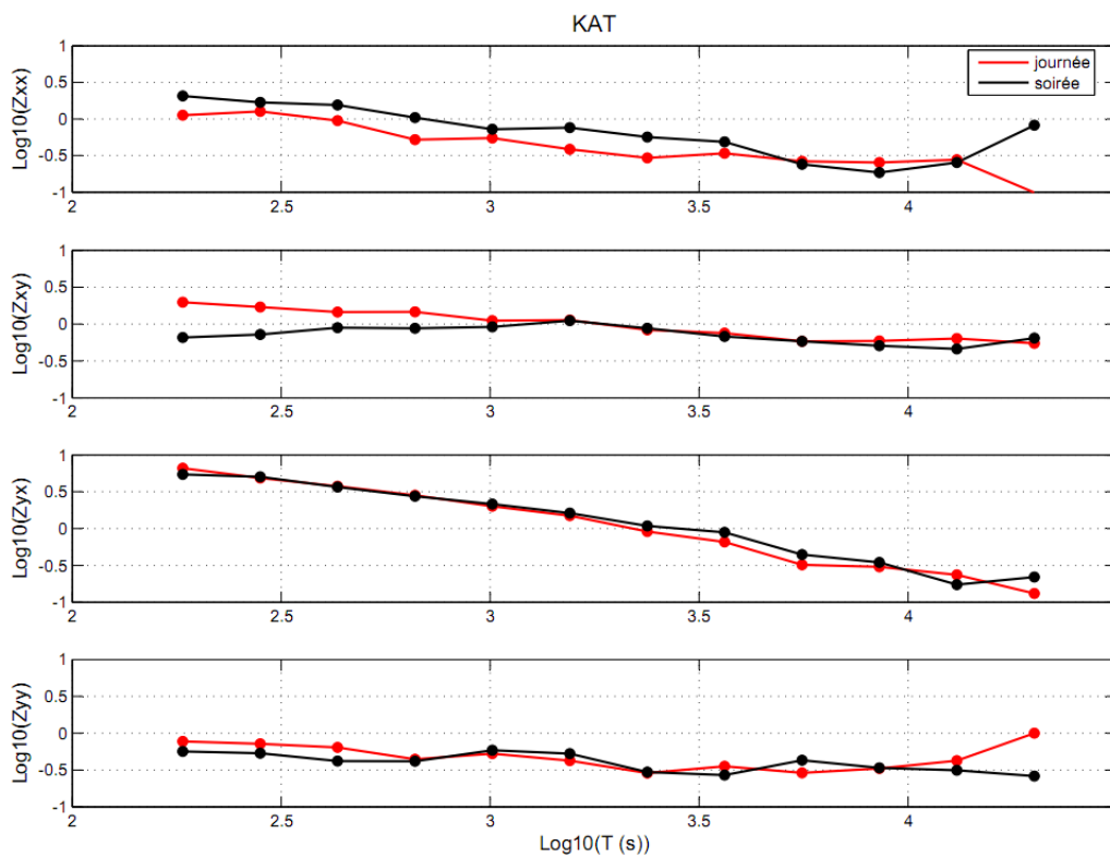
FIGURE 6.9: Composantes du tenseur MT calculées aux stations de l'AIEE. Les courbes en noir et en rouge sont calculées pour les données enregistrées en soirée et en journée, respectivement.
