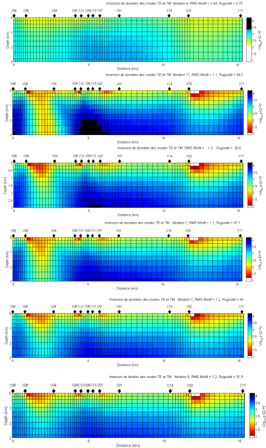
FIGURE 5.18: Pseudo-sections électriques des trois premiers kilomètres obtenues par l'inversion d'Occam 2-D des données des modes TE et TM. De haut en bas : l'inversion a été effectuées avec un substratum à une profondeur de 3 km, 5 km, 8 km, 10 km, 15 km et 20 km.
