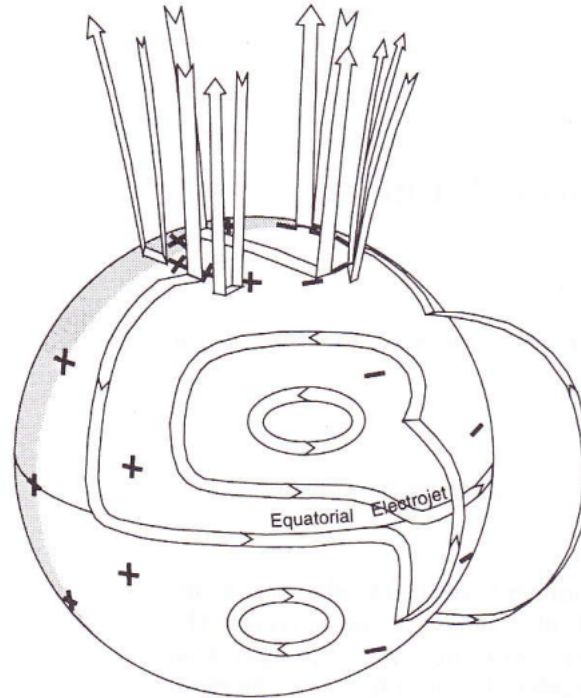
Figure 2.15: Schéma des courants électriques ionosphériques mondiale (rubans avec des flèches) et des potentiels électriques (+ et -), vu du côté jour de la Terre (figure 1 de Richmond et Thayer, 2000).
