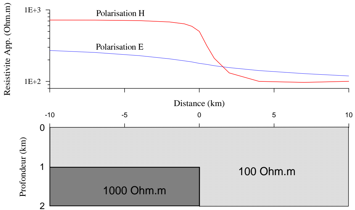
Figure 3.6: (en bas) Modèle 2-D d'un pas de résistivité de 1000 \Omega.m dans un milieu dont la résistivité est de 100 \Omega.m . (en haut) Résistivités apparentes à la surface de la structure, calculées pour les polarisations H et E à la période de 10 s.
