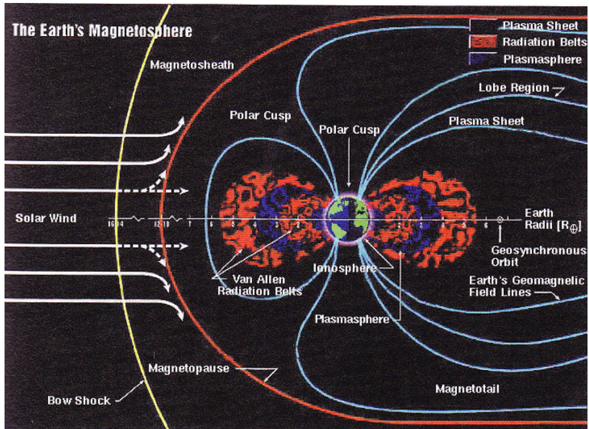
FIGURE 2.7: Illustration schématisique de la magnétosphère, avec l'insistance sur les ceinture de radiation de Van Allen et sur la plasmasphère (tirée de Bothmer et Daglis, 2007).
