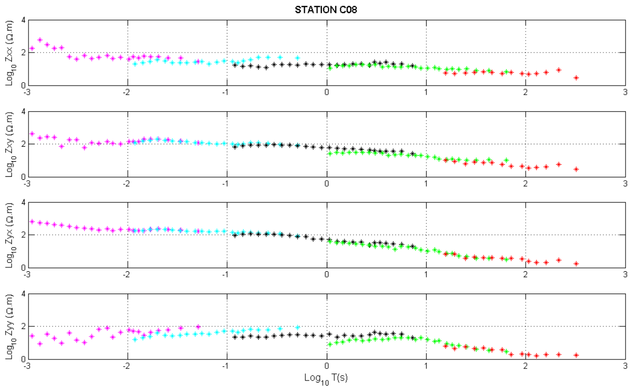
Figure 5.3: Valeurs des éléments du tenseur d'impédance calculés à partir des données enregistrées pour les gammes de période G1 (en magenta), G2 (en cyan), G3 (en noir), G5 (en vert) et G7 (en rouge)
