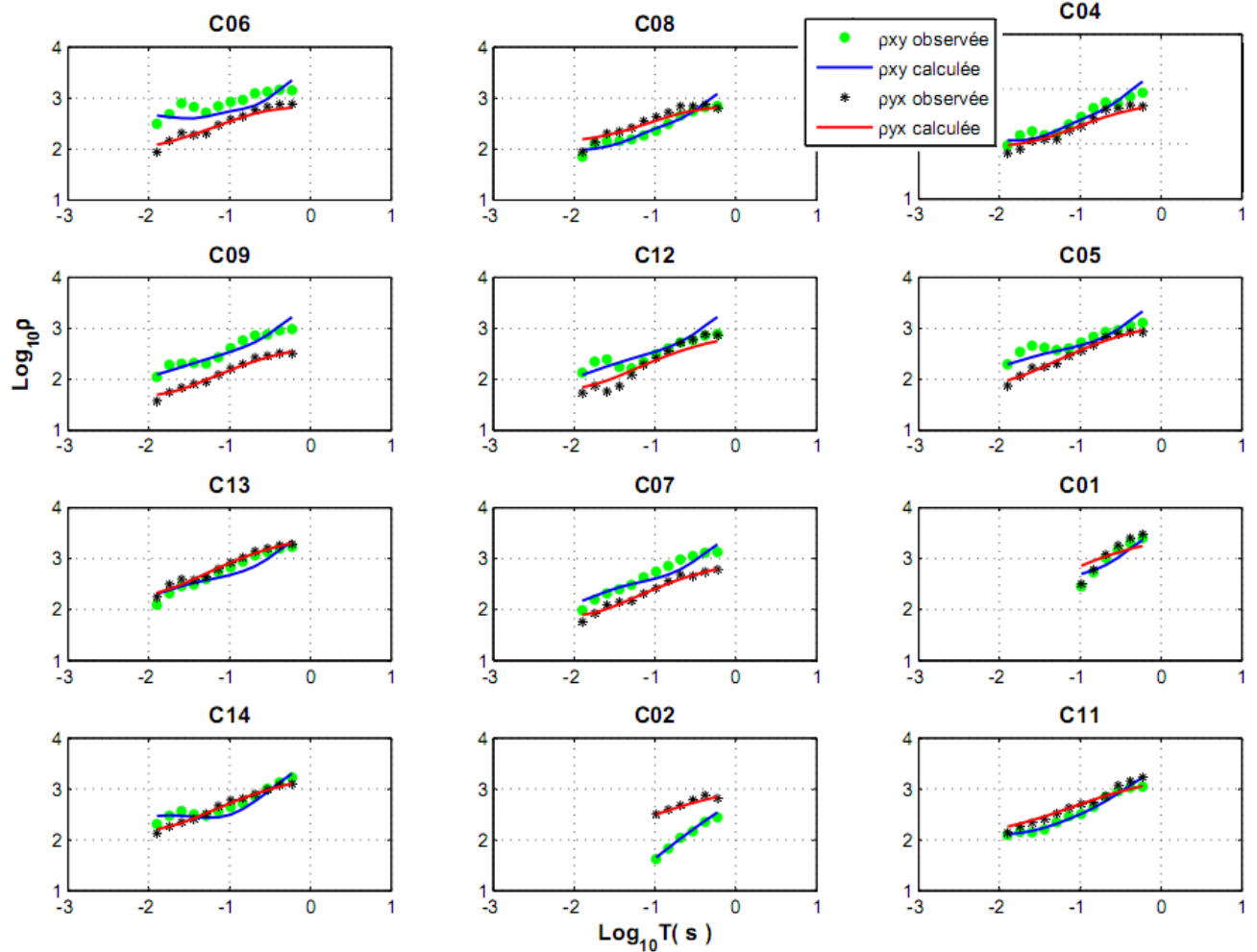
FIGURE 5.22: Résistivités apparentes observées et calculées à partir du modèle obtenu par l'inversion 2-D des modes TE et TM. Sur chaque sous-figure, les cercles verts et les astérisques noirs correspondent aux résistivités apparentes observées \rho_{xy} et \rho_{yx} , respectivement, et les courbes bleue et rouge correspondent respectivement aux résistivités apparentes \rho_{xy} et \rho_{yx} calculées à partir du modèle obtenu après 7 itérations.
