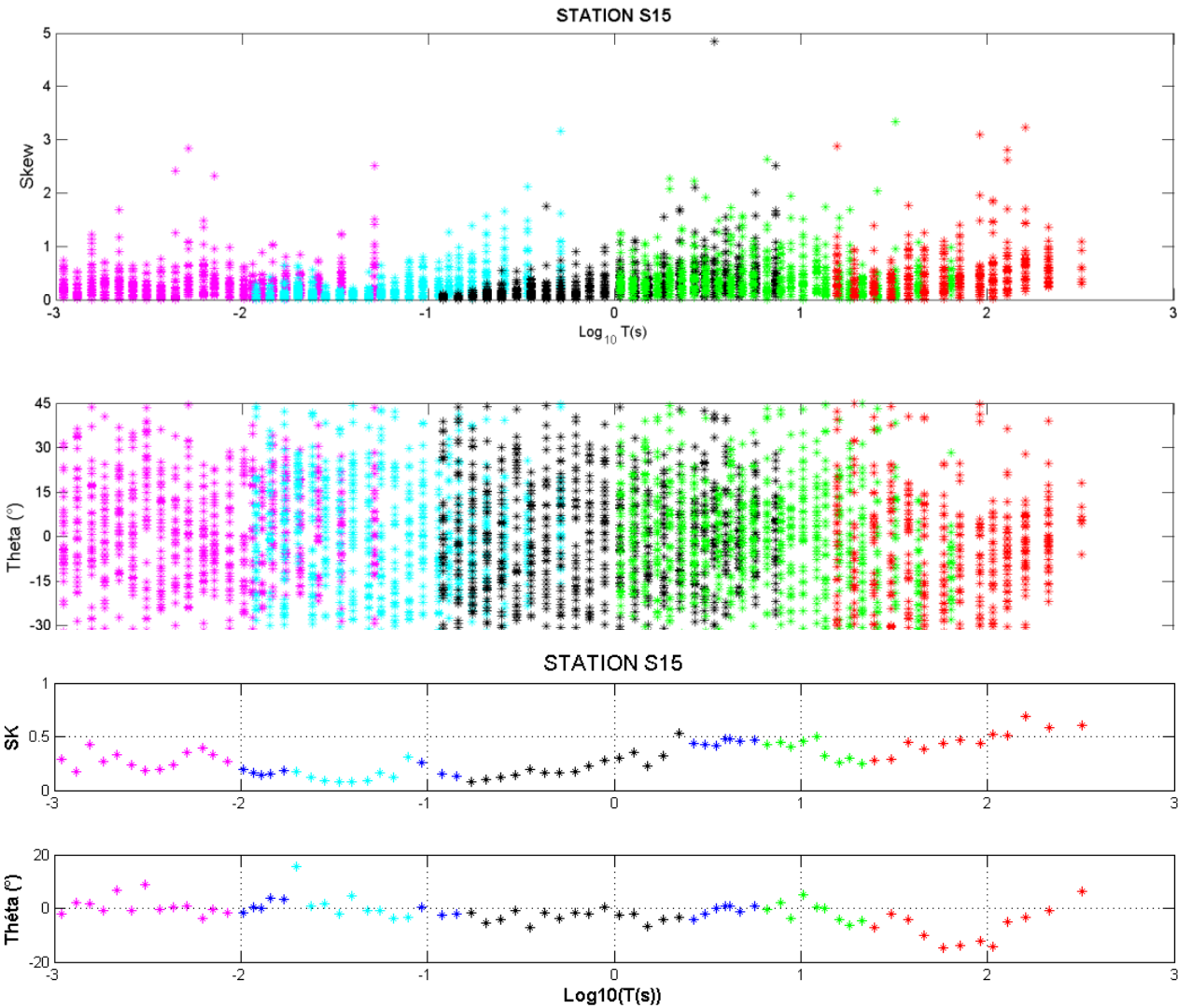
FIGURE 4.14: Courbes des valeurs de Skew (en haut) et de Théta (en bas) après avoir traité des chevauchements entre les gammes.
