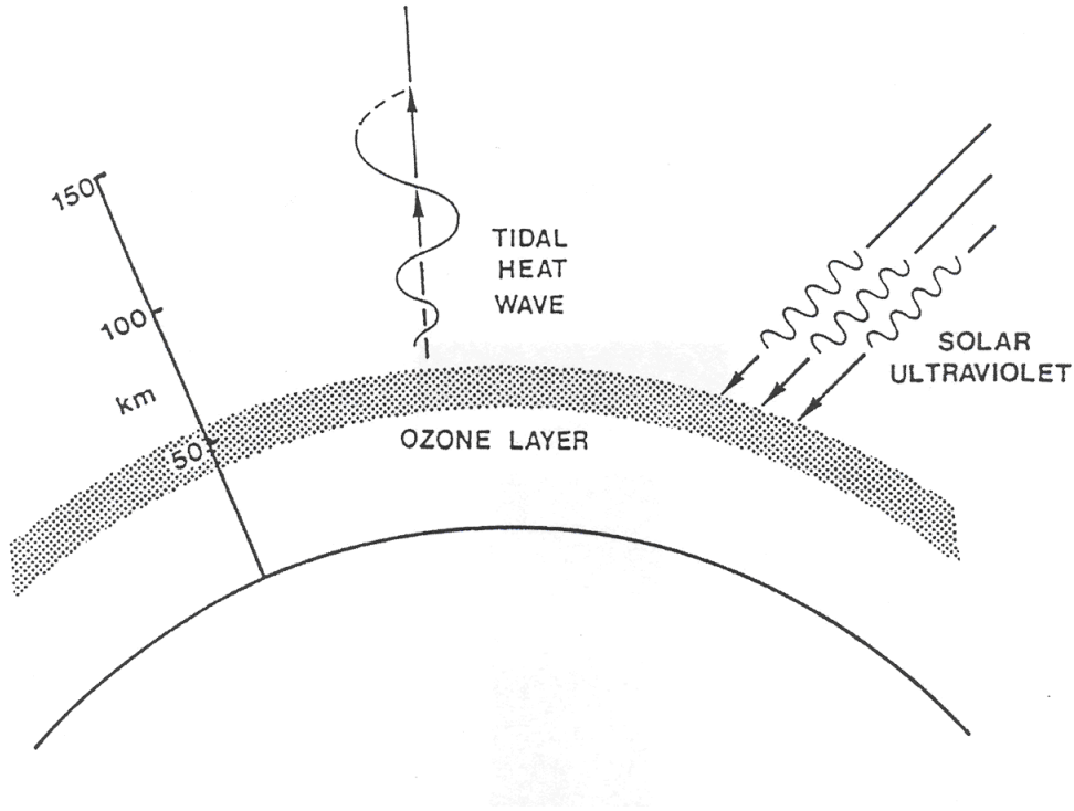
Figure 2.13: Sources principales des courants électriques dans l'ionosphère : les marées atmosphériques (Evans, 1977)
