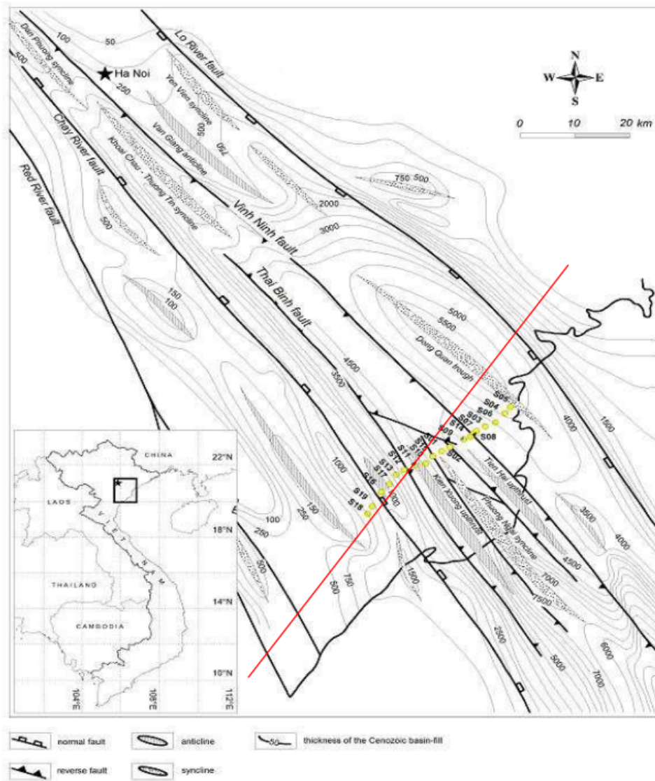
Figure 4.1: Carte structurale du bassin de la Rivière Rouge (adapté de la figure 3 de Phach, 1996). Les stations MT sont indiquées par des points jaunes et par leur nom. La ligne rouge indique la localisation de la coupe géologique présentée figure 4.3.
