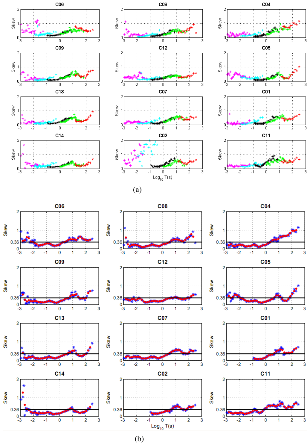
Figure 5.11: (a) Valeurs du coefficient de disymétrie ( Skew ) aux périodes calculées des gammes de période de toutes les stations du profil.
