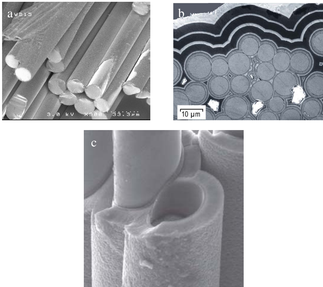
Figure 1.6 a) Fibres de SiC [Cabrero09], b) coupe transverse de SiC fibré /SiC [CEA08] et c) fracture de SiC fibré /SiC avec une interphase en carbone [CEA07]
