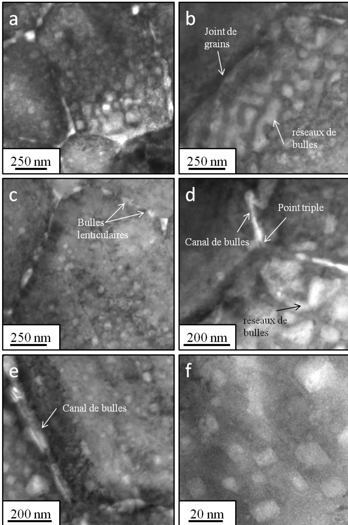
Figure 3.35 Micrographies MET d'un échantillon implanté à 10^{17} \text{Xe.cm}^{-2} et recuit 1 heure à 1800^\circ\text{C} . Les clichés de a à e ont été réalisés dans la zone 2 (milieu de la lame), le cliché f dans la zone 1 (bord de lame).
