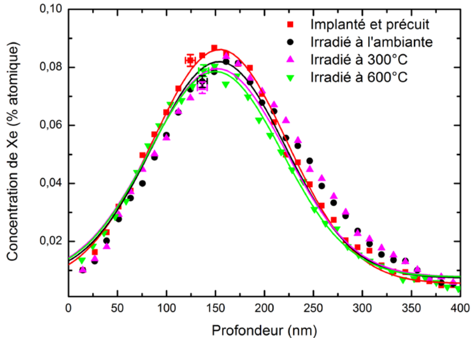
Figure 4.5 Profils de concentration en ^{136}\text{Xe} d'un échantillon implanté (800 keV, 10^{15} \text{Xe.cm}^{-2} ) et précuit, irradiés avec des ions W (2,85 MeV, 5 \times 10^{15} \text{W.cm}^{-2} ) à température ambiante, 300 et 600°C
