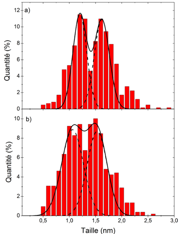
Figure 3.24 Distributions de la taille des bulles de deux échantillons implantés à 10^{16} Xe.cm -2 et recuits (a) 1 et (b) 16 heures à 1800°C
