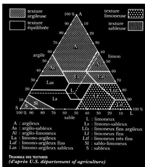
Figure 2 : Triangle de texture des sols
